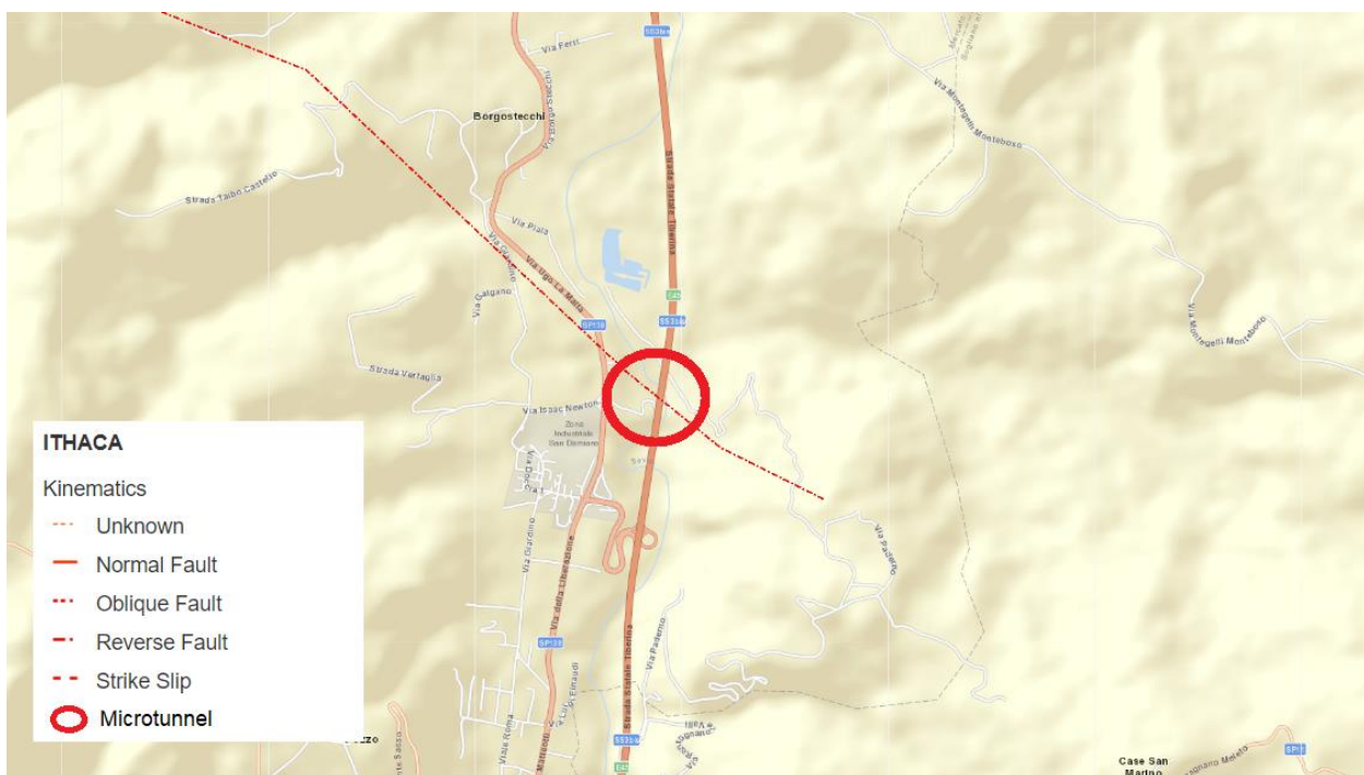
Figura 6-I: Stralcio database ITHACA (ISPRA) relativamente all'area di interesse. Accessibile al link https://sgi.isprambiente.it/ithaca/viewer/index.html
