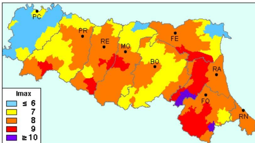
Figura 6-B: Massime intensità macrosismiche in scala MCS osservate nella Regione Emilia-Romagna (GNDT, ING, SSN).
