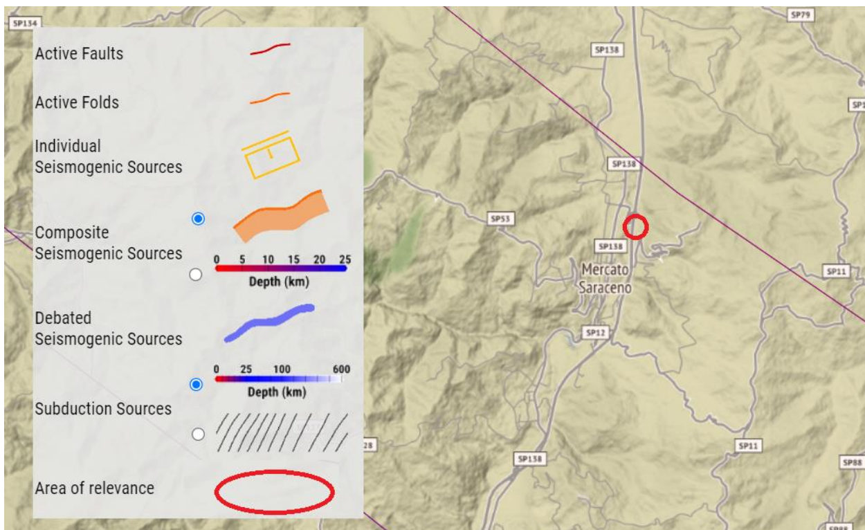
Figura 6-H: Stralcio database DISS versione 3.3.0 (2021, INGV) relativamente all'area di interesse.
