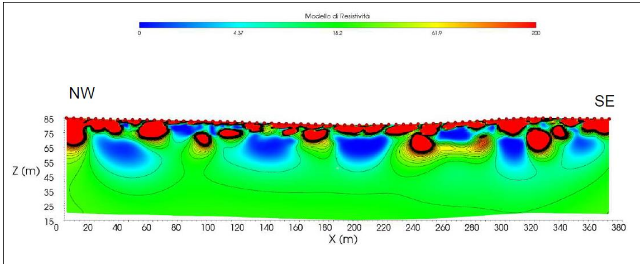
Figura 7-B: Tomografia elettrica ERT39_SM_L
