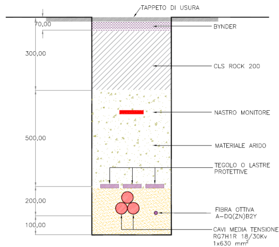
Figura 21 - sezione tipica di posa della linea in cavo su strada
