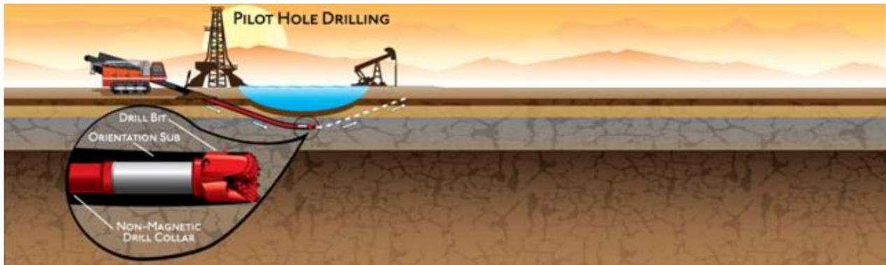
Figura 17 - Perforazione pilota -TOC
