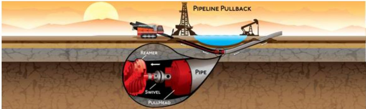
Figura 19 - tiro e posa -TOC
