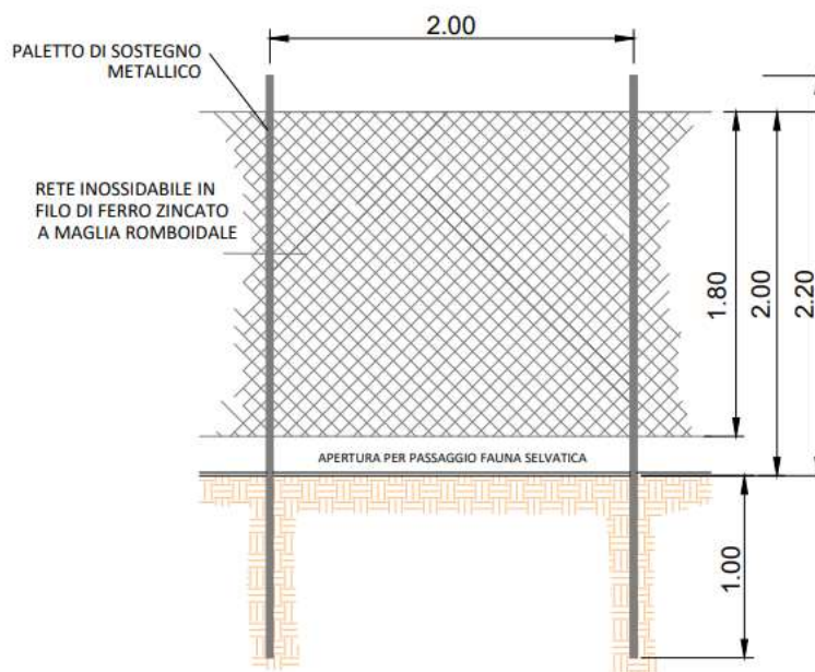
Figura 8 - Composizione recinzione
