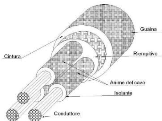
Figura 6 - Composizione Cavo elettrico con guaina
