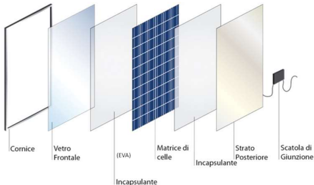
Figura 3 – Composizione dei moduli fotovoltaici
