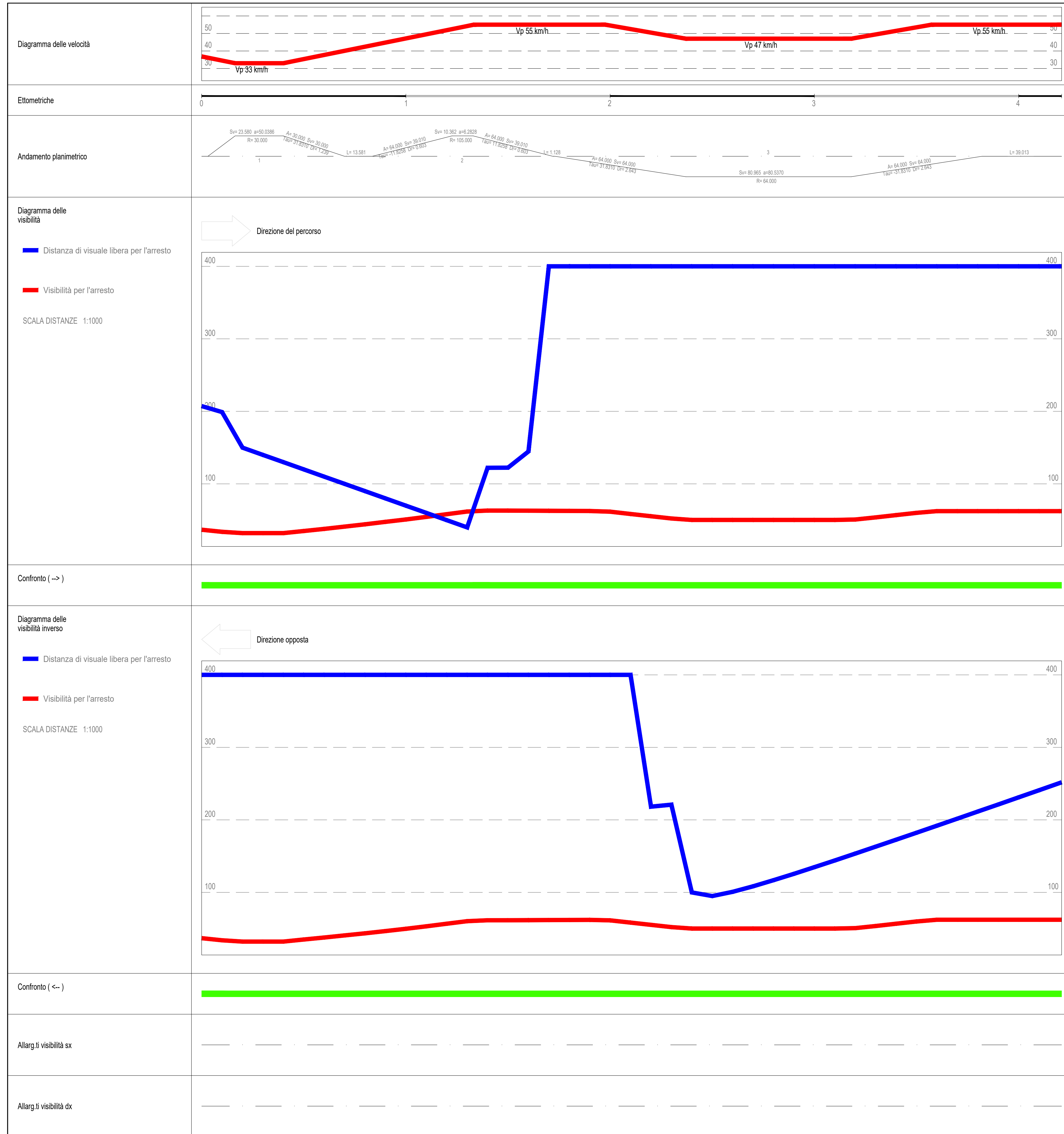
DIAGRAMMA DELLE VISIBILITA' E DELLE VELOCITA' - INTERVENTO 31 SCALA 1:1000
