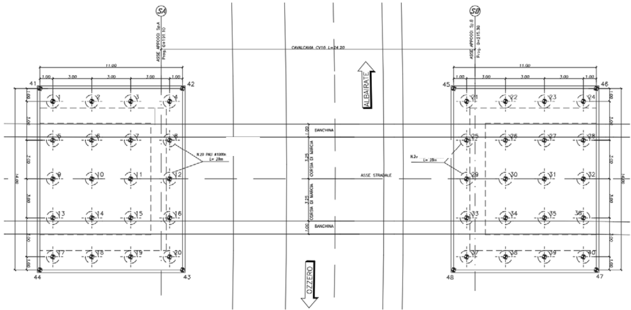
Figura 2: Pianta fondazioni
