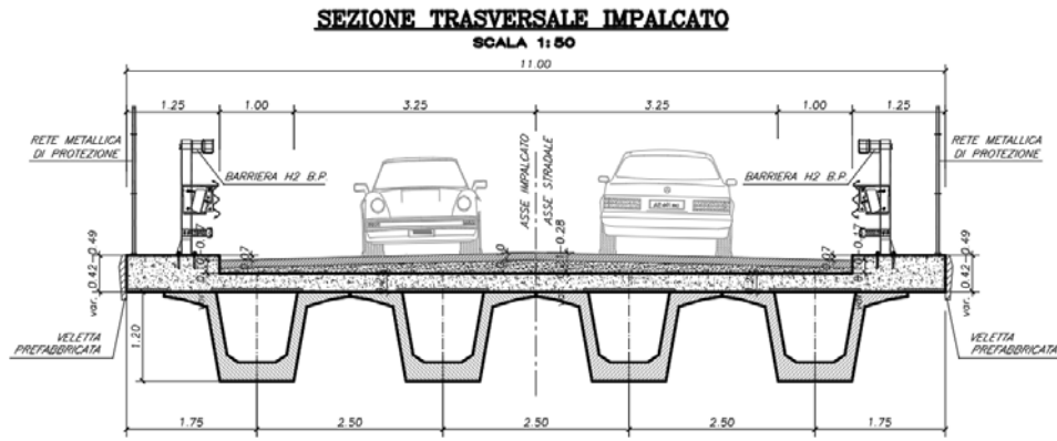
Figura 4: Sezione trasversale
