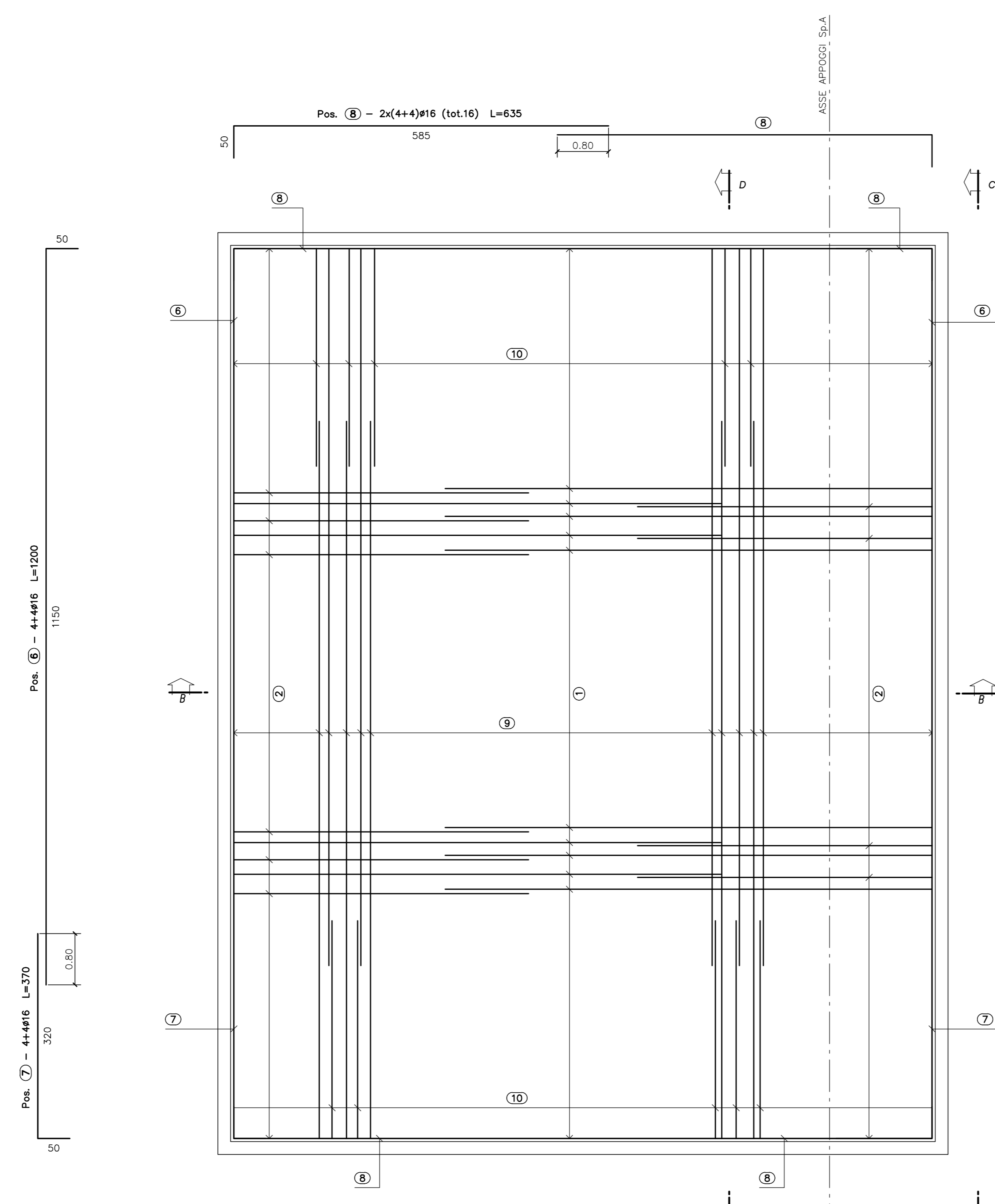
PIANTA FONDAZIONI SUPERIORE SCALA 1:50
