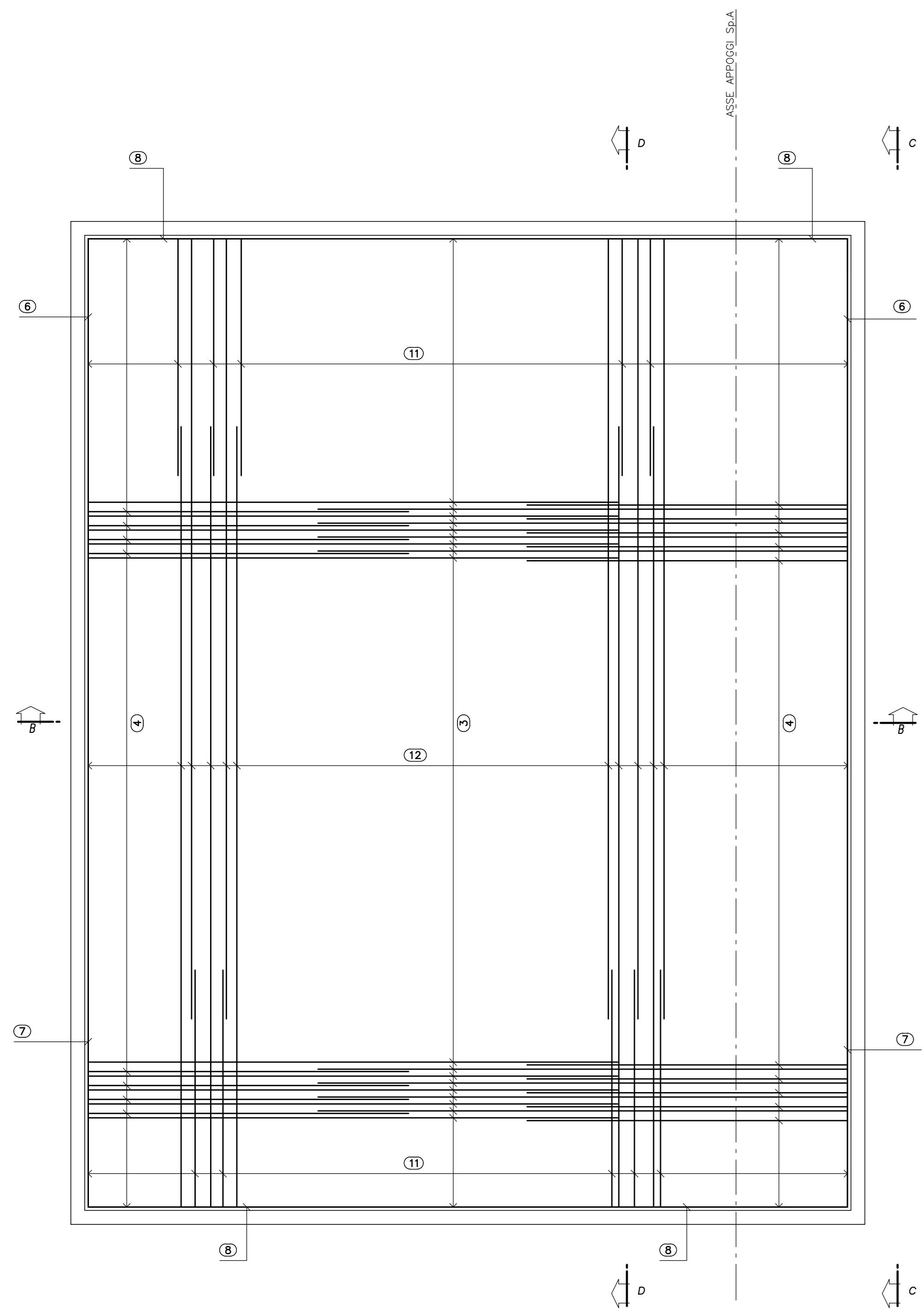
PIANTA FONDAZIONI INFERIORE SCALA 1:50
