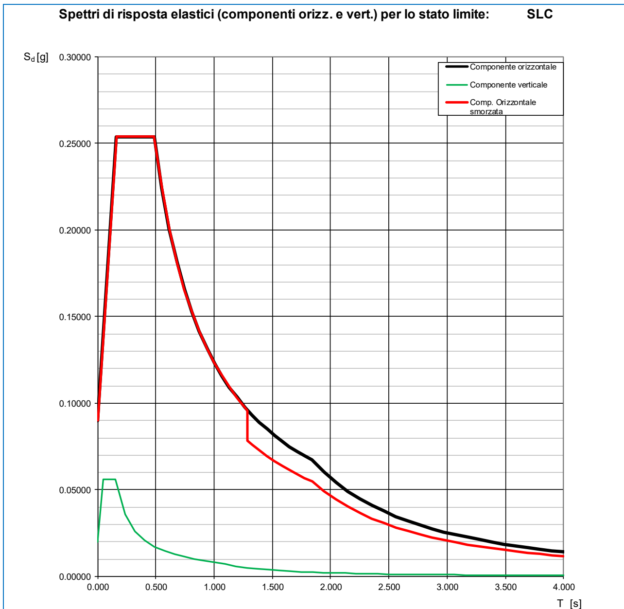
Spettri di risposta elastici e smorzati SLC
