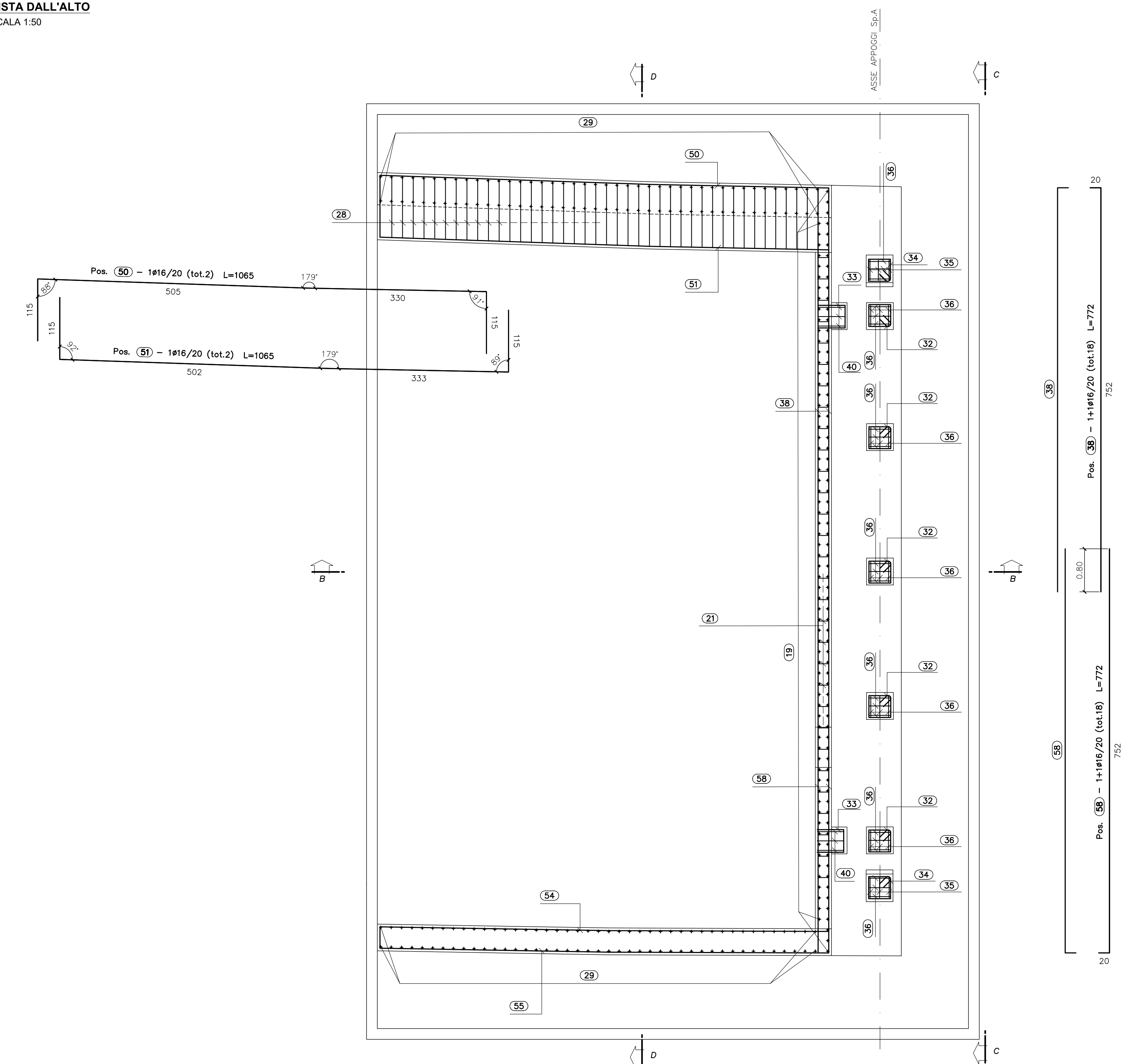
VISTA DALL'ALTO SCALA 1:50
