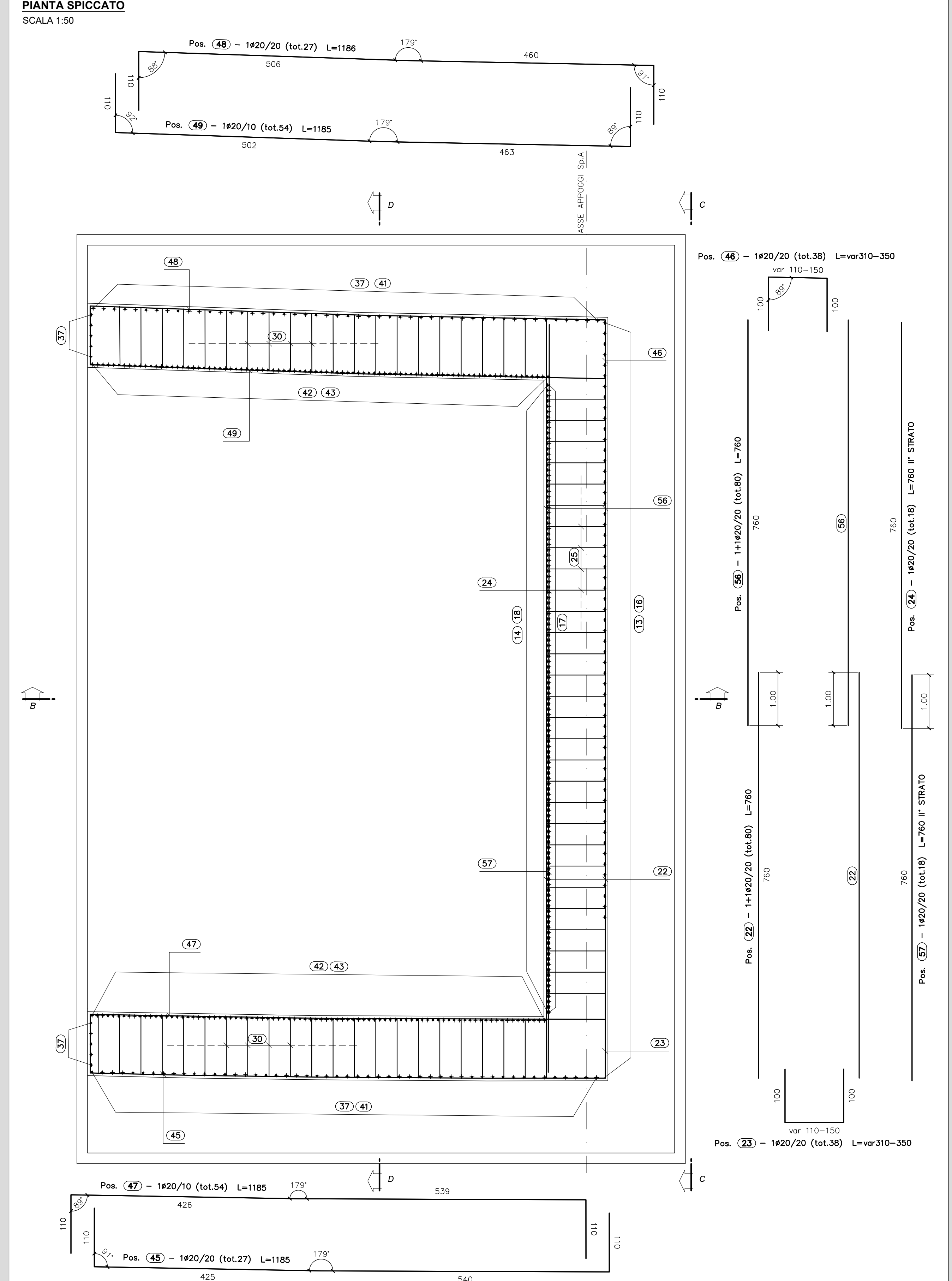
PIANTA SPICCATO SCALA 1:50
