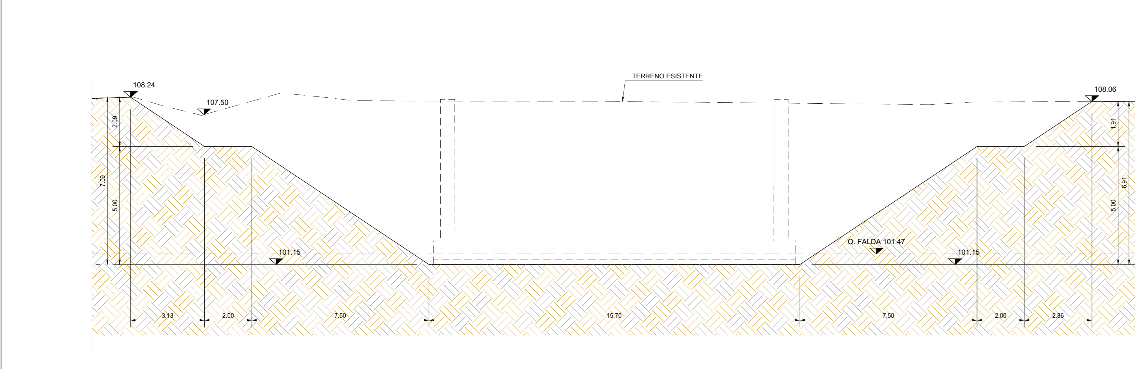
SEZIONE G-G SCALA 1:100
