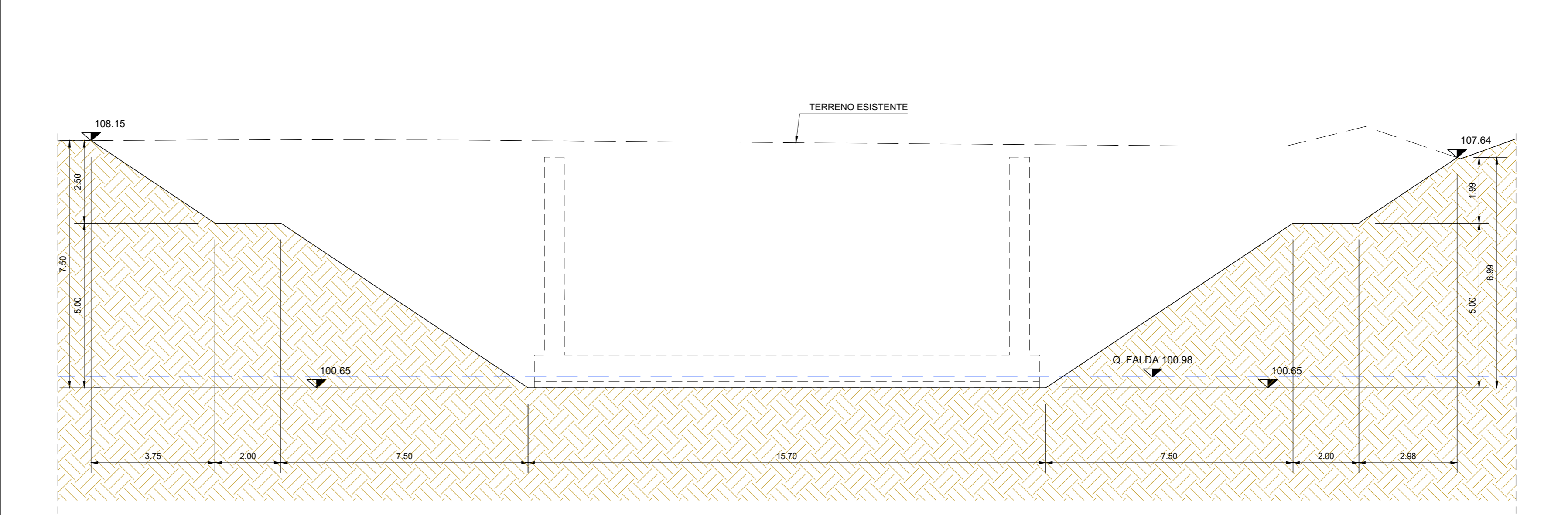
SEZIONE F-F SCALA 1:100
