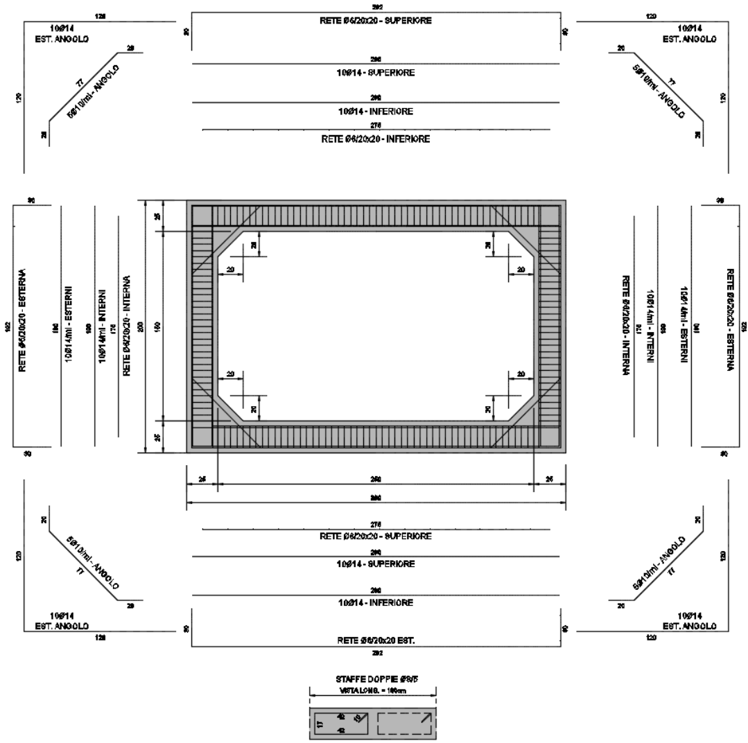
SEZIONE TRASVERSALE DEL MANUFATTO SCATOLARE - ARMATURA
