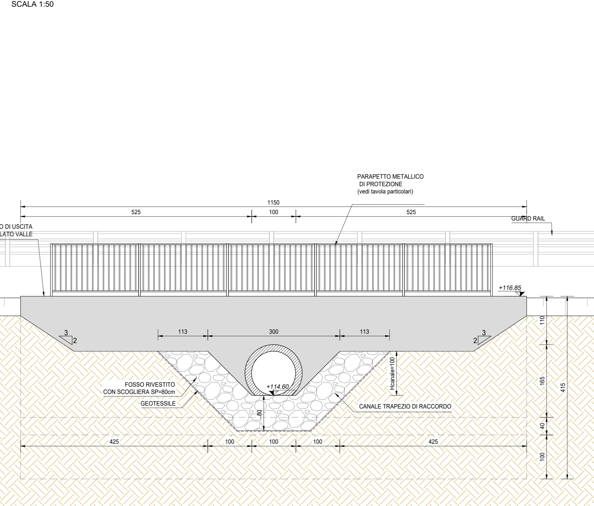
VISTA PROSPETTICA MURO DI SBOCO (SEZIONE D-D) SCALA 1:50
