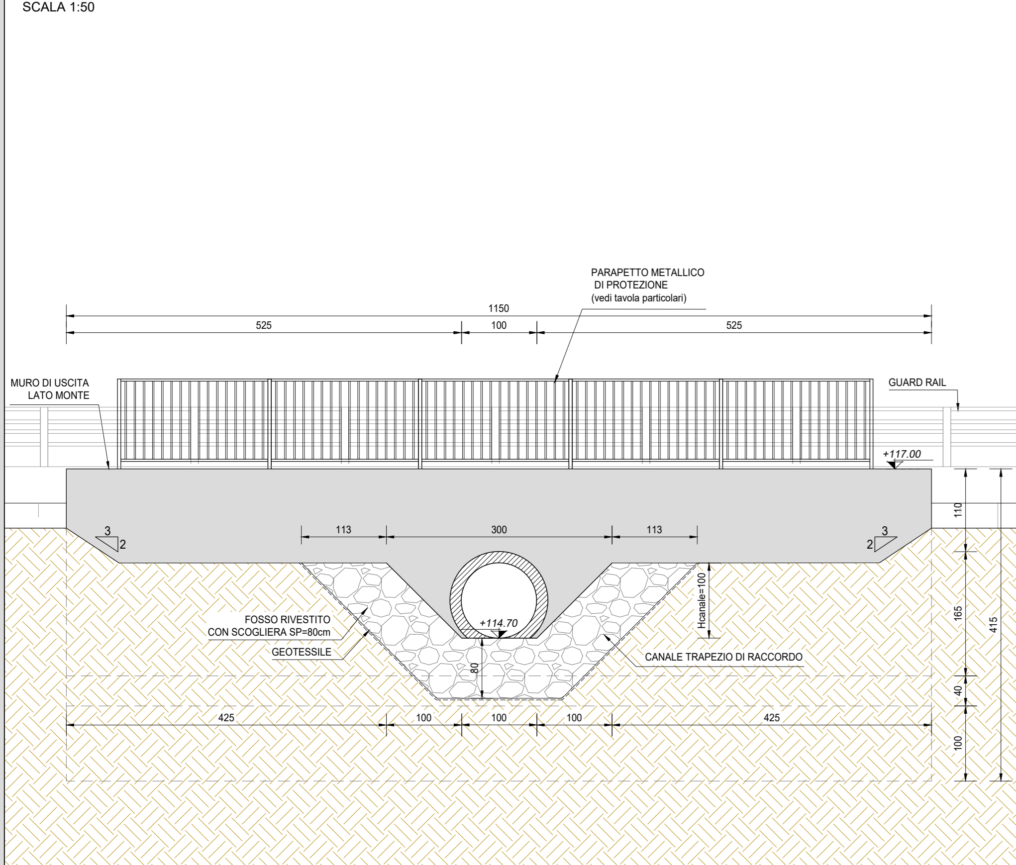
VISTA PROSPETTICA MURO DI SBOCO (SEZIONE B-B) SCALA 1:50
