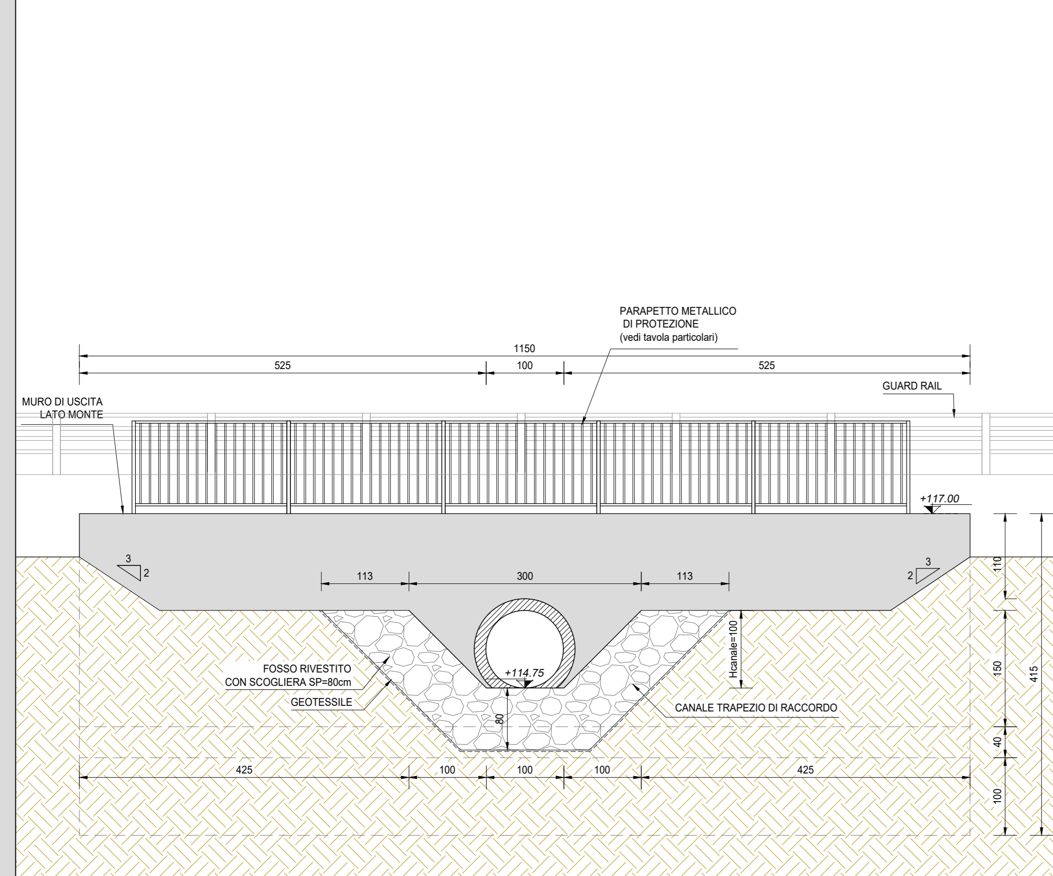
VISTA PROSPETTICA MURO DI SBocco (SEZIONE B-B) SCALA 1:50
