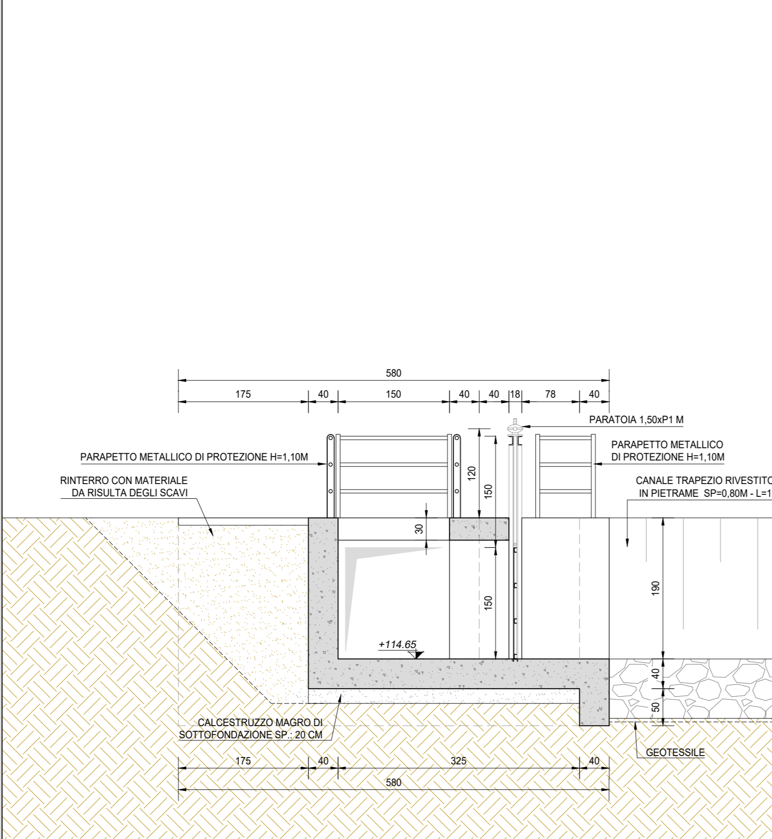
VISTA PROSPETTICA MURO DI SBocco (SEZIONE D-D) SCALA 1:50
