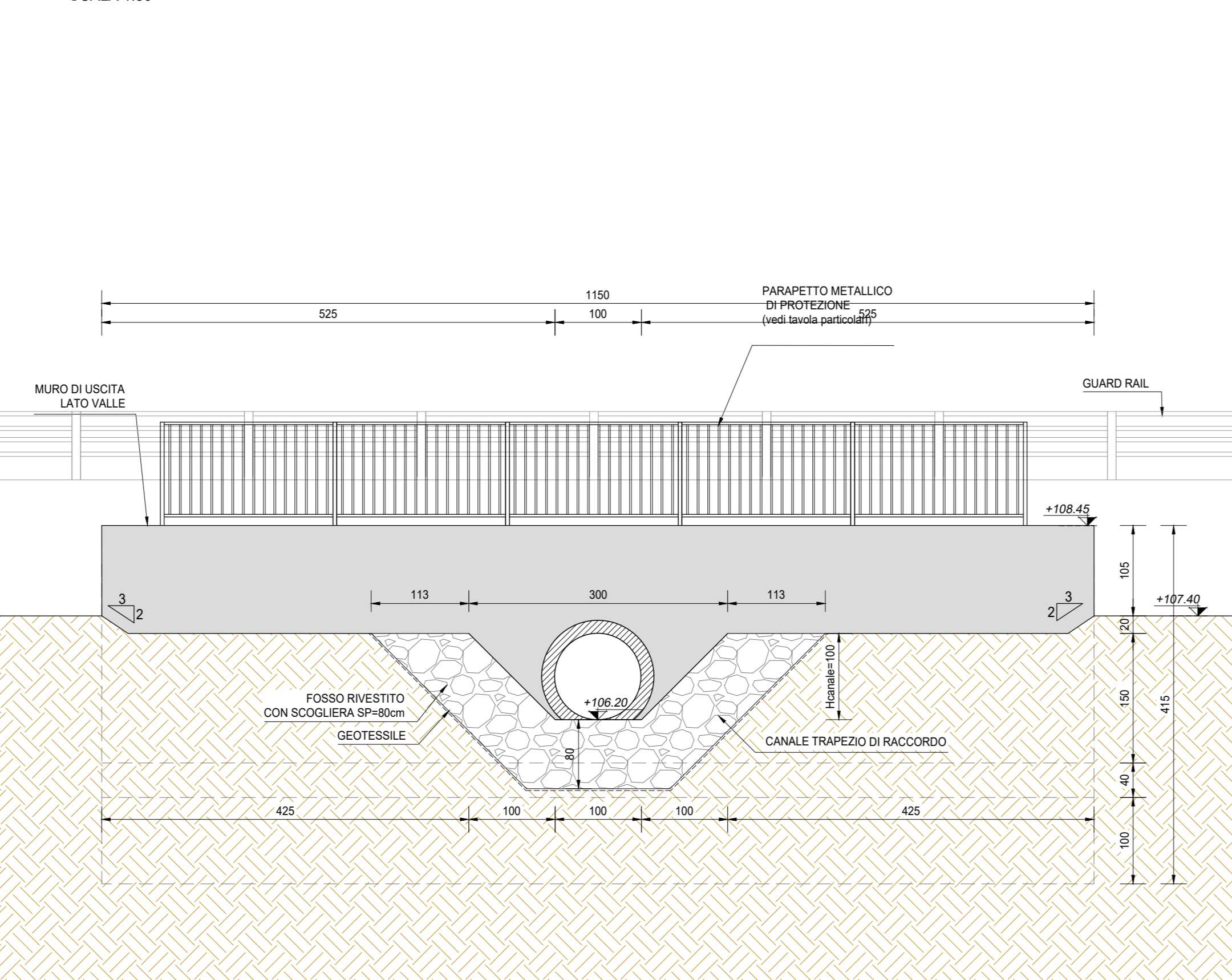
VISTA PROSPETTICA MURO DI SBOTTO (SEZIONE D-D) SCALA 1:50
