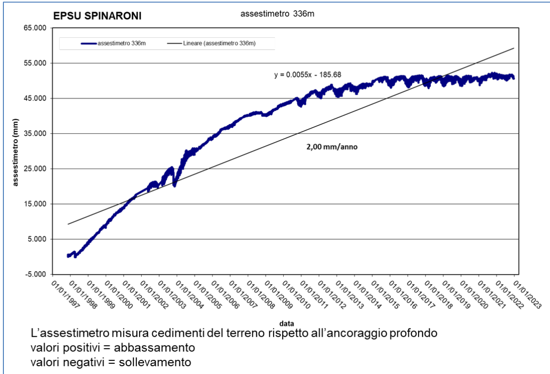
Figura 7B - Serie storica delle misure assestimetriche nella stazione EPSU di Spinaroni
