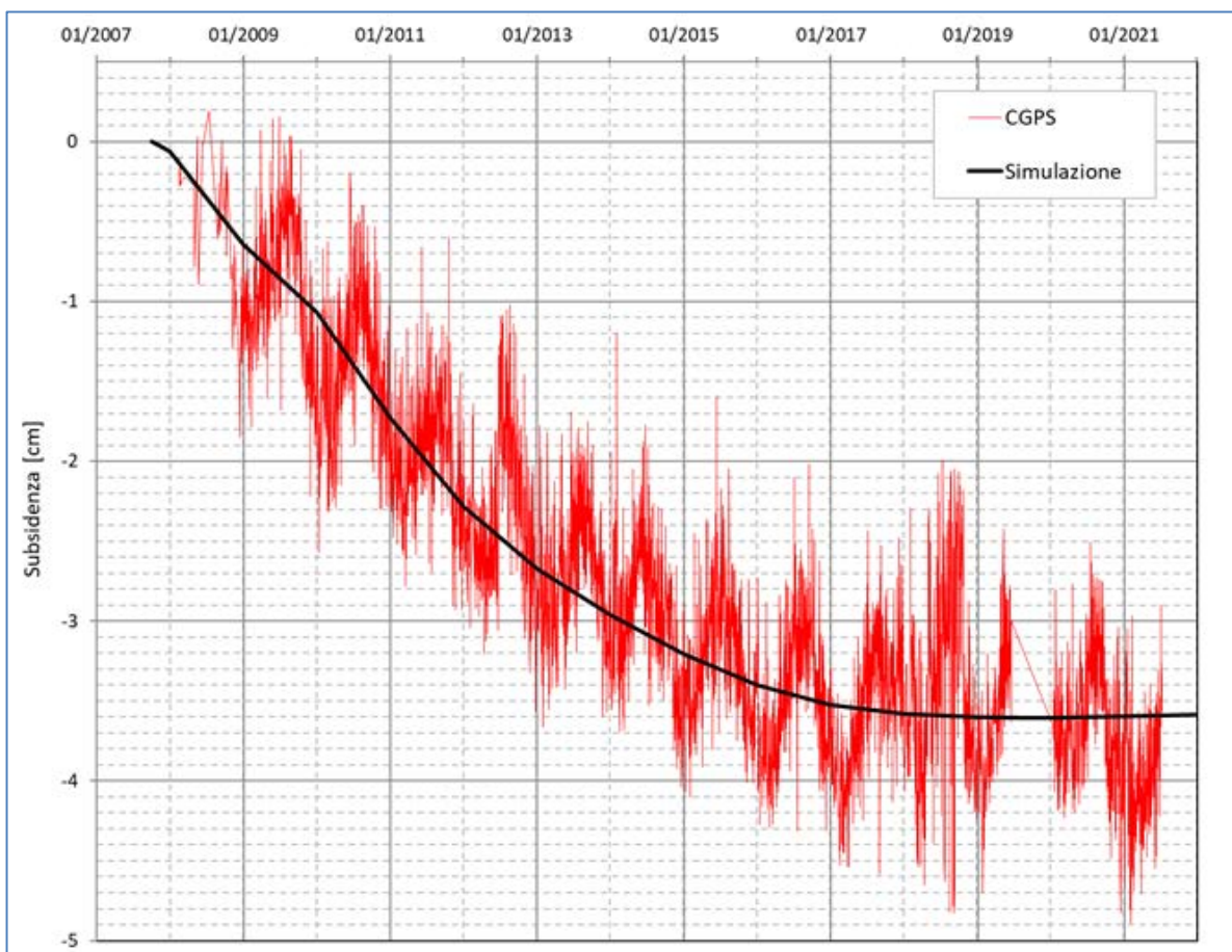
Figura 5 - Campo di TLA: confronto tra spostamento simulato da modello (linea rossa) e spostamento misurato (linea nera), in corrispondenza della stazione CGPS di Tea
