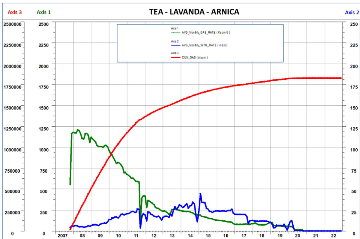
Figura 3 - Campo di TLA: produzione storica
