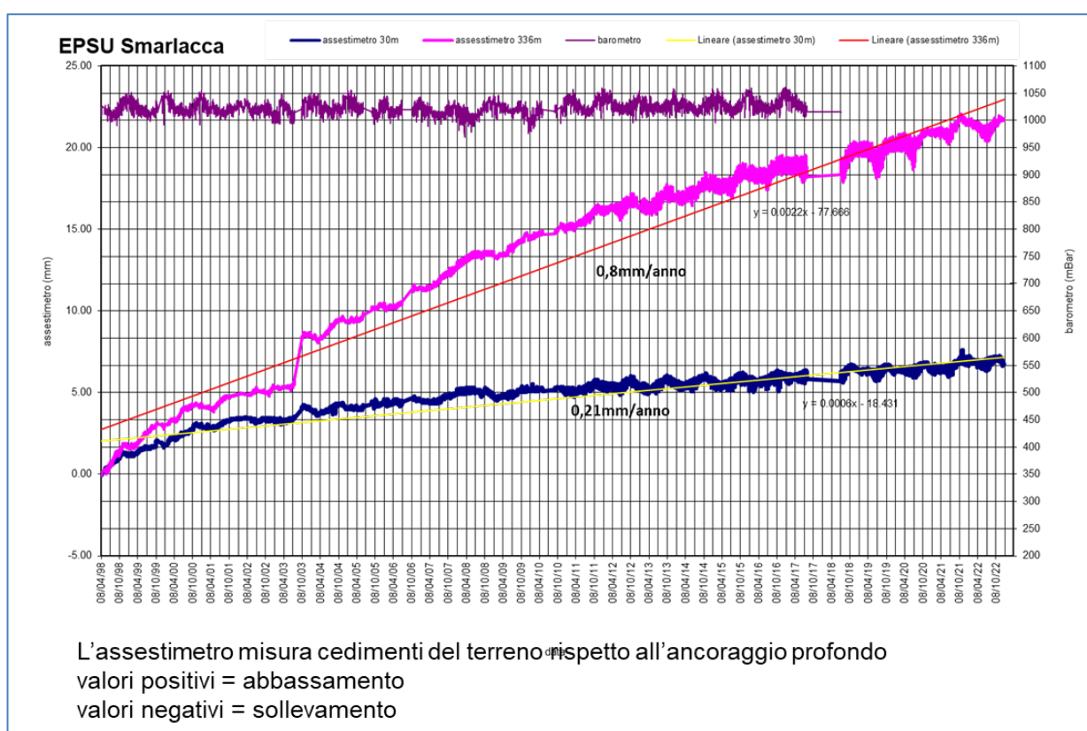
Figura 4B - Serie storica delle misure assestimentriche e barometriche nella stazione EPSU di Smarlacca
