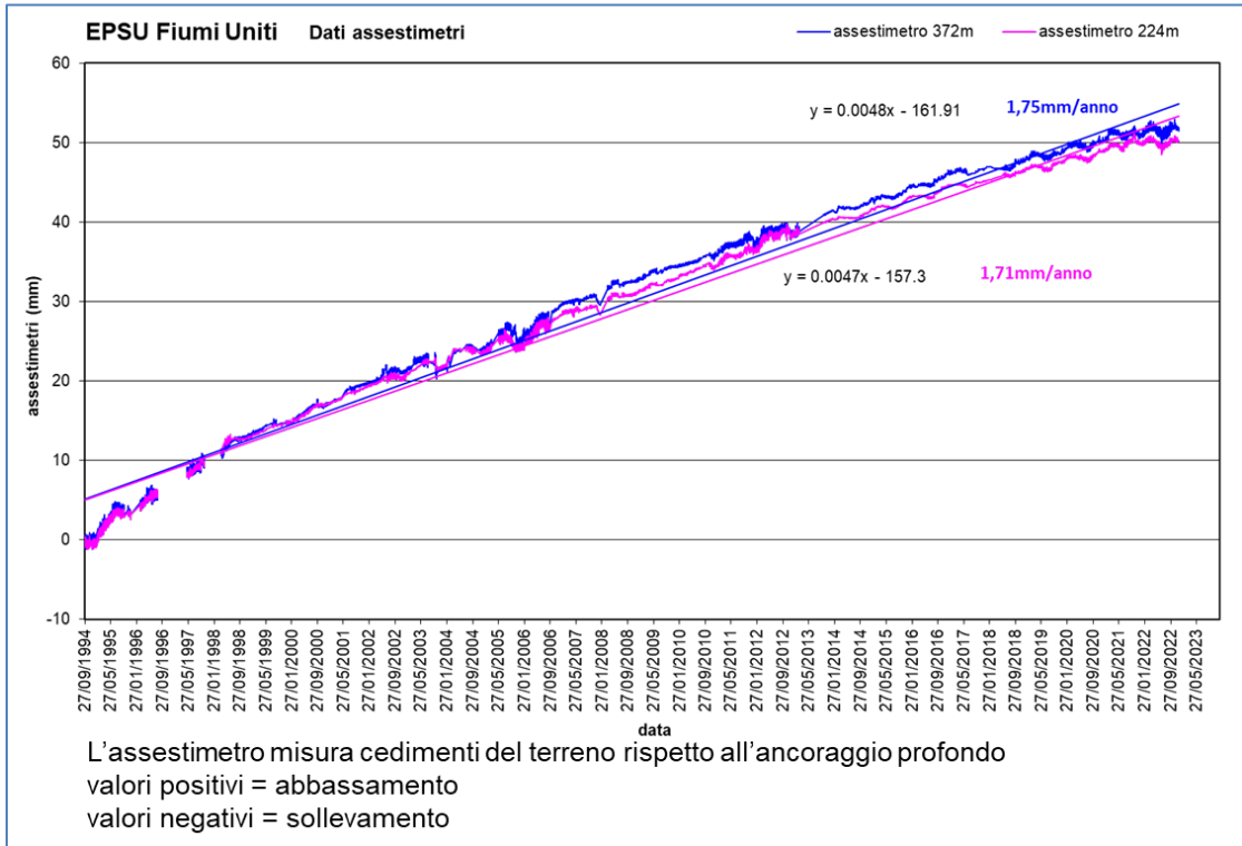
Figura 13B - Curva di compattazione degli assestimetri della stazione EPSU di Fiumi Uniti
