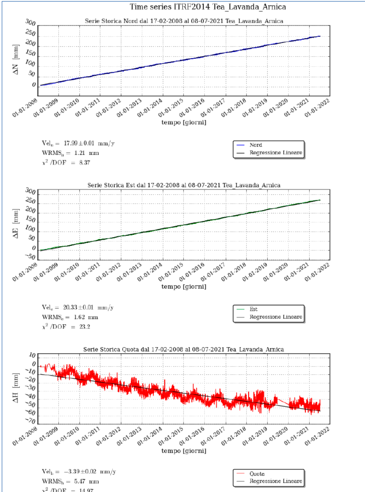
Figura 9 - Campo di TLA: serie storiche di misure CGPS
