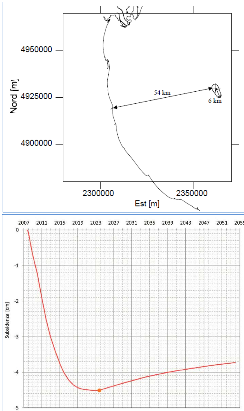
Figura 8 - Campo di TLA: curve di iso-subsidenza (in alto) a fine simulazione (2054) ed evoluzione nel tempo della subsidenza massima (in basso). Il cerchio arancione indica l'abbassamento atteso al termine della produzione (settembre 2023).
