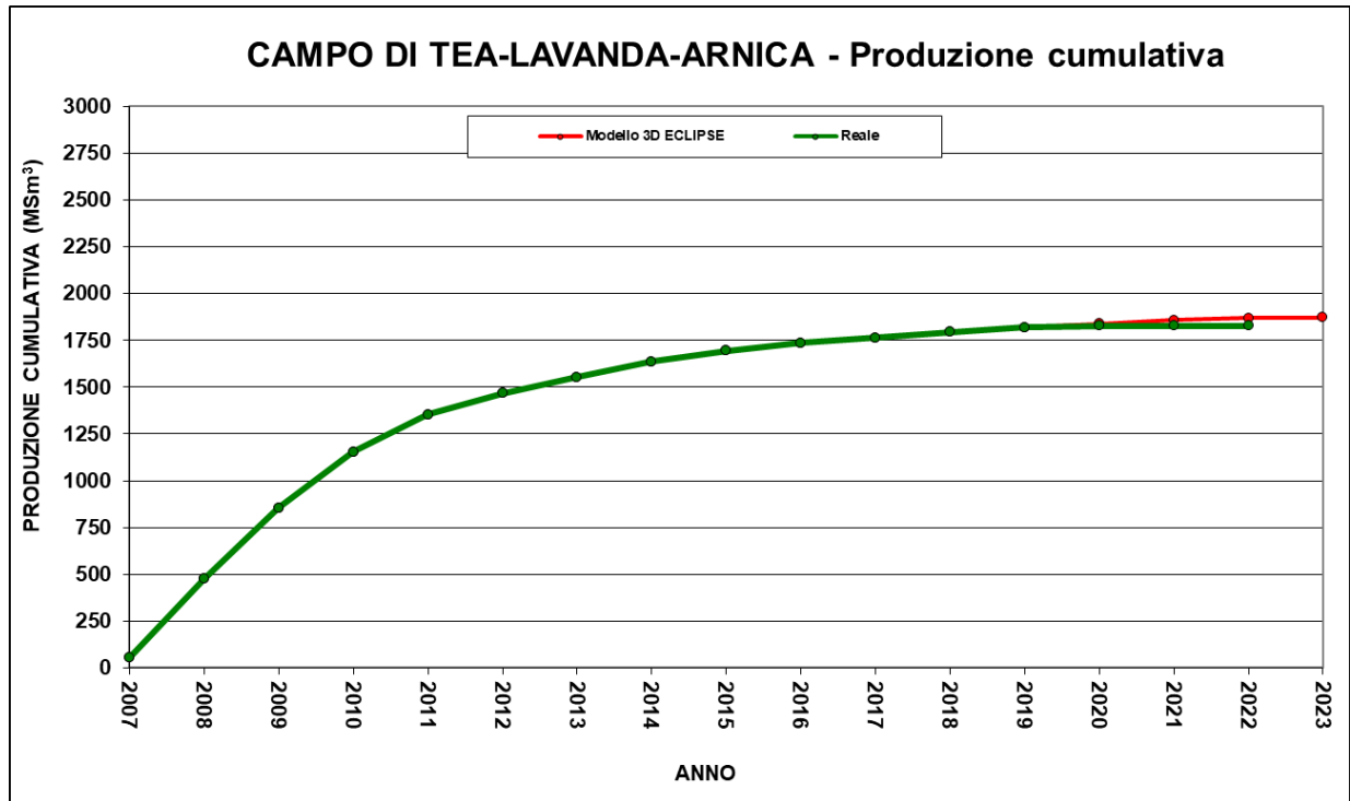
Figura 5 - Campo di TLA: grafico di produzione reale e da modello Eclipse dic.2019
