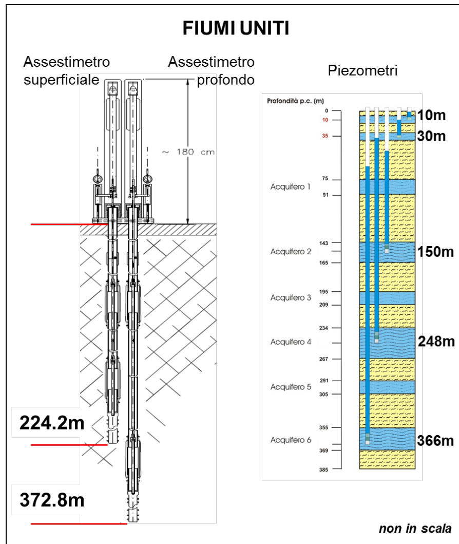
Figura 9B - Schema della stazione EPSU di Fiumi Uniti. Le profondità dei piezometri sono riferite alla quota centrale del tratto filtrante
