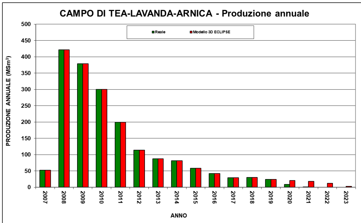
Figura 6 - Campo di TLA: produzioni (annuale) reale e da modello Eclipse dic.2019
