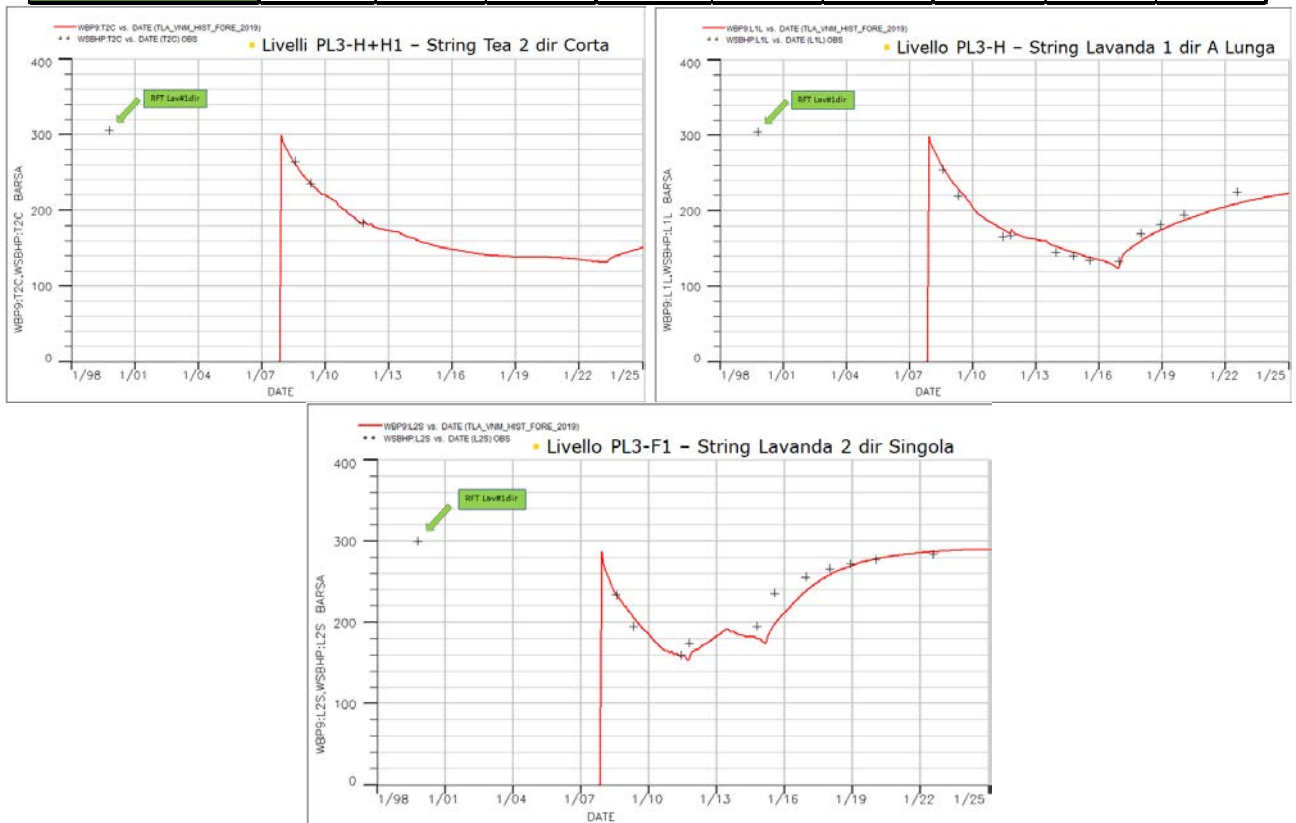
Figura 7 – Campo di TLA: confronto tra dati di pressione da profili statici e modello Eclipse dic.2019
