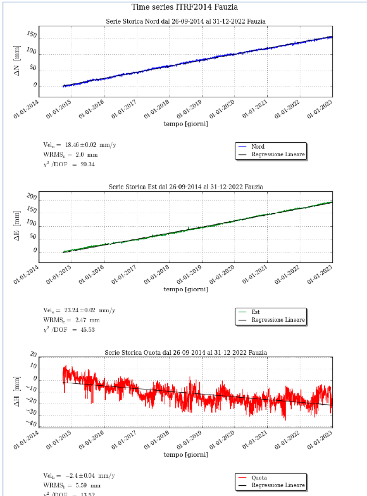
Figura 11 - Campo di Fauzia: serie storiche di misure CGPS
