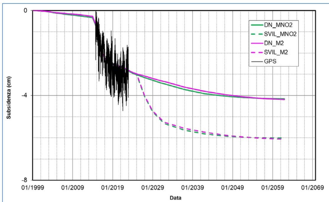
Figura 15 - Confronto fra subsidenza misurata (CGPS) e valore calcolato (modello geomeccanico marzo 2021) in corrispondenza della stazione CGPS di Fauzia
