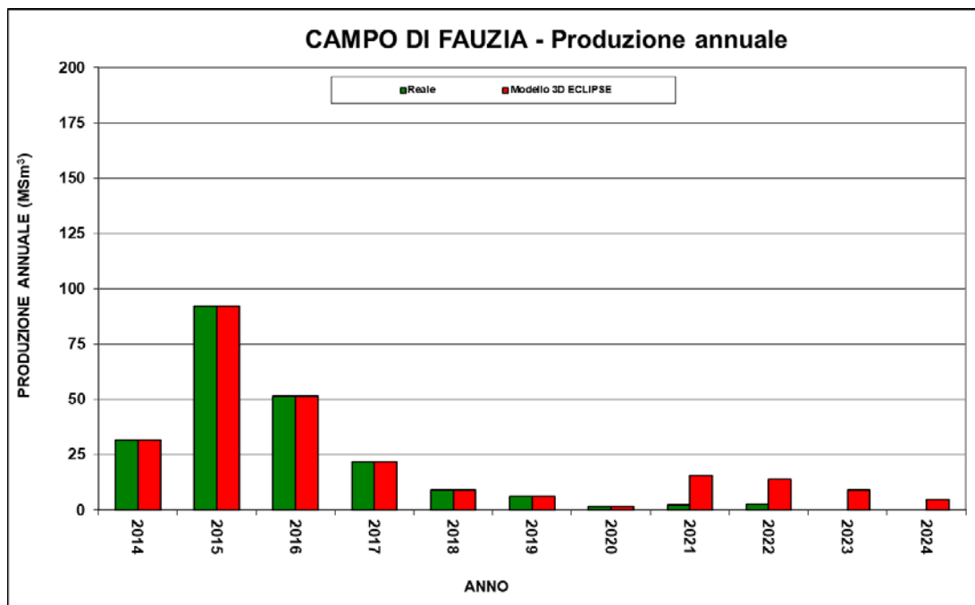
Figura 6 - Campo di Fauzia: produzione (annuale) reale e da modello Eclipse 2021
