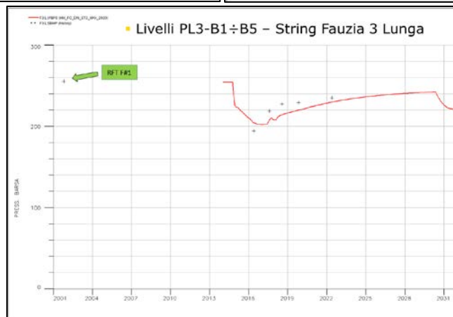
Figura 7 - Campo di Fauzia: dati di pressione (da RFT) vs. modello Eclipse 2021
