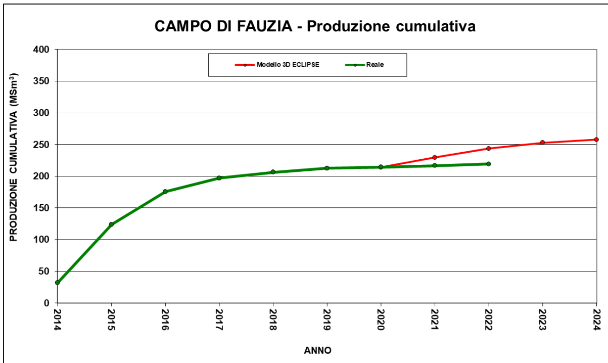
Figura 5 - Campo di Fauzia: grafico di produzione reale e da modello Eclipse 2021
