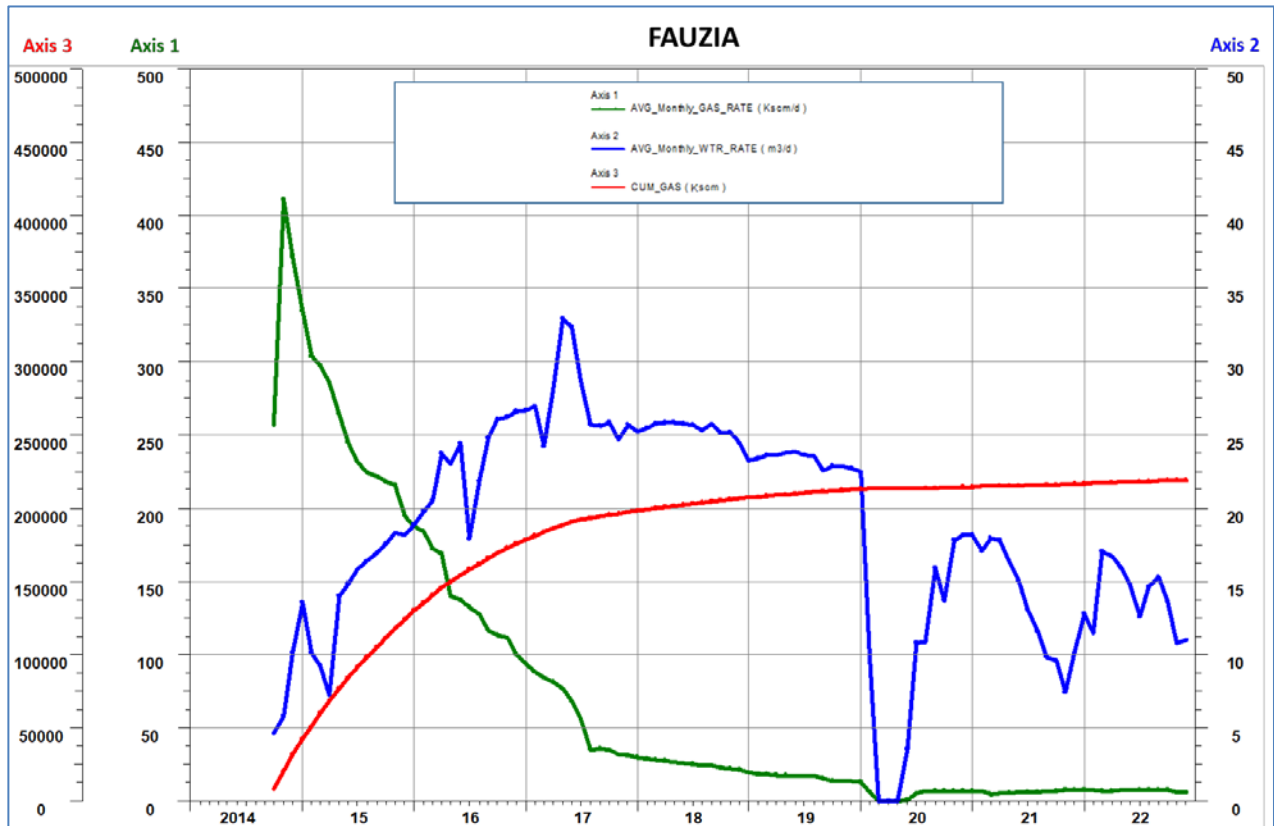
Figura 3 - Campo di Fauzia: grafico di produzione storica (agg. 31 dic. 2022)
