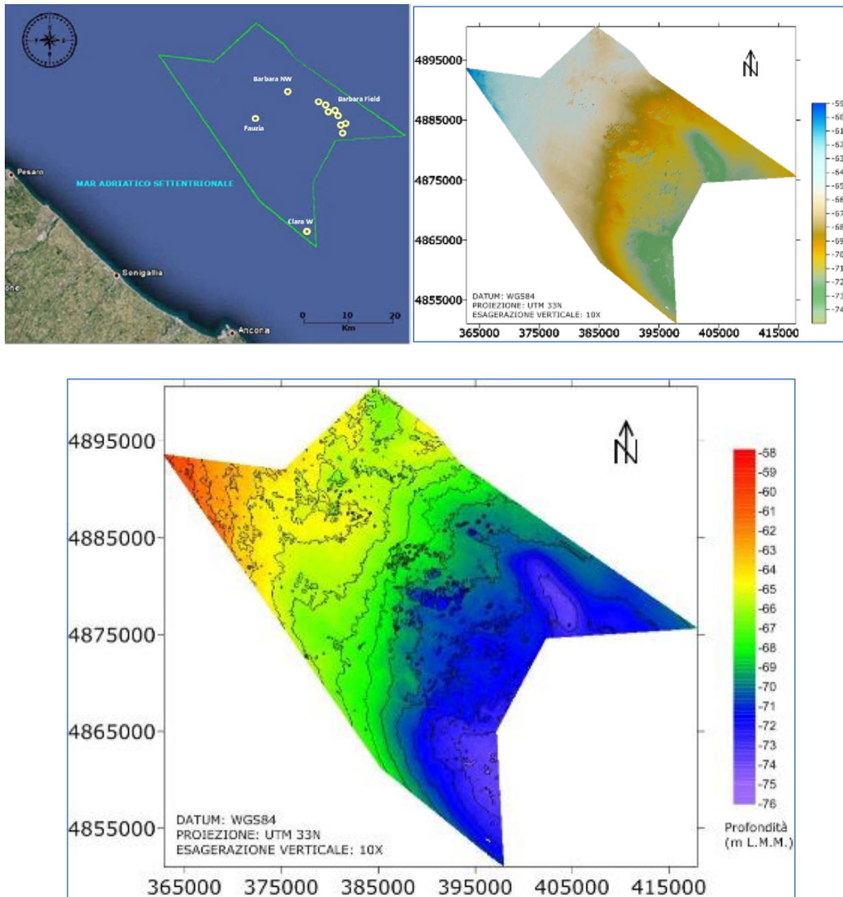
Figura 10 - Campo di Fauzia: rilievo batimetrico. In alto e a lato: ubicazione-estensione dell'area rilevata e superficie 3D dell'area indagata; in basso: la mappa delle isobate.
