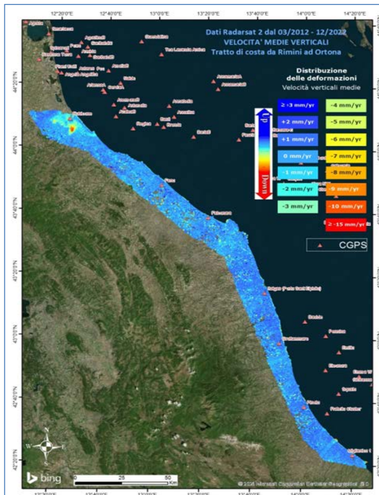
Figura 20. Distribuzione dei PS ricavati dall'elaborazione delle immagini radar da Radarsat-2. Periodo di copertura dal 2012 al 2022. Tratto di costa da Rimini ad Ortona.
