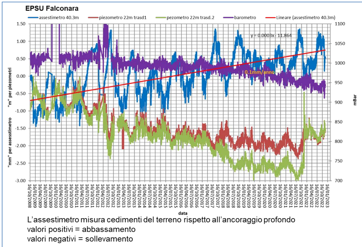
Figura 16B - Stazione EPSU di Falconara: misure piezometriche-assestimeriche e barometriche.
