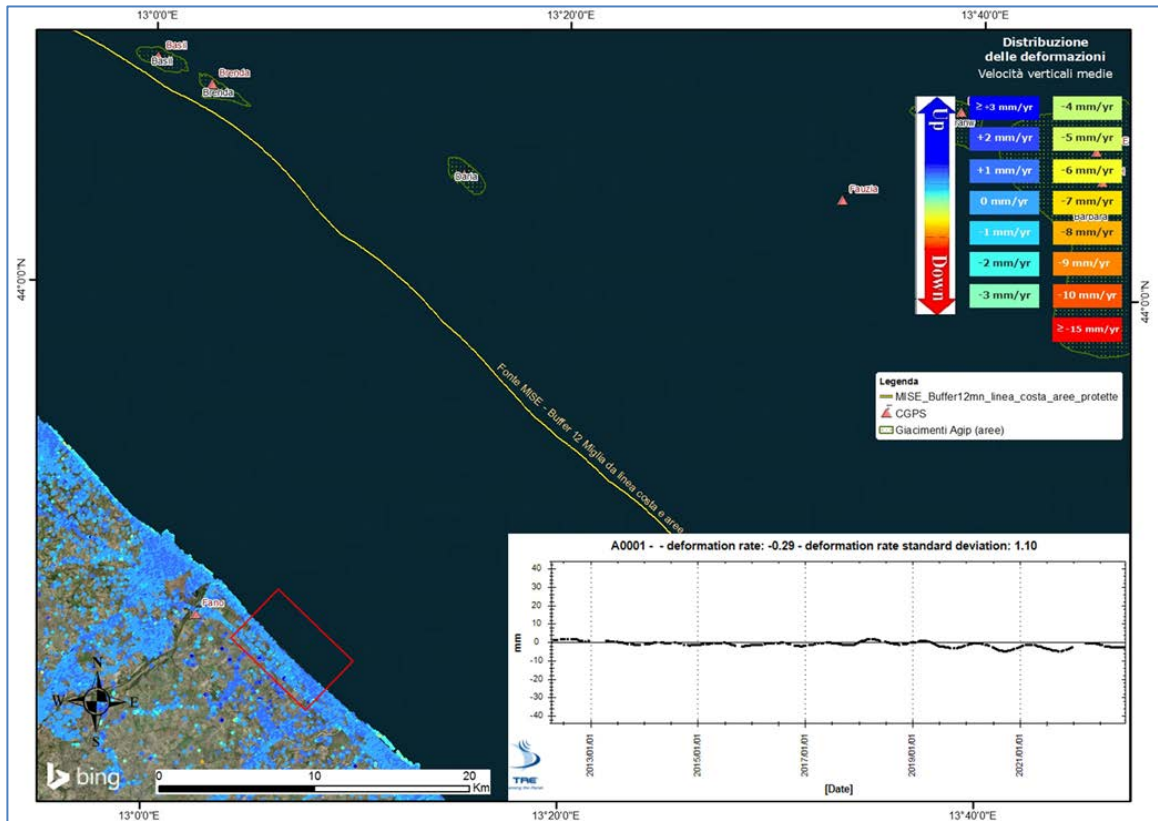
Figura 14 - Analisi dati InSAR dal 2012 al 2022 nel tratto di costa antistante il campo di Fauzia. Serie storica media (dal 2012 al 2022) dello spostamento medio ricavata dai dati InSAR all'interno del poligono rosso.
