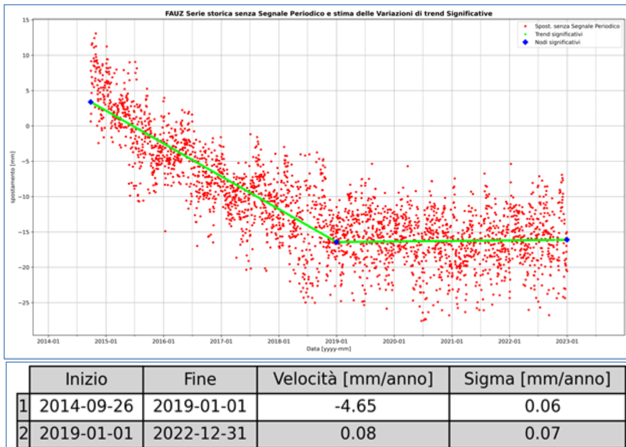
Figura 12 - Campo di Barbara NW: analisi della serie storica di misure CGPS
