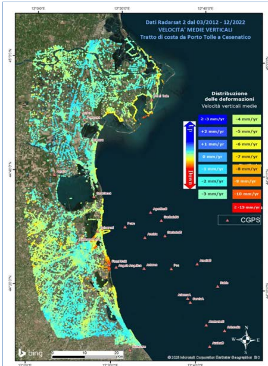
Figura 19. Distribuzione dei PS ricavati dall'elaborazione delle immagini radar da Radarsat-2. Periodo di copertura dal 2012 al 2022. Tratto di costa da Porto Tolle a Cesenatico.
