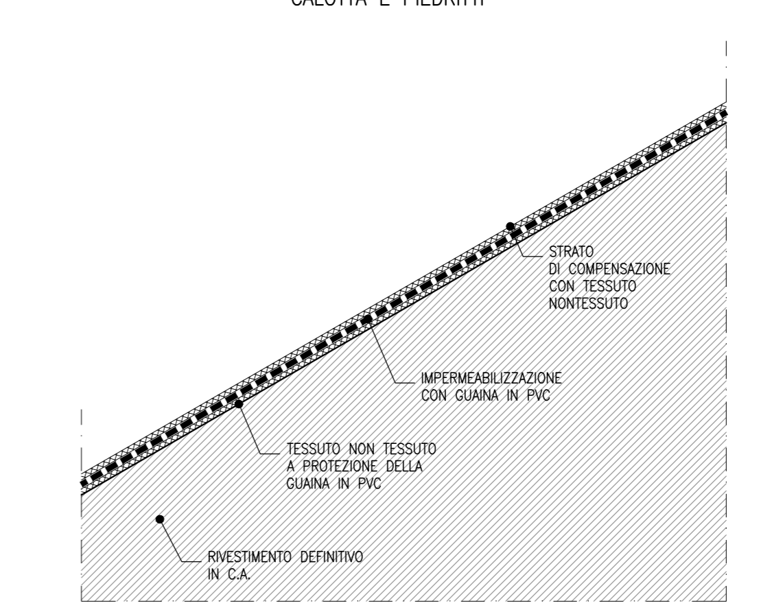
PARTICOLARE "3" SCALA 1:10 IMPERMEABILIZZAZIONE CALOTTA E PIEDRITTI
