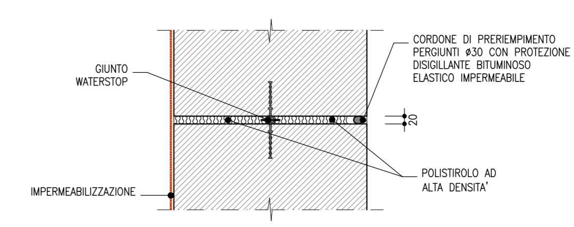
PARTICOLARE "2" SCALA 1:10 IMPERMEABILIZZAZIONE ARCO ROVESCIO E MURETTE
