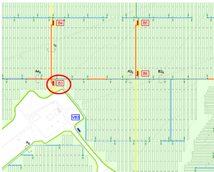
Cabina MT/BT in prossimità del ricettore R2
