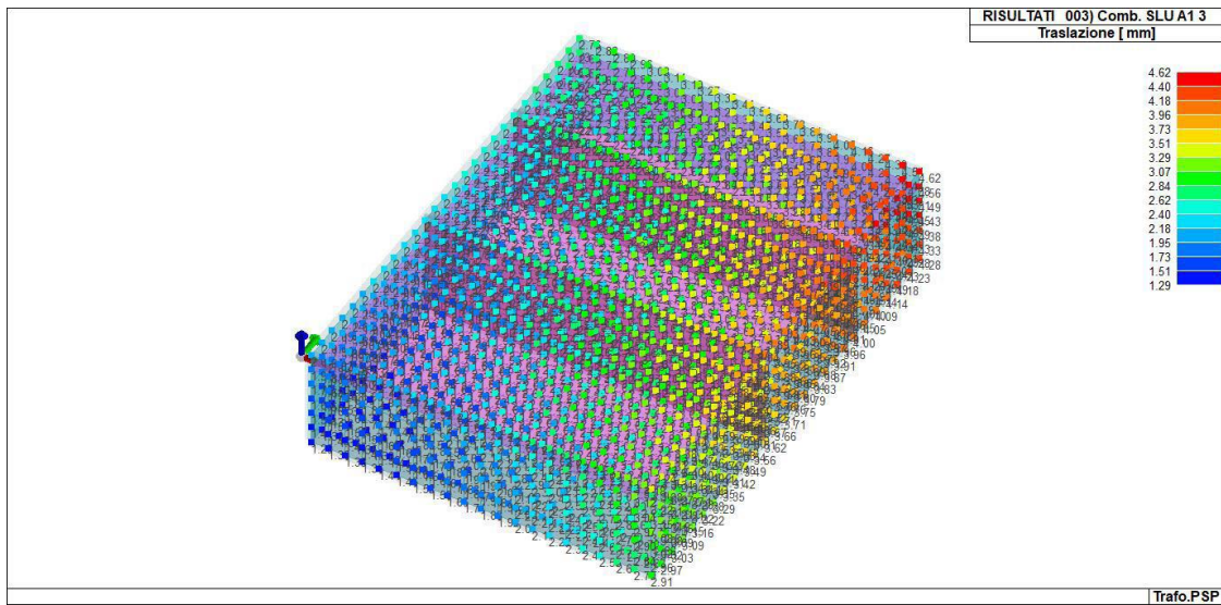
Figura 15-1 RIS_SPOSTAMENTI_003_Comb. SLU A1 3
