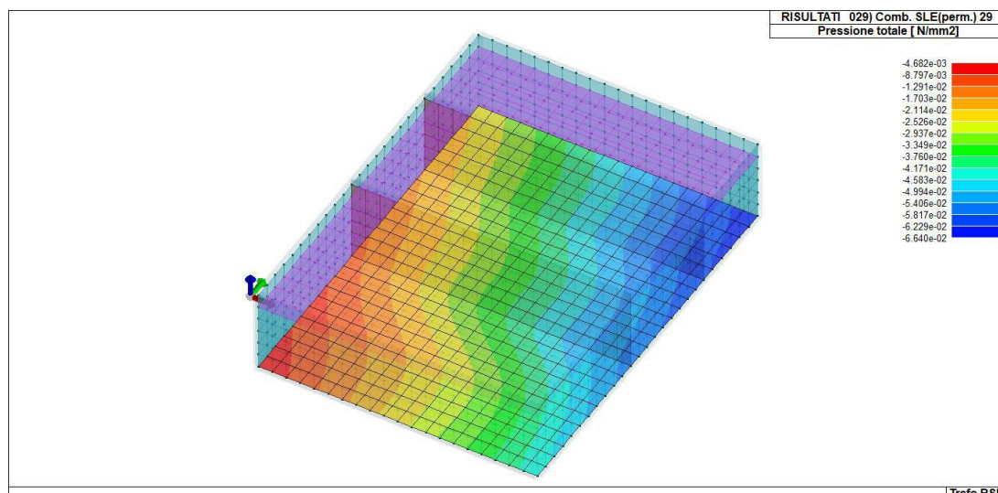
Figura 16-9 RIS_PRESSIONI_029_Comb. SLE(perm.) 29
