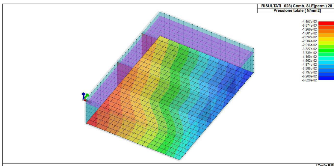
Figura 16-8 RIS_PRESSIONI_028_Comb. SLE(perm.) 28
