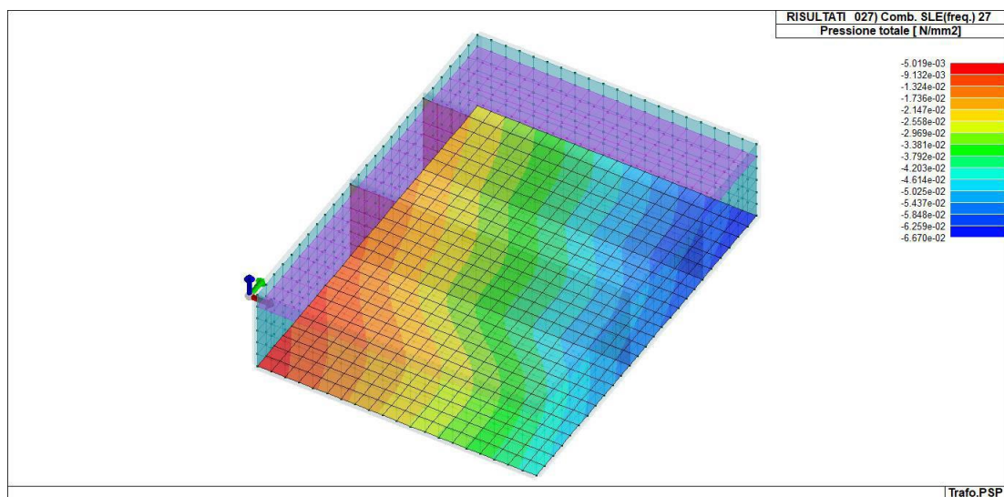
Figura 16-7 RIS_PRESSIONI_027_Comb. SLE(freq.) 27
