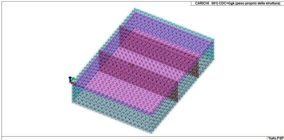
Figura 11-1 CDC_001_CDC=Ggk (peso proprio della struttura)
