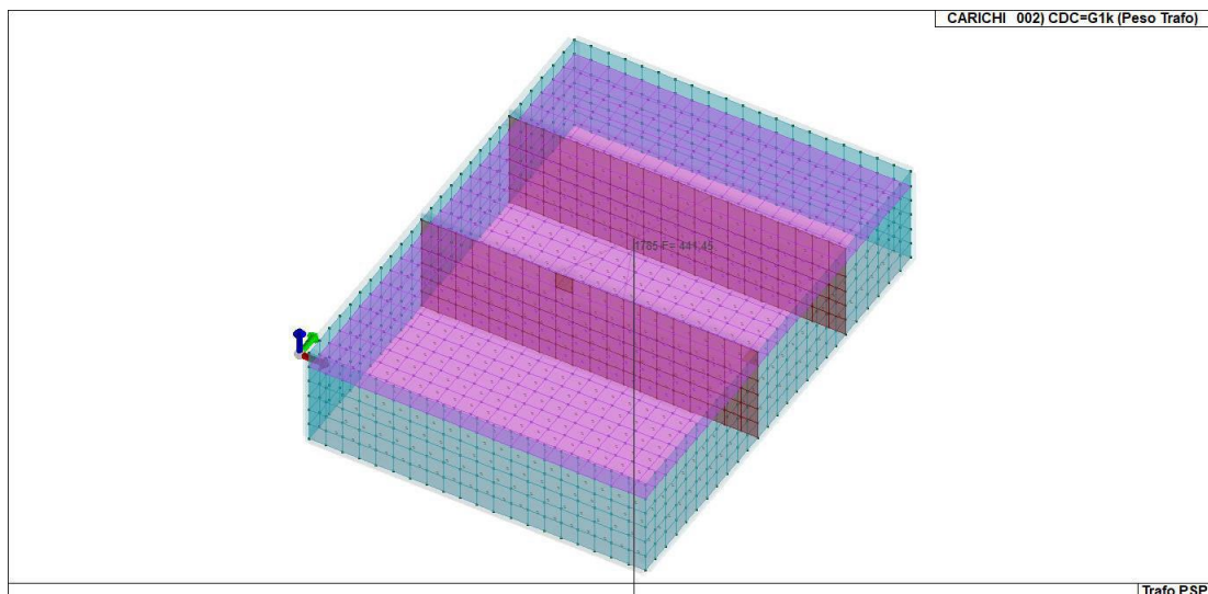
Figura 11-2 CDC_002_CDC=G1k (Peso Trafo)
