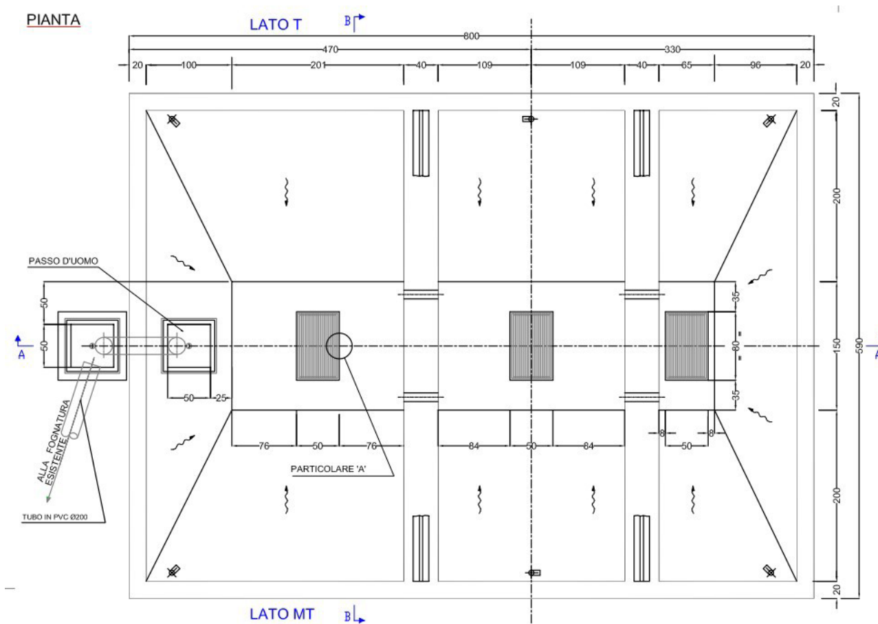
Figura 1-1 Pianta struttura supporto trafo
