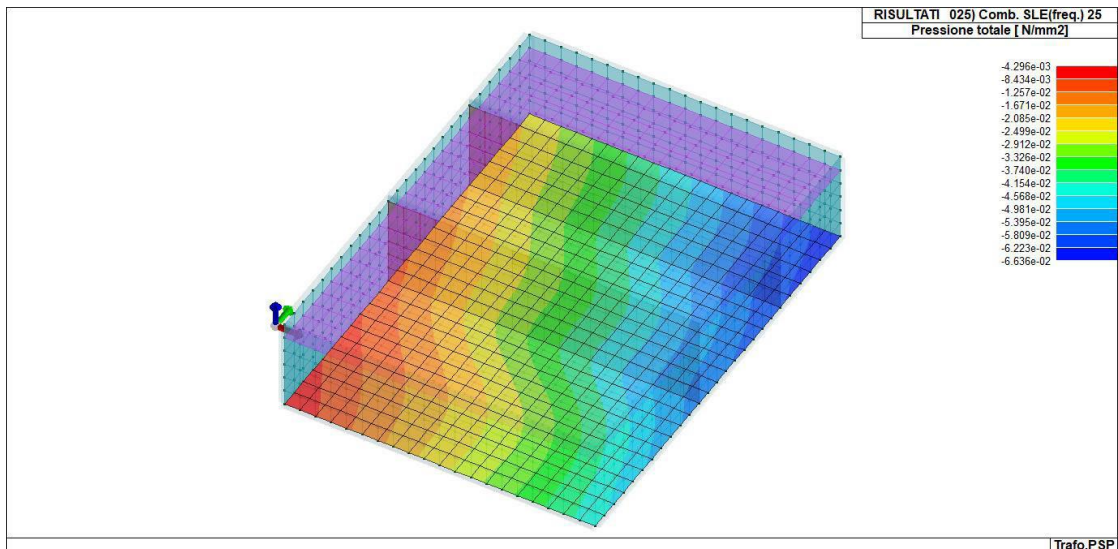
Figura 16-6 RIS_PRESSIONI_025_Comb. SLE(freq.) 25
