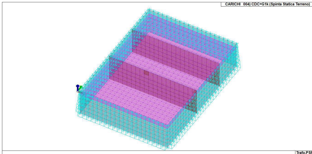
Figura 11-4 CDC_004_CDC=G1k (Spinta Statica Terreno)
