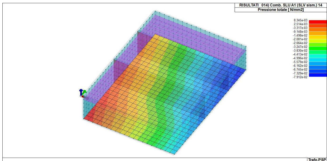
Figura 16-3 RIS_PRESSIONI_014_Comb. SLU A1 (SLV sism.) 14
