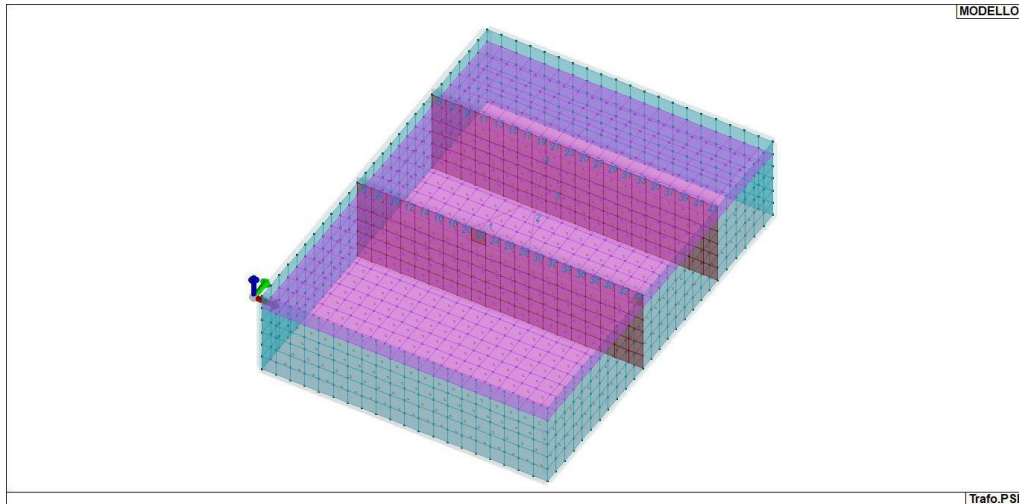
Figura 8-1 MOD_NUMERAZIONE_D2
