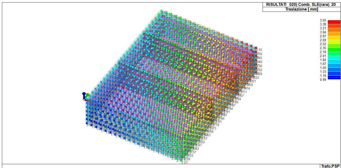
Figura 15-3 RIS_SPOSTAMENTI_020_Comb. SLE(rara) 20
