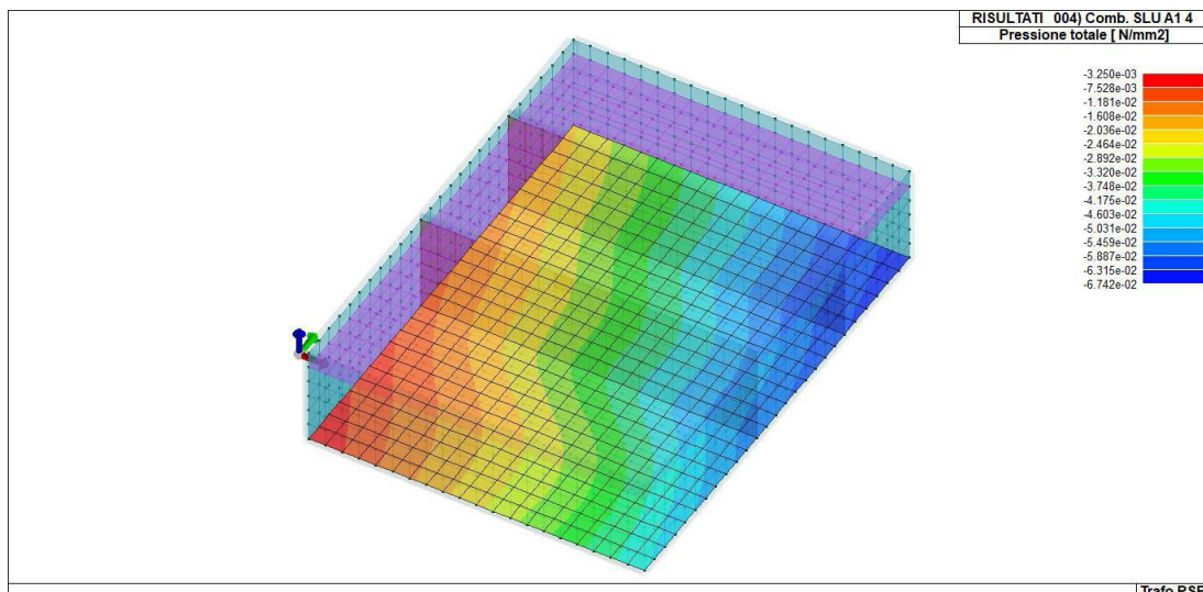
Figura 16-1 RIS_PRESSIONI_004_Comb. SLU A1 4
