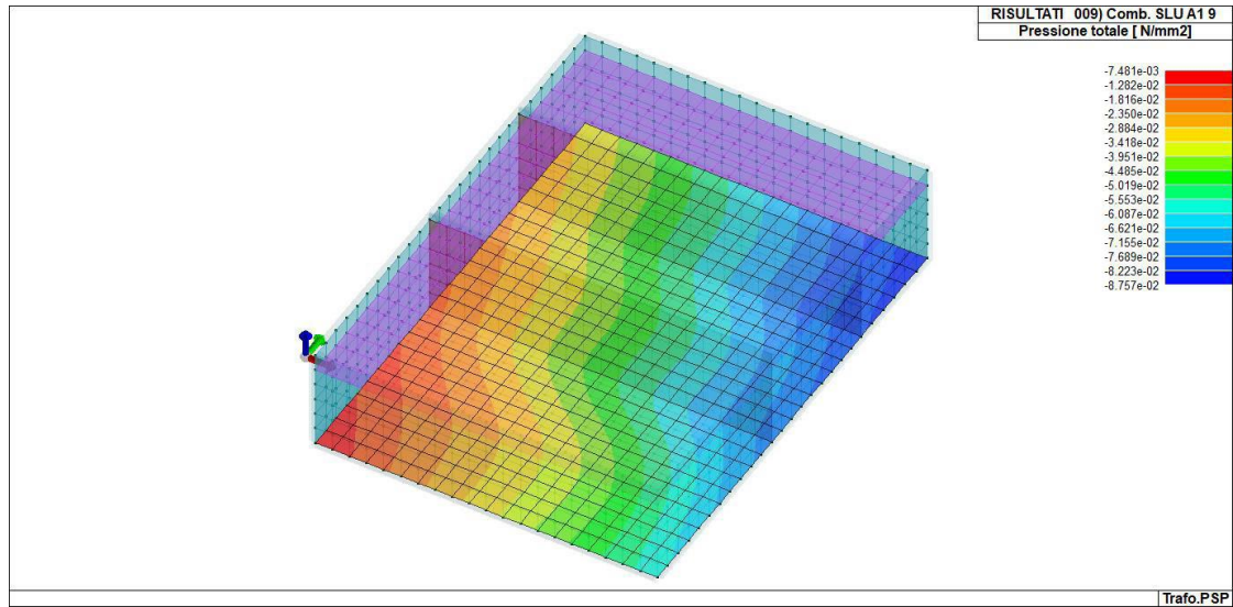
Figura 16-2 RIS_PRESSIONI_009_Comb. SLU A1 9
