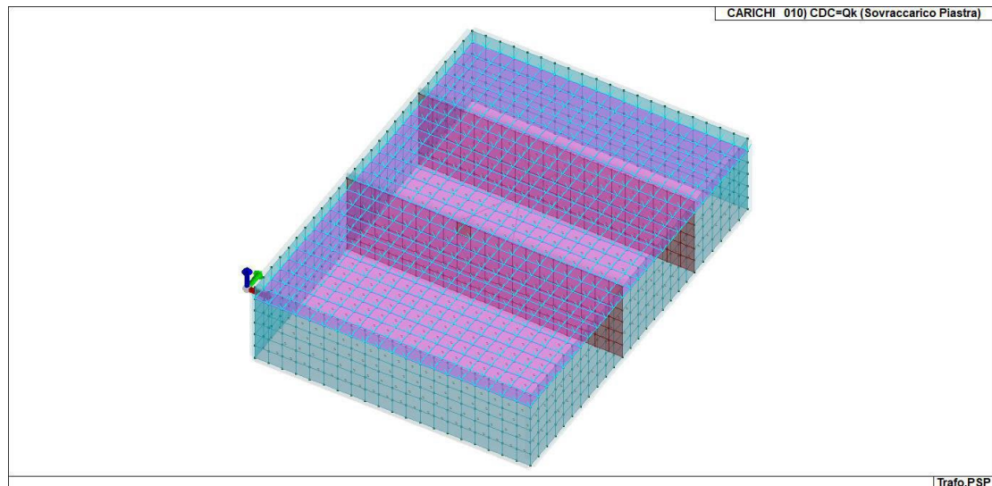
Figura 11-10 CDC_010_CDC=Qk (Sovraccarico Piastra)
