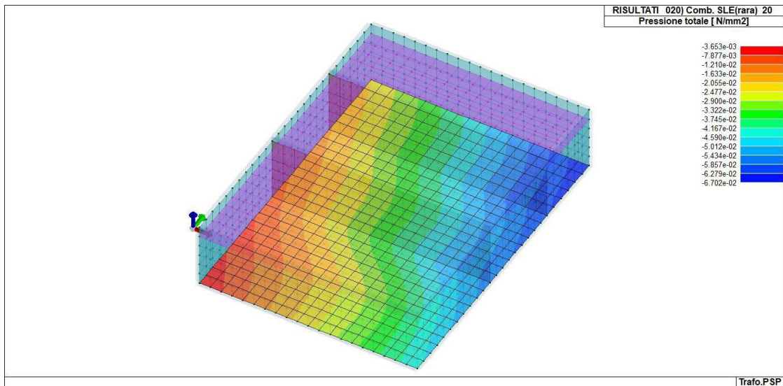
Figura 16-4 RIS_PRESSIONI_020_Comb. SLE(rara) 20
