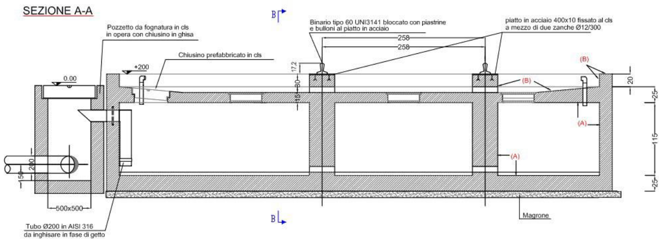
Figura 1-2 Sezione struttura supporto trafo
