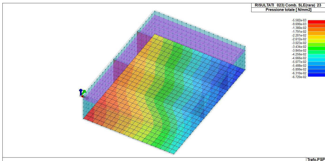
Figura 16-5 RIS_PRESSIONI_023_Comb. SLE(rara) 23
