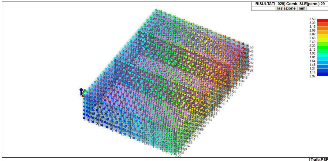
Figura 15-5 RIS_SPOSTAMENTI_029_Comb. SLE(pern.) 29
