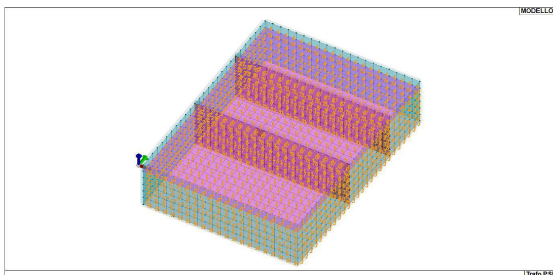
Figura 9-2 MOD_NUMERAZIONE_D3_PARETI
