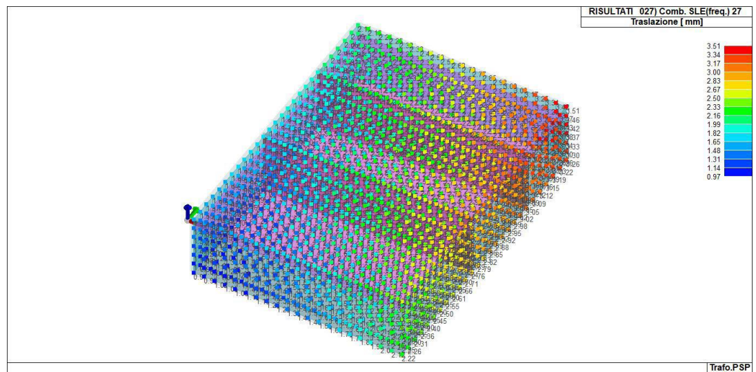
Figura 15-4 RIS_SPOSTAMENTI_027_Comb. SLE(freq.) 27
