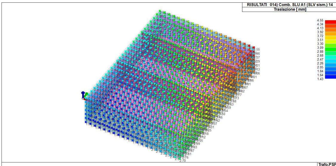
Figura 15-2 RIS_SPOSTAMENTI_014_Comb. SLU A1 (SLV sism.) 14
