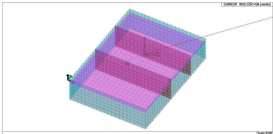
Figura 11-3 CDC_003_CDC=Qk (vento)
