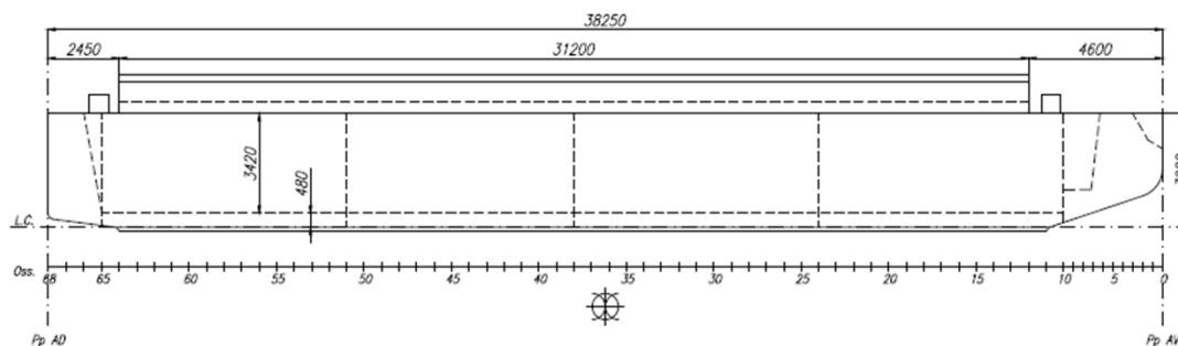
VISTA LONGITUDINALE
