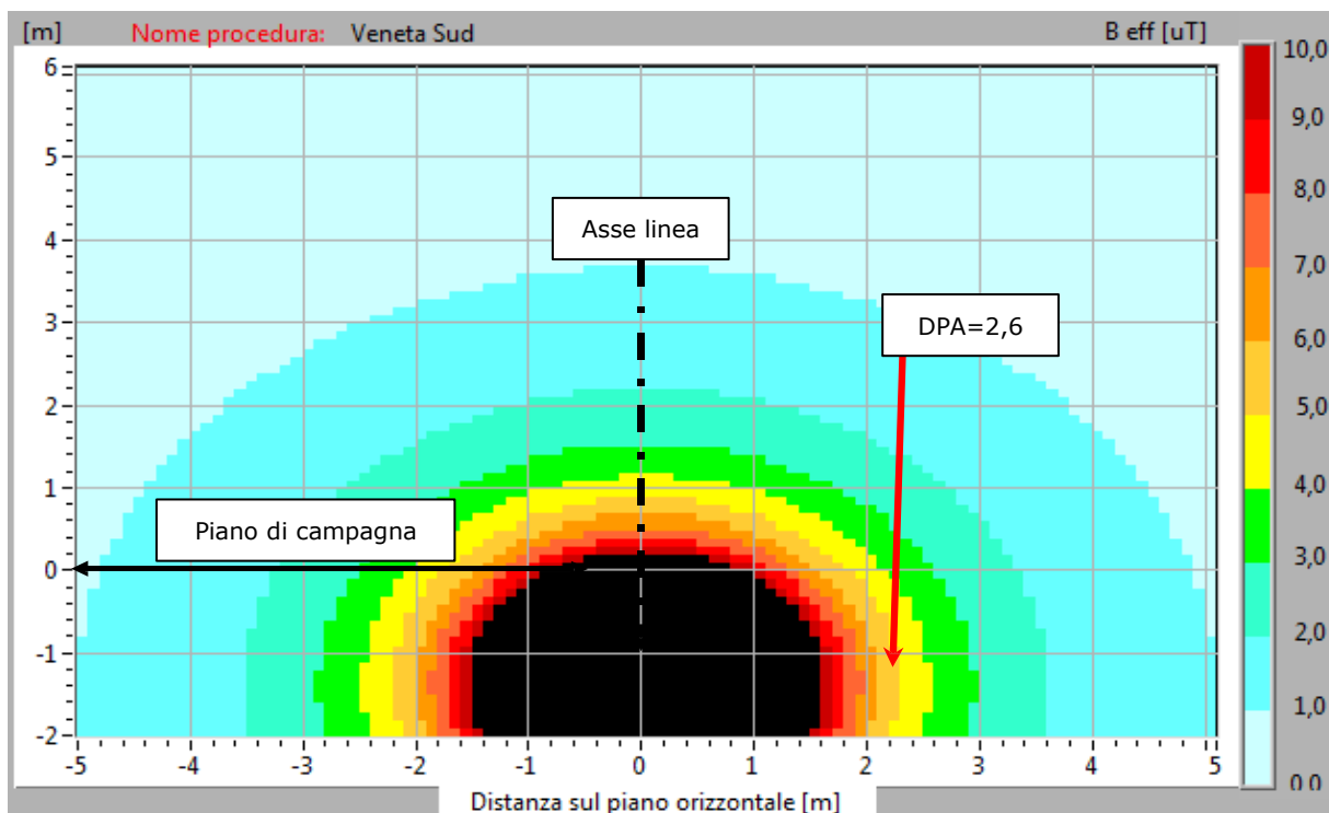
Figura 4 - Mappa verticale induzione magnetica (B) sezione tipo con indicazione della DPA - V=150\text{ kV} I = 900\text{ A}
