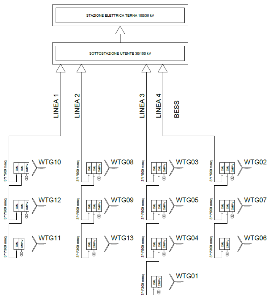
Schema elettrico unifilare parco eolico
