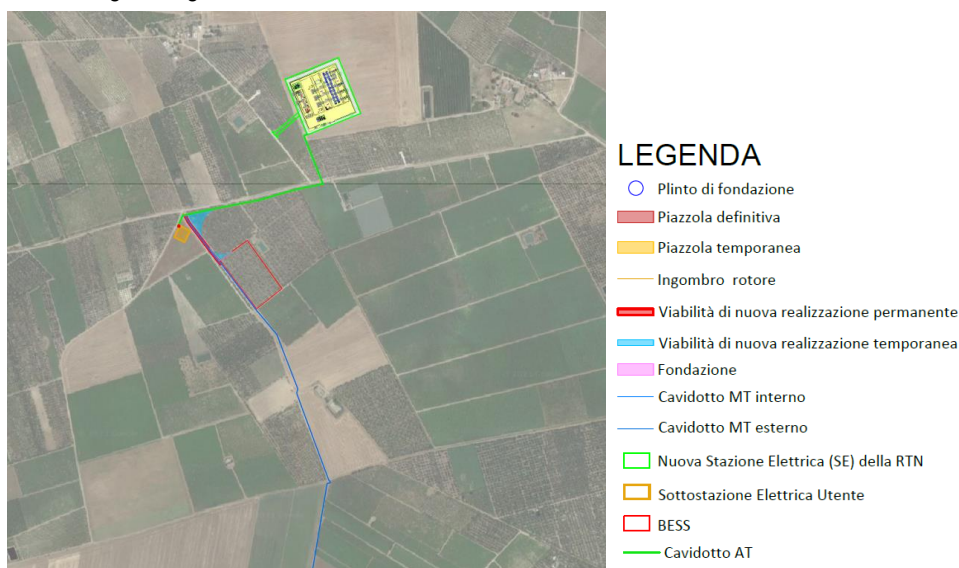
Layout impianto con posizionamento BESS
