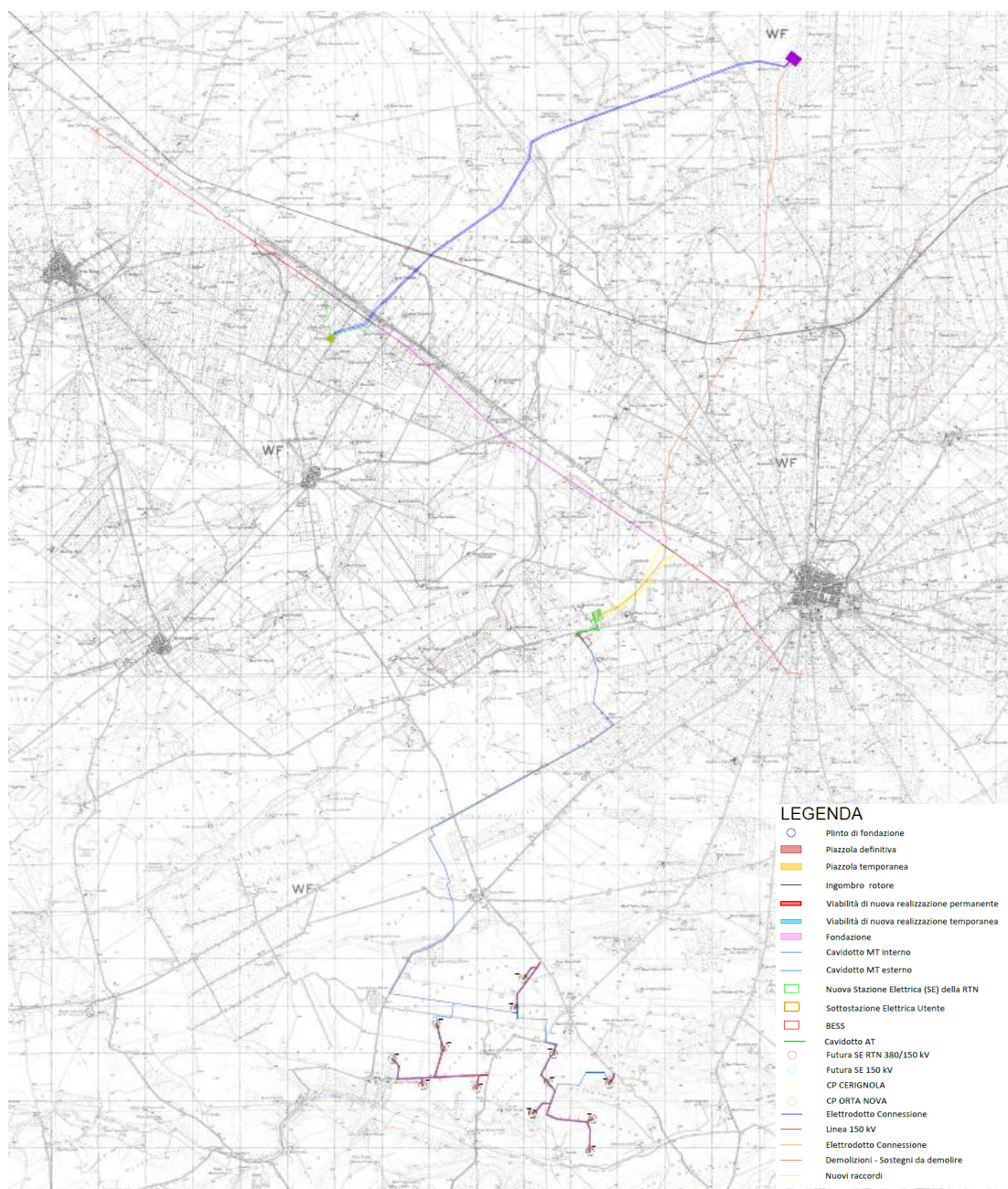
Planimetria soluzione di connessione
