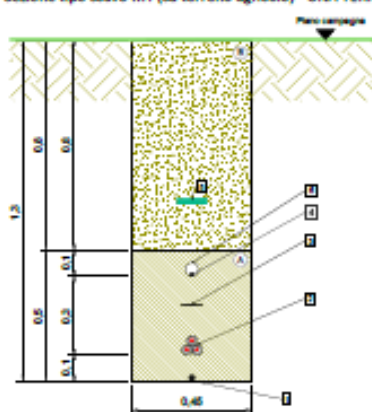
Sezione tipo posa cavidotto a 1 terna MT su terreno agricolo
