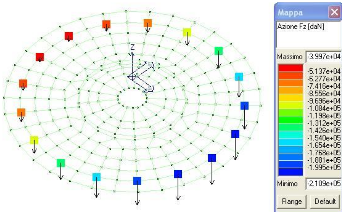
Mappa cromatica delle massime azioni di sforzo normale sui pali – Combinazione 7) SLE RA (c)
