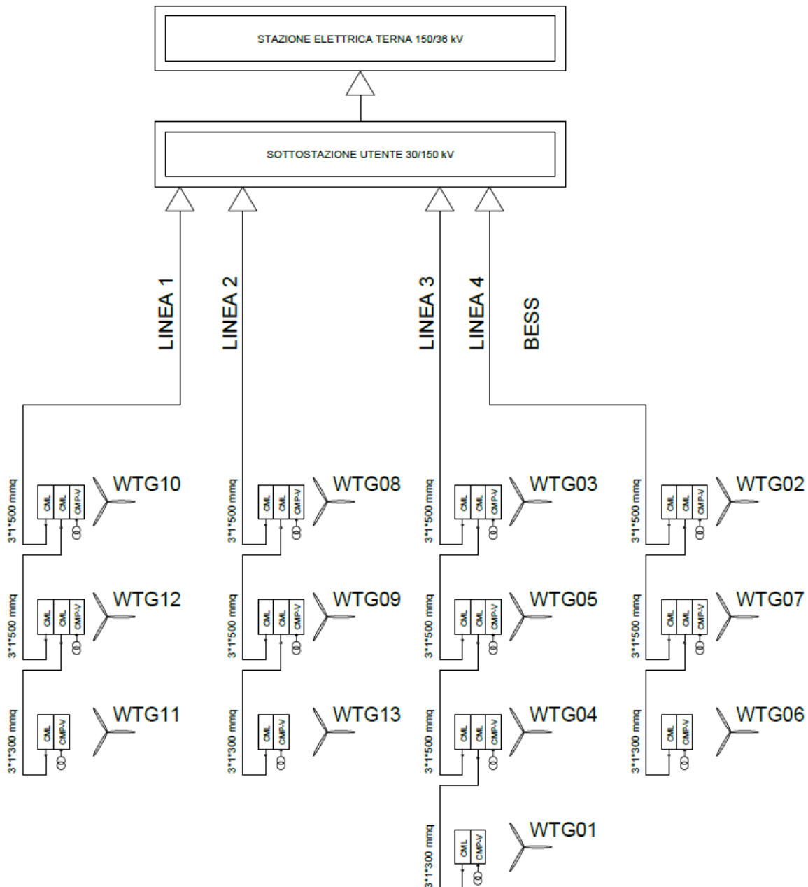
Schema Unifilare WTG
