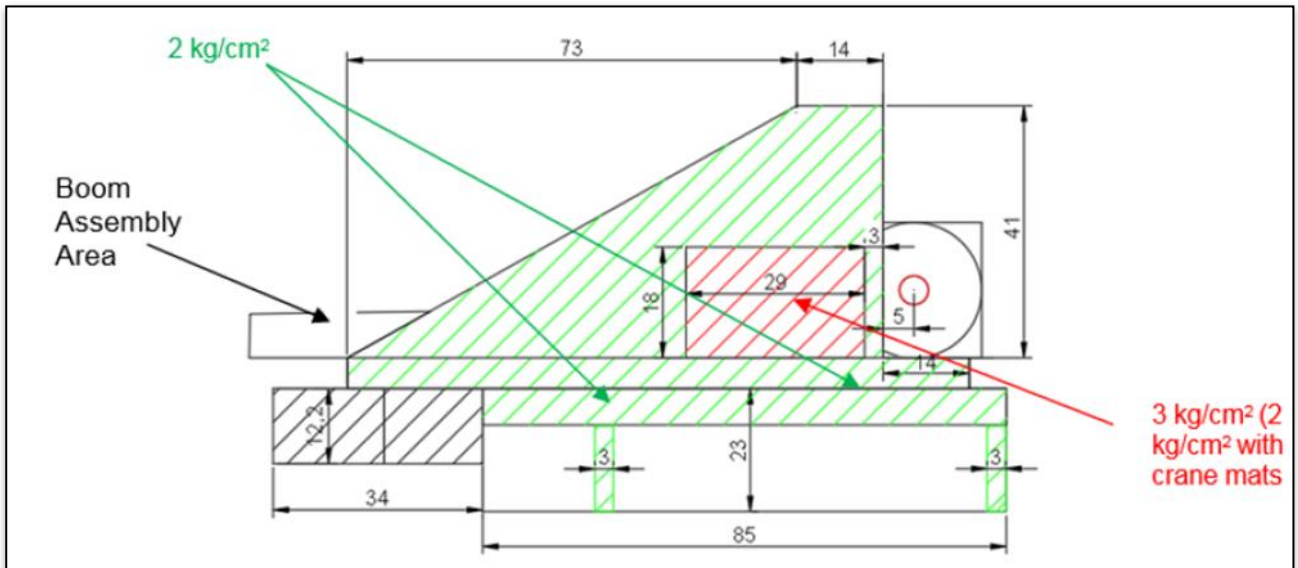
Schema della piazzola temporanea e dell'area di cantiere
