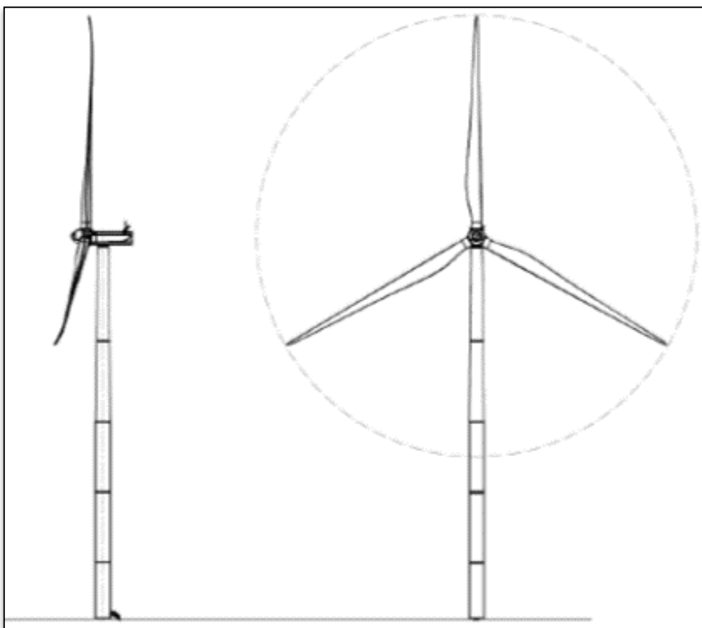
Prospetti dell'aerogeneratore tipo SIEMENS GAMESA SG 6.0 - 170
