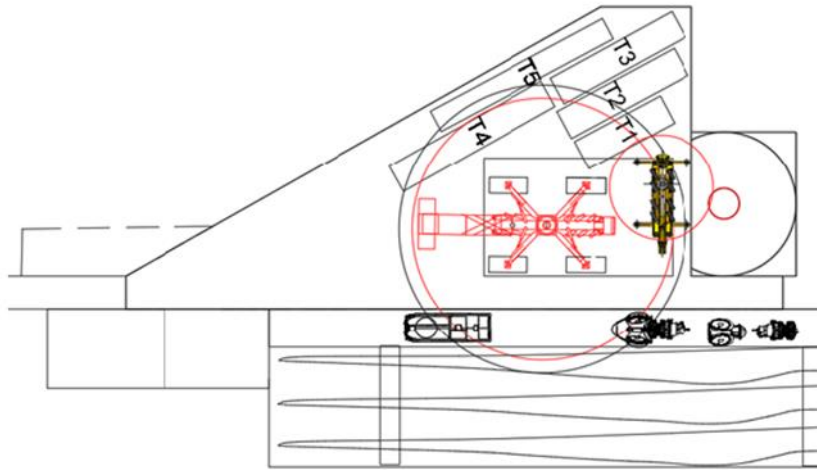
Particolare della piazzola di esercizio
