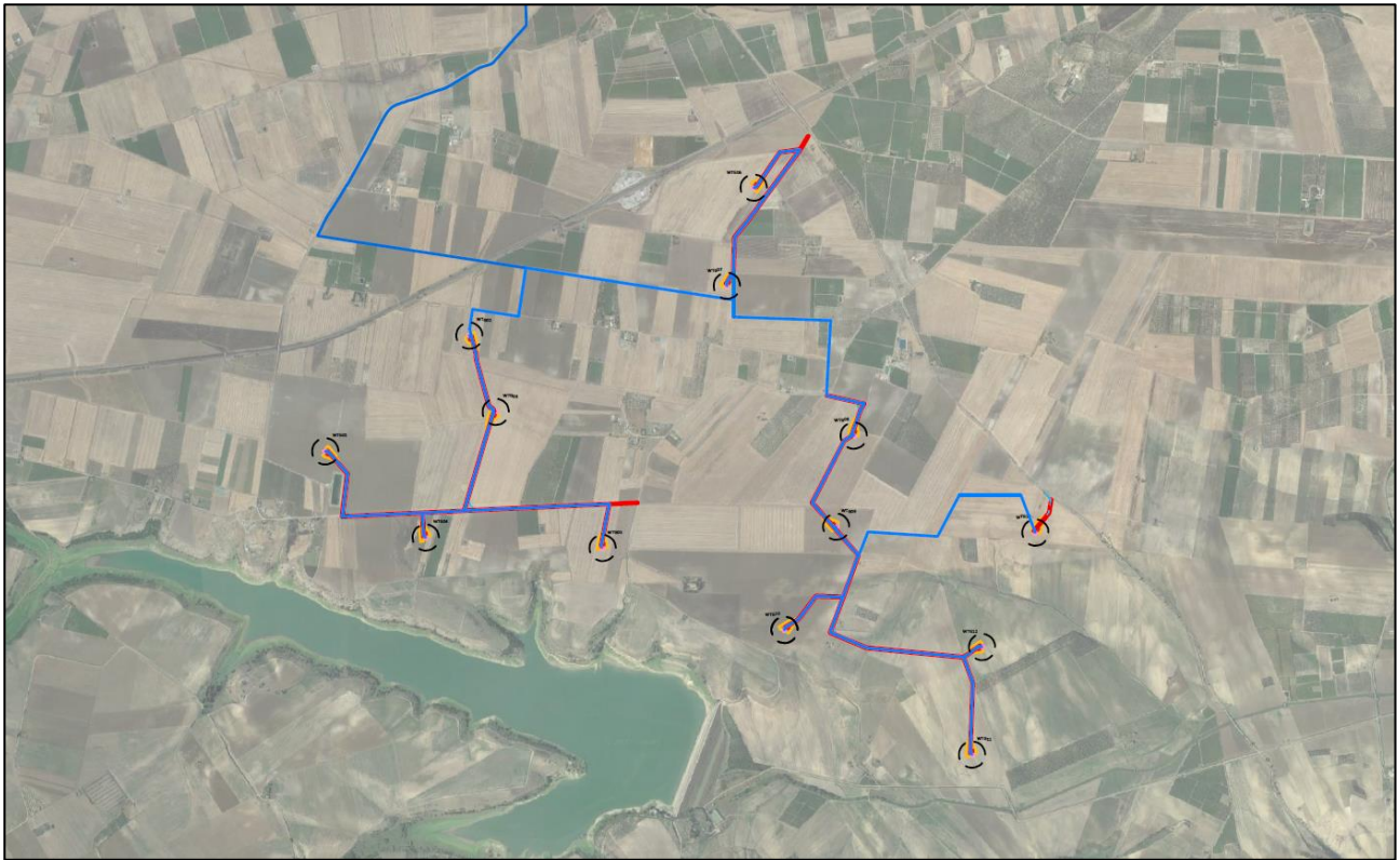
Planimetria di progetto – Aerogeneratori su Ortofoto
