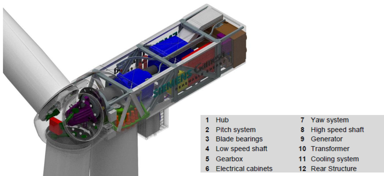
Dettaglio rotore
