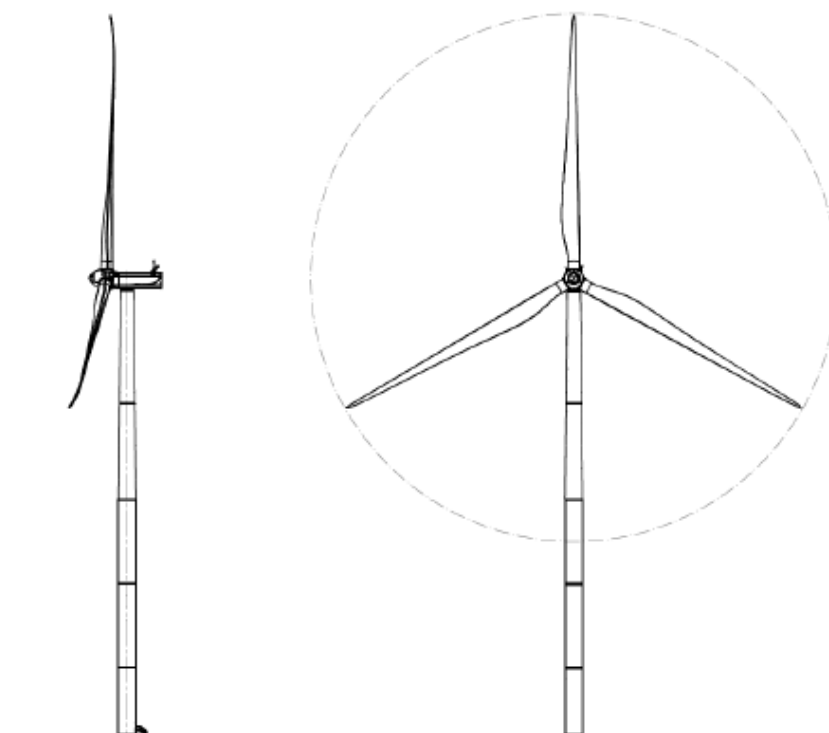
Prospetto aerogeneratore
