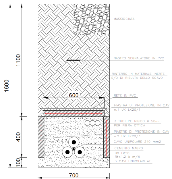
CAVIDOTTO AT INTERRATO SEMPLICE TERNA PERCORSO STERRATO/MASSICIATA scala 1:20
