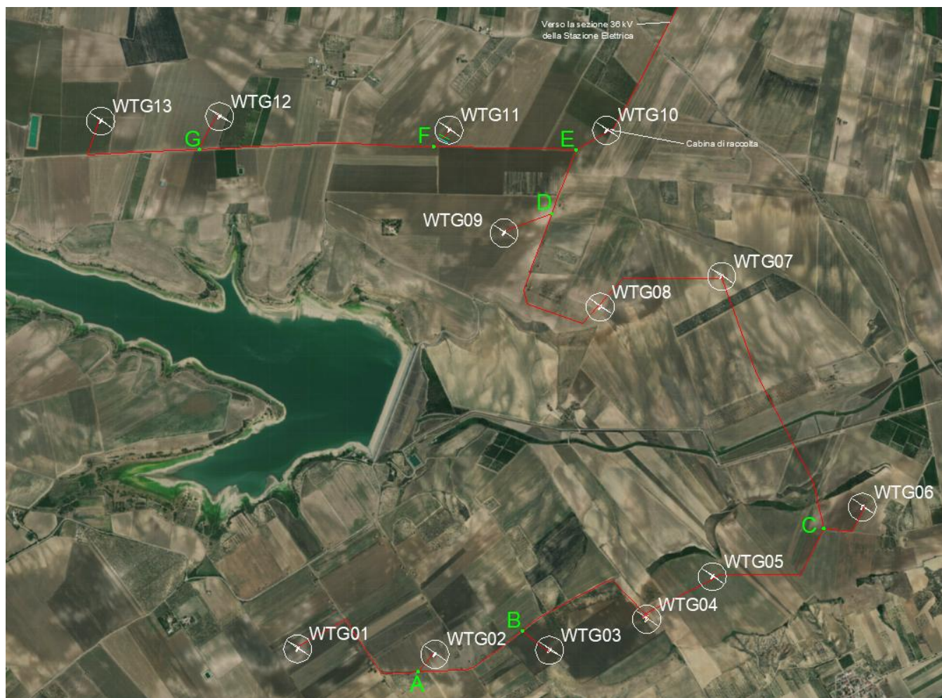
Figura 3 - Inquadramento su ortofoto del layout impianto
