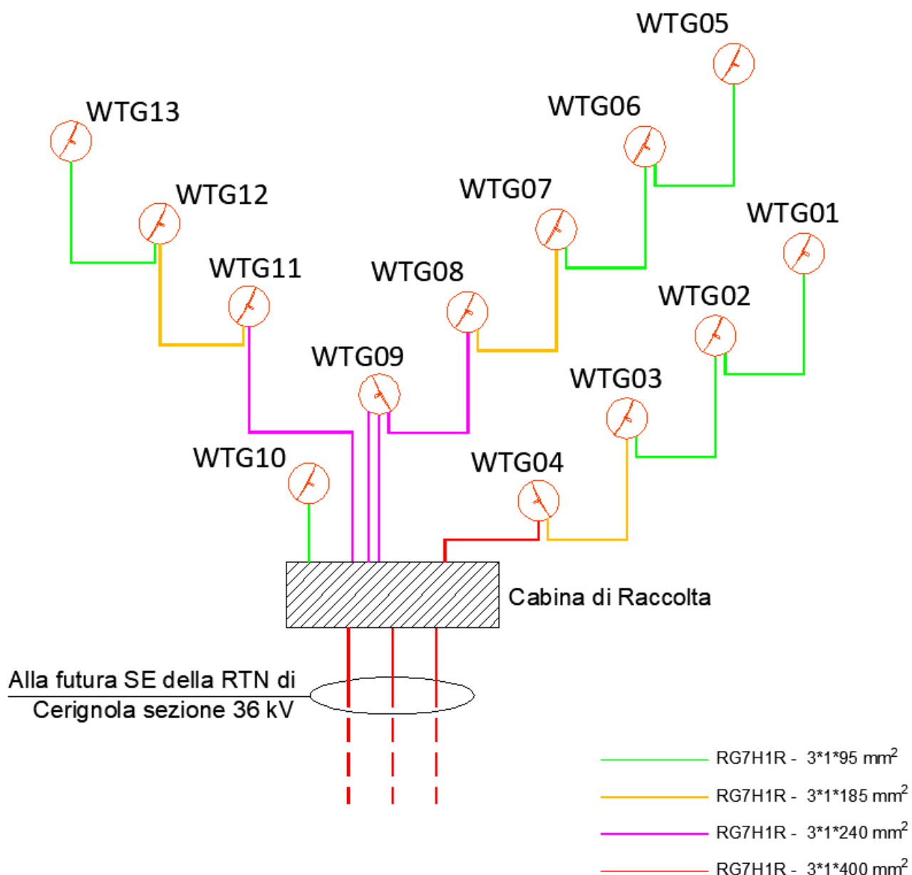
Figura 4 - Schema di connessione elettrica dell'impianto eolico in progetto
