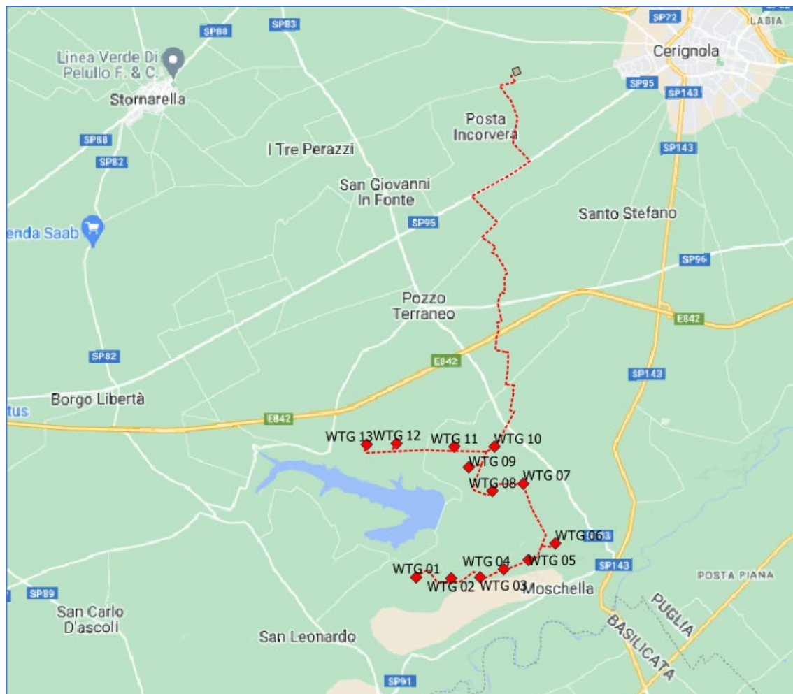
Figura 6 - Inquadramento strade di accesso
