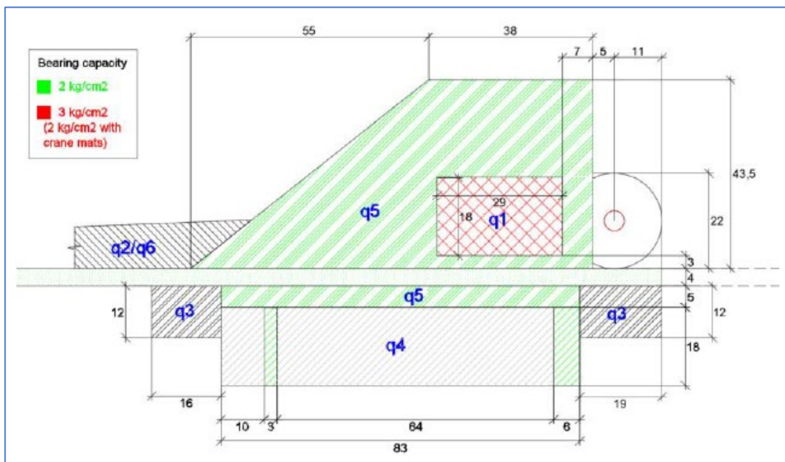
Figura 14 – tipologico della piazzola di montaggio
