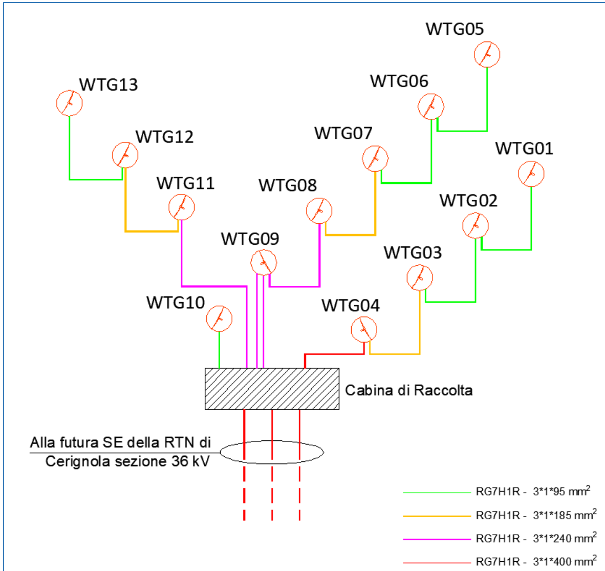
Figura 53 - Schema di connessione elettrica dell'impianto eolico in progetto
