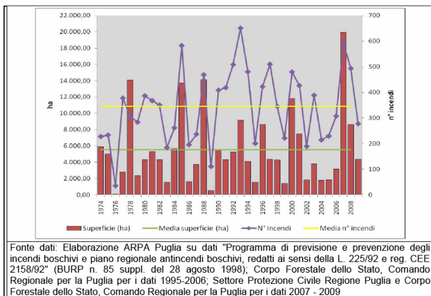
Figura 18 - Andamento del numero e della superficie degli incendi boschivi, periodo 1974 - 2009
