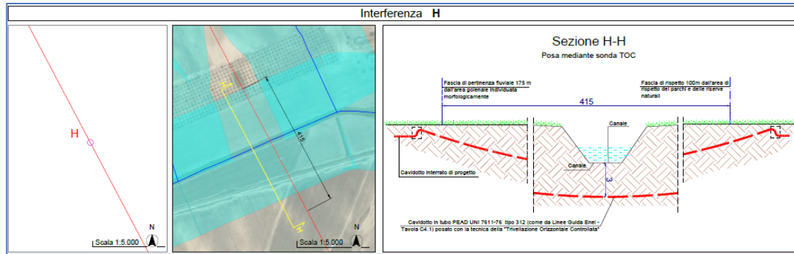
Figura 54 - Stralcio studio degli attraversamenti – “CRE-CIV-TAV-017 – Studio degli attraversamenti”
