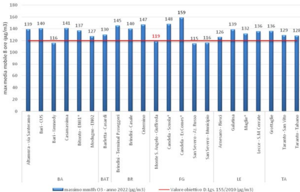
Figura 10 -Massimo della media mobile sulle 8 ore per l'O3 (µg/m3) – anno 2022
