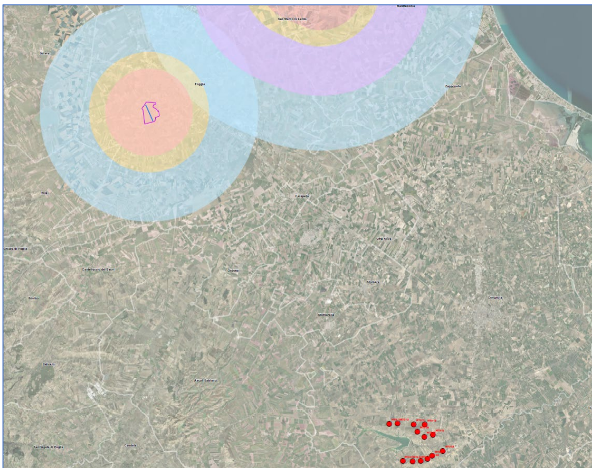
Figura 50 – Interferenze con le infrastrutture di volo stralcio tavola CRE_AMB_TAV_053_01
