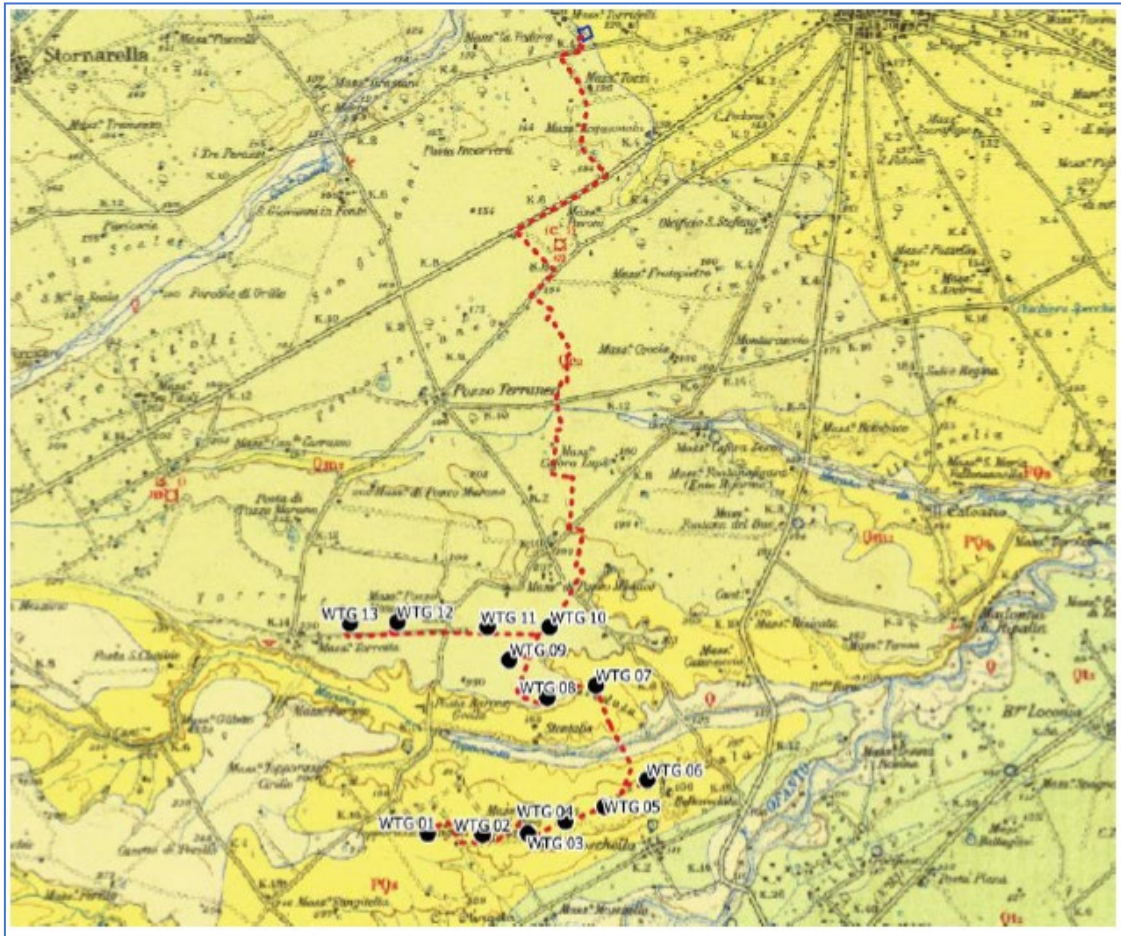
Figura 12 – Stralcio della Carta Geologica d'Italia
