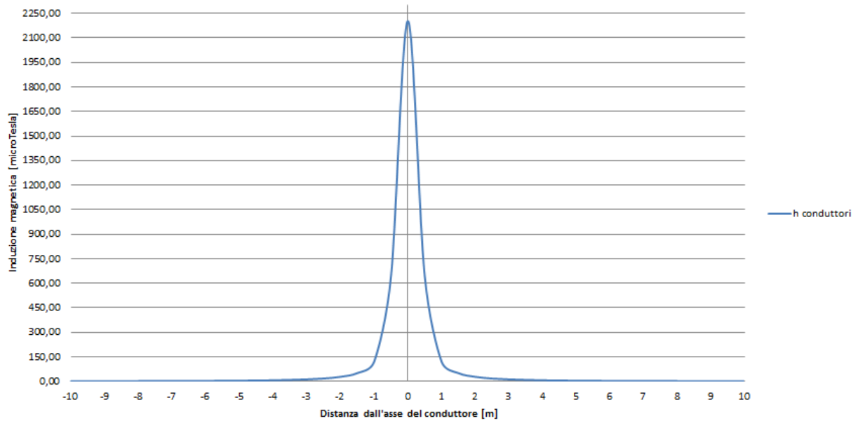
Andamento del campo magnetico - Sbarre MT stazione elettrica 150/30 kV
