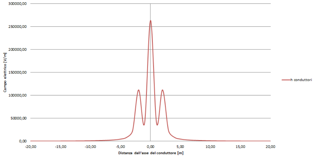
Andamento del campo elettrico - Sbarre AT stazione elettrica 150/30 kV
