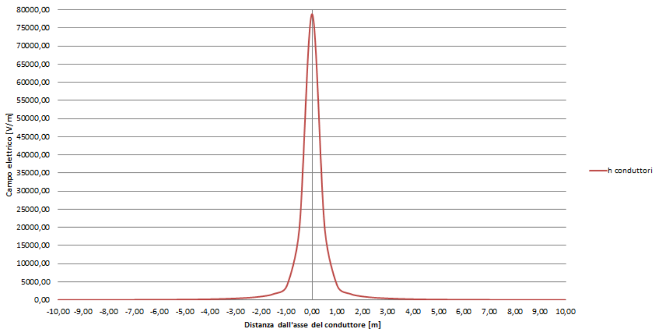
Andamento del campo elettrico - Sbarre MT stazione elettrica 150/30 kV
