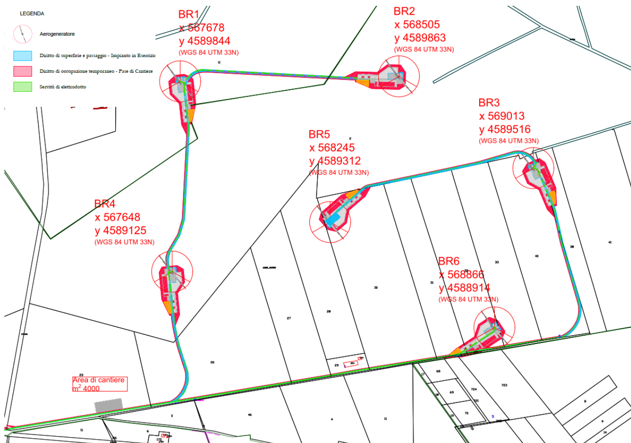
Figura 4 – Rappresentazione grafica generale aree di occupazione e servitù (1/2)
