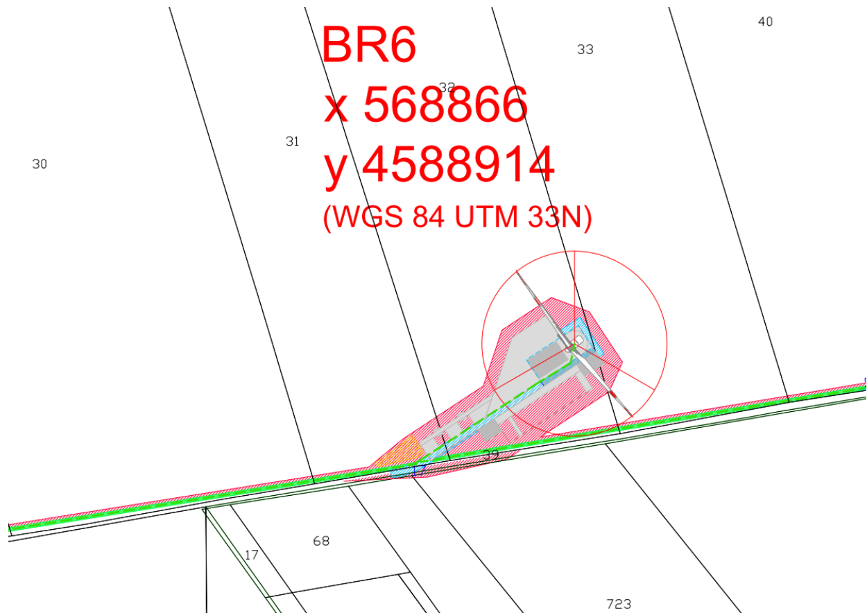
Figura 6 – Dettaglio strade di accesso-aree provvisorie e definitive
