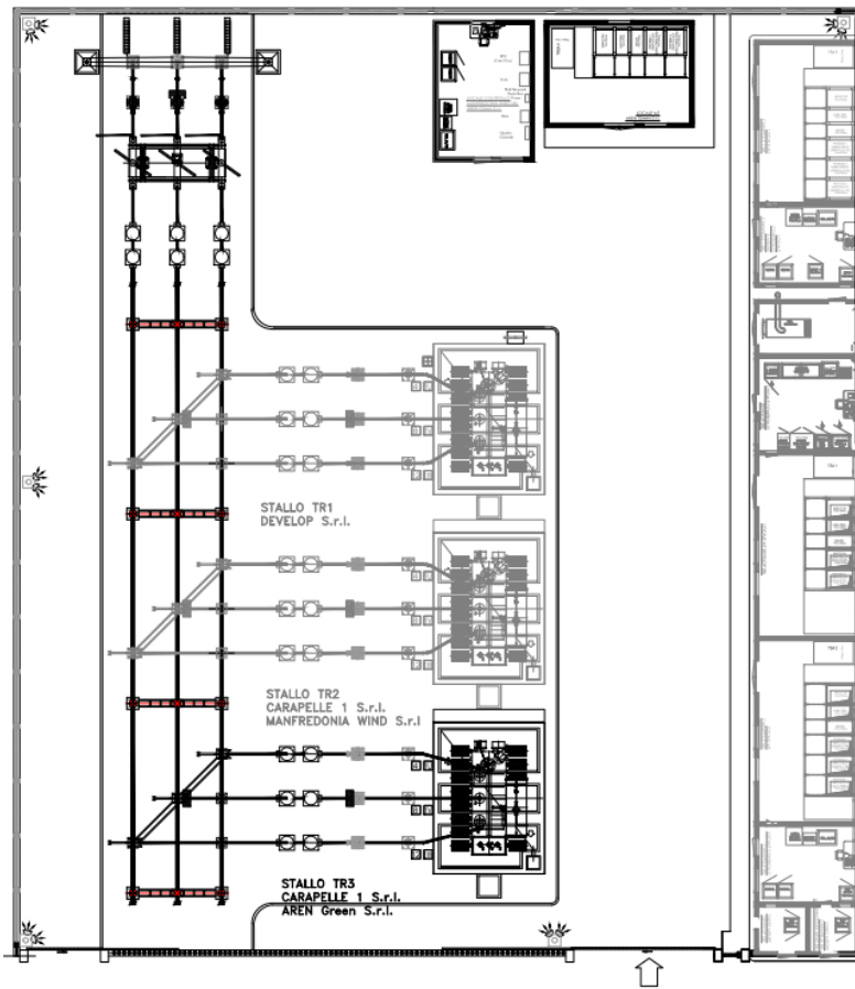
Figura 12 – Localizzazione della SSE (2/2)
