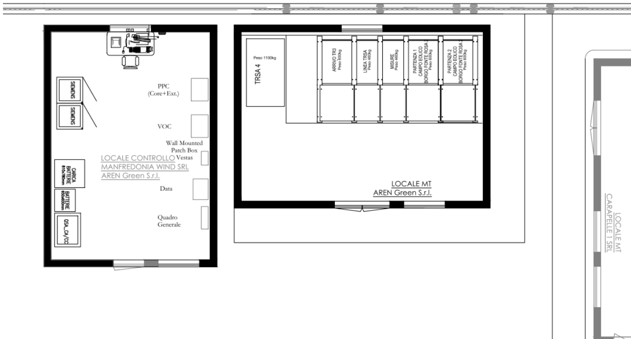
Figura 14 - Planimetria del Locale Controllo e Locale MT (2/2)
