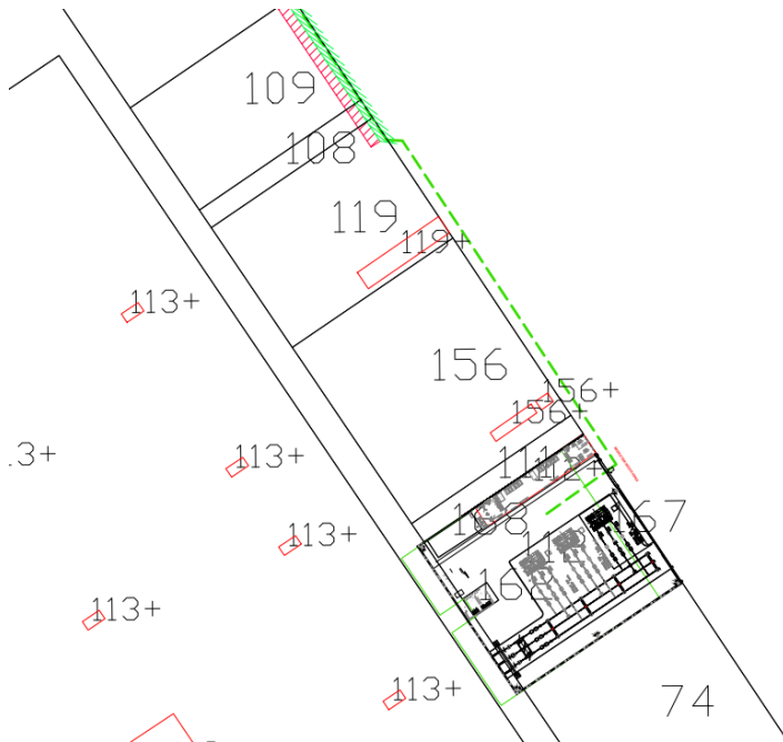
Figura 12 – Localizzazione della SSE (2/2)
