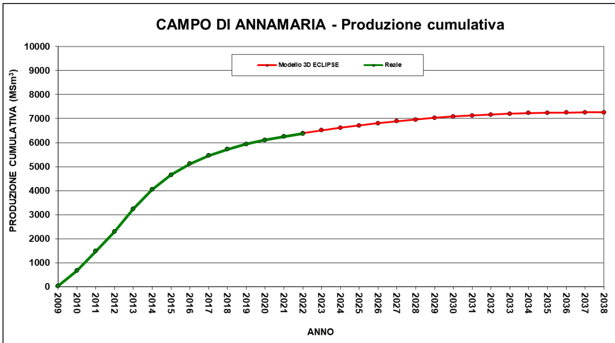
Figura 6 - Campo di Annamaria: grafico di produzione reale e da modello Eclipse 2021
