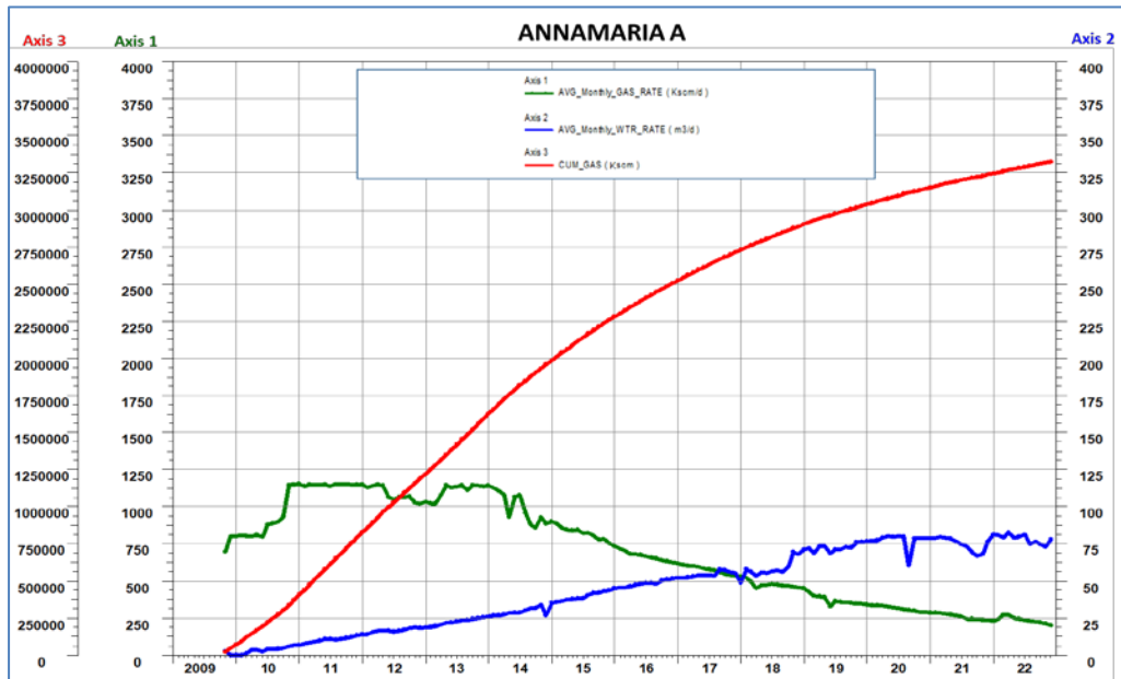
Figura 3 - Annamaria A (campo di Annamaria): produzione storica
