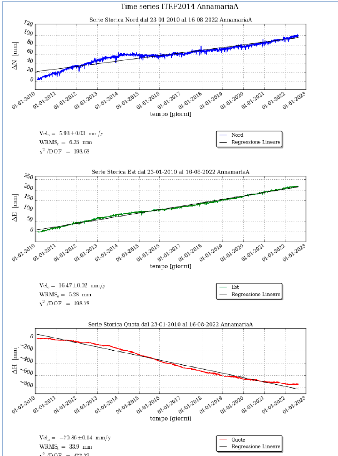
Figura 15 - Serie storiche di misure CGPS: piattaforma Annamaria A (acque croate)
