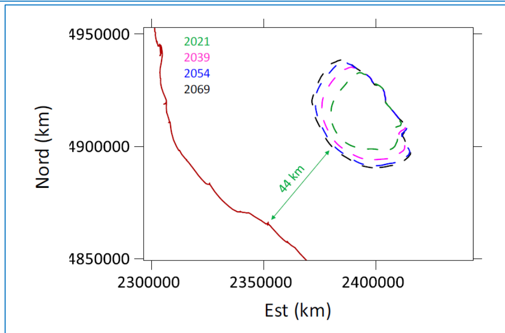
Figura 9 - Modello geomeccanico 2021. Caso DN . In alto: linee di iso-subsidenza dei 2 cm (linea tratteggiata) e 5 cm (linea continua) al termine della produzione (a sinistra) e a fine simulazione (a destra). Sotto: evoluzione temporale della linea di iso-subsidenza dei 2 cm. L'asterisco indica il punto di massimo.
