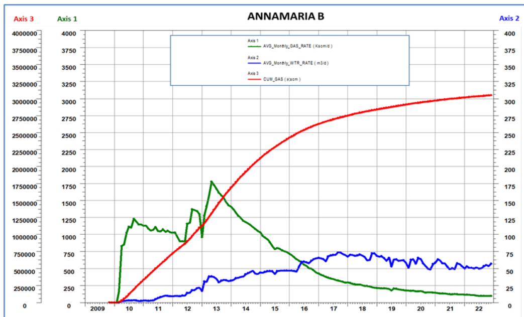
Figura 4 - Annamaria B (campo di Annamaria): produzione storica
