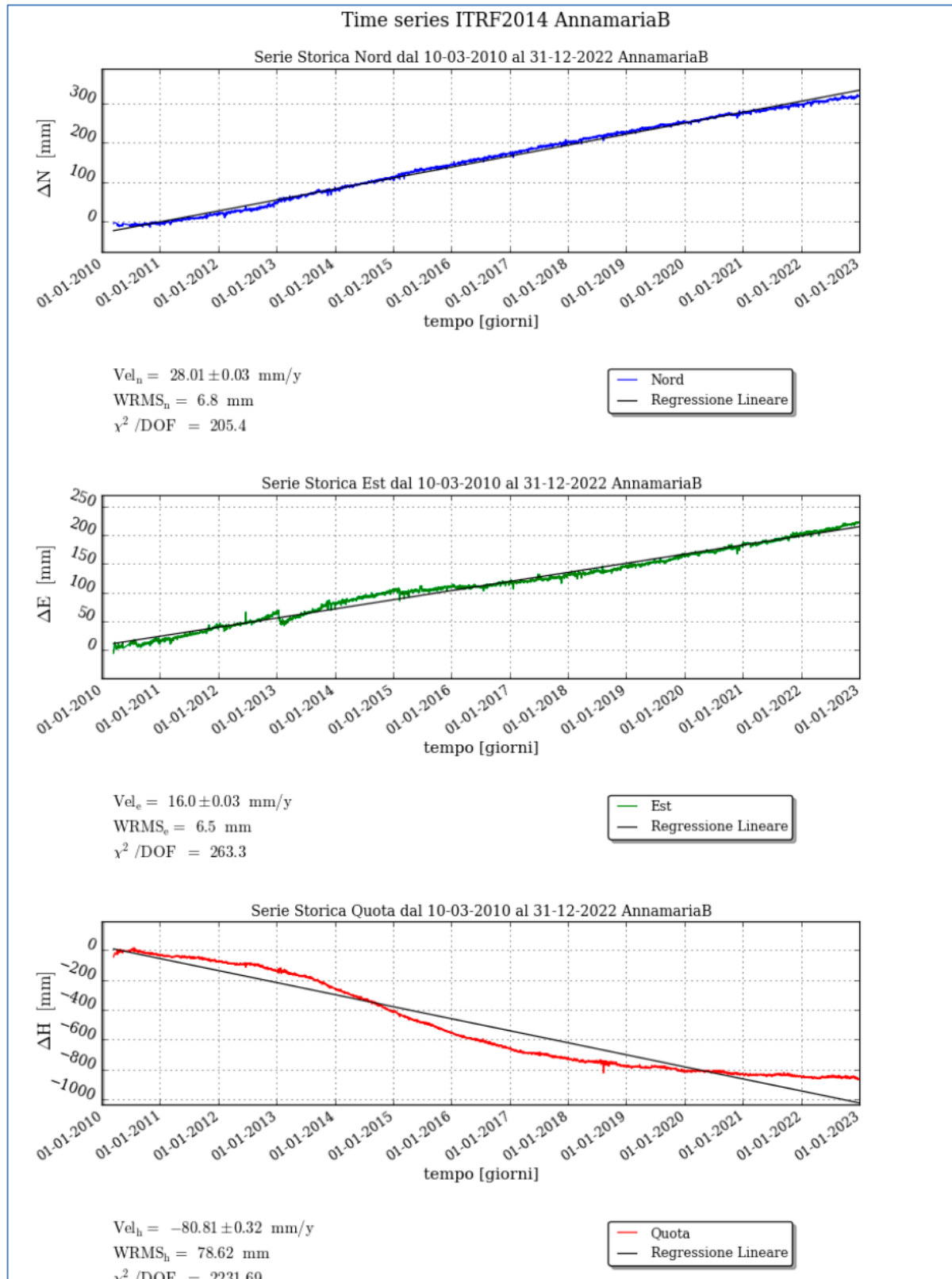
Figura 14 - Serie storiche di misure CGPS: piattaforma Annamaria B (acque italiane)
