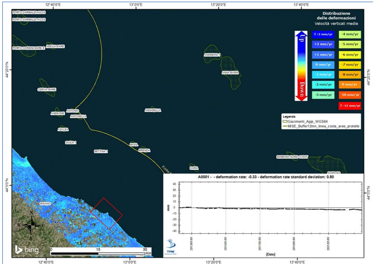
Figura 18 - Analisi dati InSAR dal 2012 al 2022 nel tratto di costa antistante il campo di Annamaria. Serie storica media (dal 2012 al 2022) dello spostamento medio ricavata dai dati InSAR all'interno del poligono rosso.
