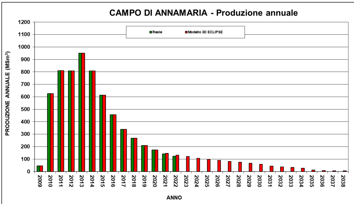
Figura 7 - Campo di Annamaria: produzione (annuale) reale e da modello Eclipse 2021
