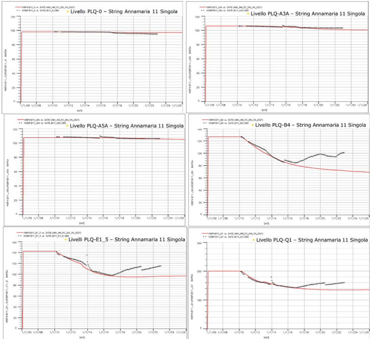
Figura 8 - Misure di pressione in continuo (Annamaria 11B PPG) e modello Eclipse 2021
