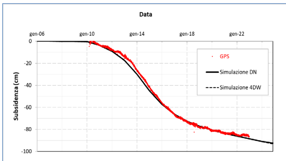
Figura 19 - Confronto fra la subsidenza totale misurata dalla stazione CGPS installata sulla piattaforma Annamaria B e i valori previsti dal modello geomeccanico del 2021
