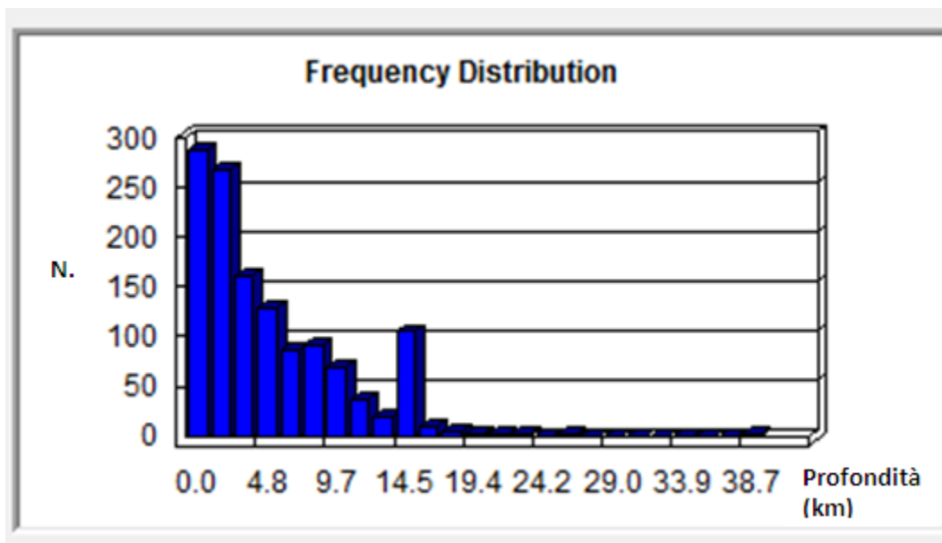
Fig. 14. Istogramma di frequenza delle profondità ipocentrali degli eventi registrati in un raggio di 20 km da Castel Giorgio nel periodo 1977-1991.
