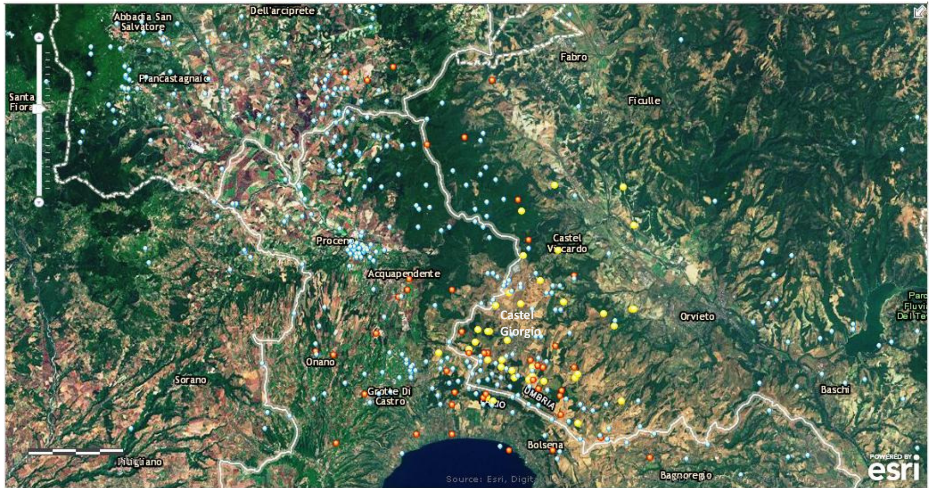
Fig. 11. Terremoti registrati dalla rete di monitoraggio INGV nel periodo compreso tra il 1984 e 2013. Arancione: eventi compresi tra il 1984 e 2004; Giallo: eventi avvenuti nel 1992. Azzurro: eventi dal 2005 al 2013 (Fonti INGV: Bollettino Sismico Italiano; ISIDE; Catalogo CSI 1.1 da Castello et al., 2006).
