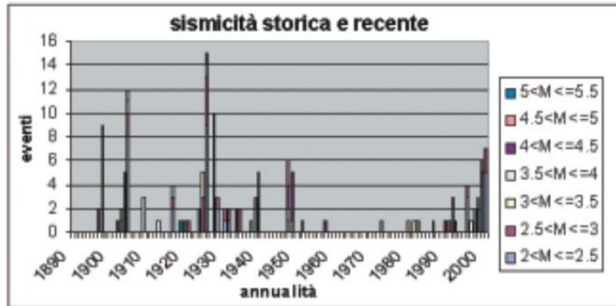
Grafico sismicità storica e recente.
