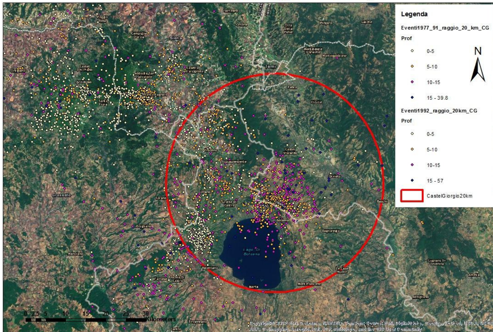
Fig. 13. Distribuzione degli epicentri dei terremoti registrati dalla rete Enel nel periodo 1977- 1992 distinti per profondità. Il cerchio rosso racchiude l'area con raggio = 20 km centrato su Castel Giorgio.
