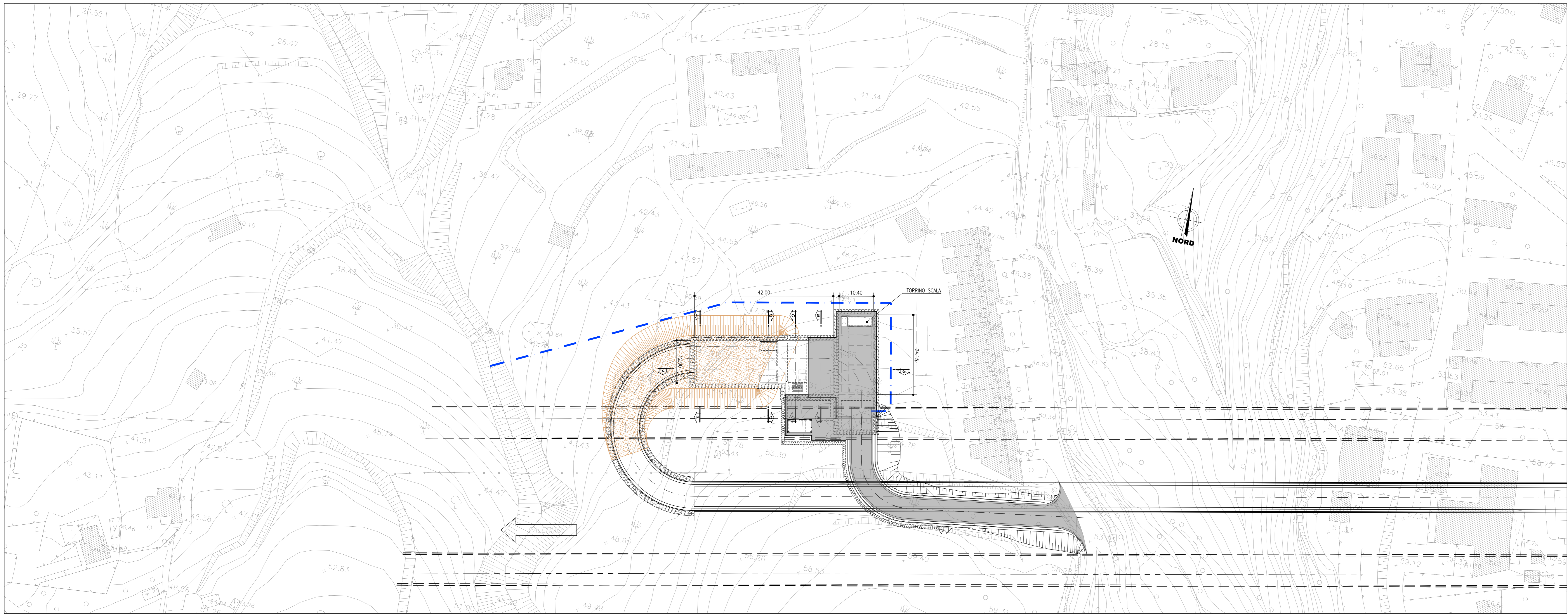
PLANIMETRIA SISTEMAZIONE DEFINITIVA - VISTA AEREA scala 1:500
