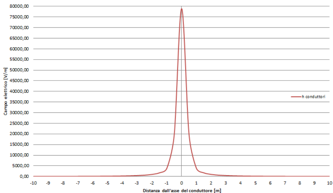
Andamento del campo elettrico e magnetico in funzione della distanza dall'asse dei conduttori in forma grafica - Sbarre MT della cabina di raccolta.
