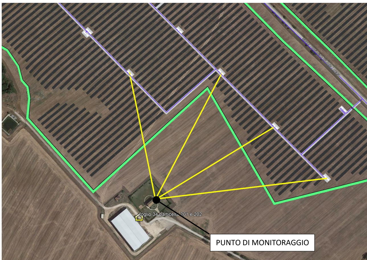
Individuazione del ricettore significativo n.7 e n.8 e distanza dalle cabine inverter e trasformazione
