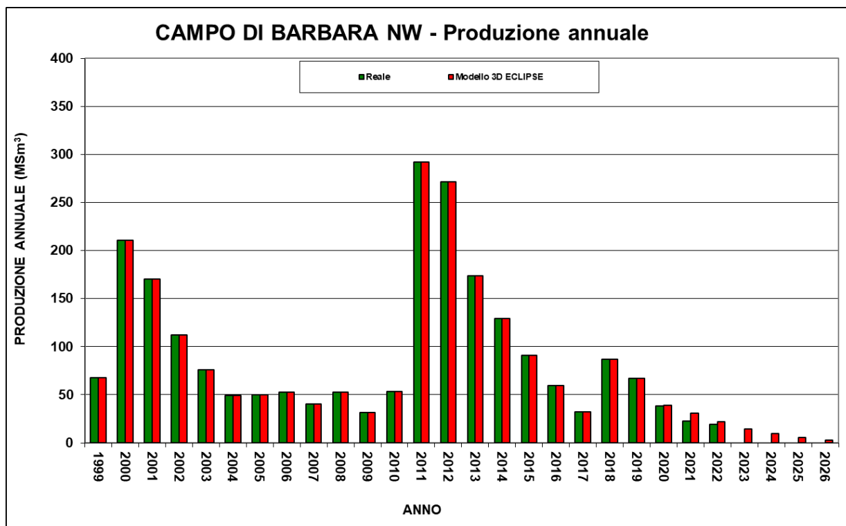
Figura 6 - Campo di Barbara NW: produzioni (annuale) reale e da modello Eclipse 2021
