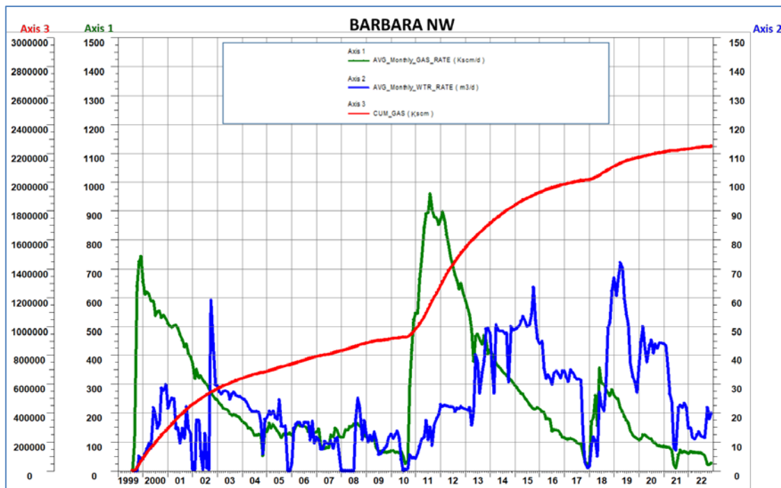
Figura 3 - Campo di Barbara NW: grafico della produzione storica
