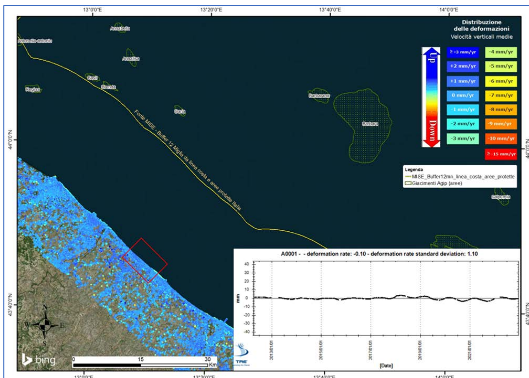
Figura 14 - Analisi dati InSAR dal 2012 al 2022 nel tratto di costa antistante il campo di Barbara-NW. Serie storica media (dal 2012 al 2022) dello spostamento medio ricavata dai dati InSAR all'interno del poligono rosso.
