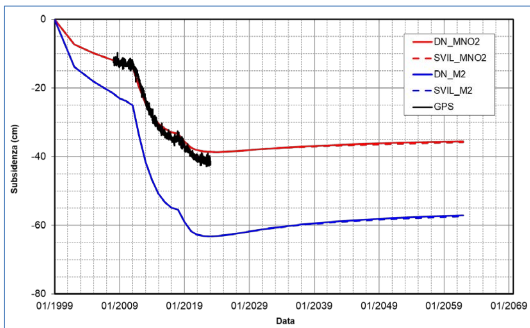
Figura 15 - Campo di Barbara NW: misure CGPS vs. previsioni di subsidenza da modello geomeccanico (in corrispondenza della piattaforma)
