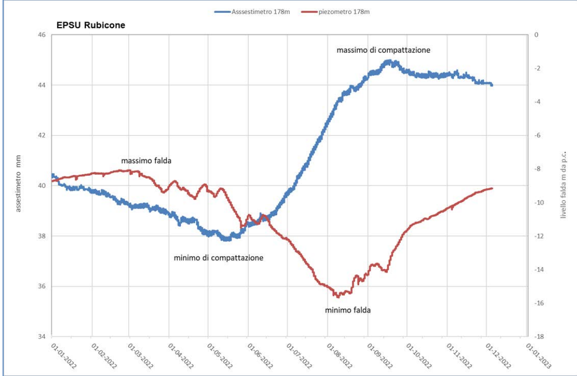
Figura 8B - Stazione EPSU di Rubicone: misure piezometrico-assestimetriche, ultimo anno di dati
