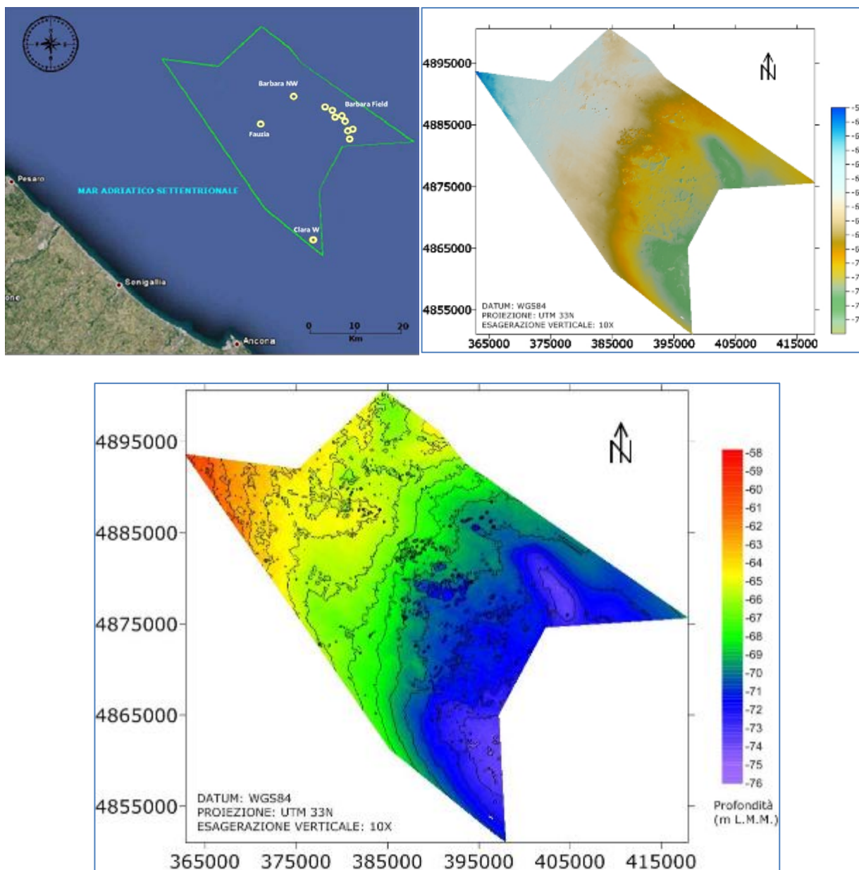
Figura 10 - Campo di Barbara NW: rilievo batimetrico. In alto e a lato: ubicazione-estensione dell'area rilevata e superficie 3D dell'area indagata; in basso: la mappa delle isobate.
