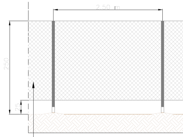
Figura 7 - Rappresentazione della recinzione prevista di altezza pari a 2.5m
