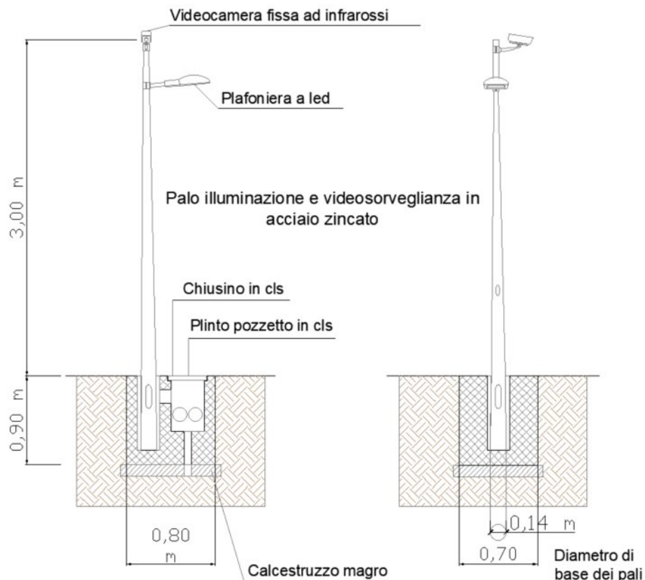
Figura 8 - Rappresentazione pali per illuminazione e videosorveglianza
