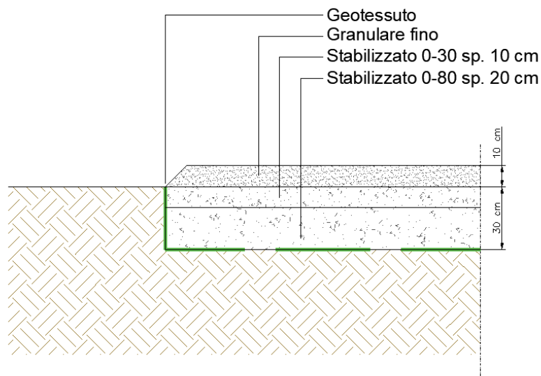
Figura 6 - Sezione tipo viabilità interna all'impianto e piazzali
