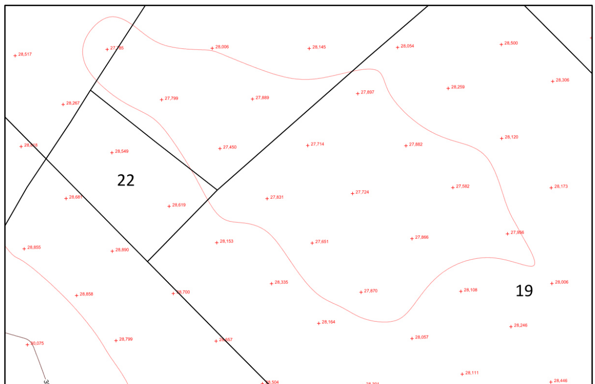
Immagine 1 -piano quotato impianto 3
