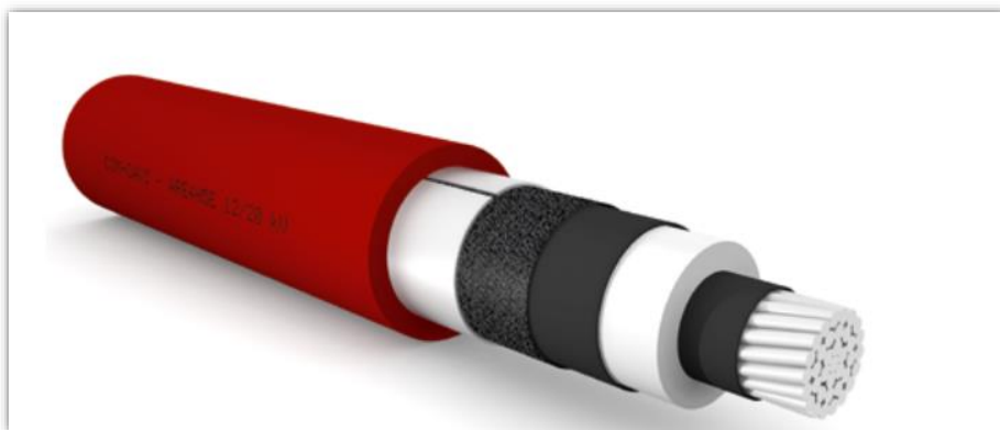
Fig. 6. Particolare degli strati costitutivi di un cavo ARE4H5EE
