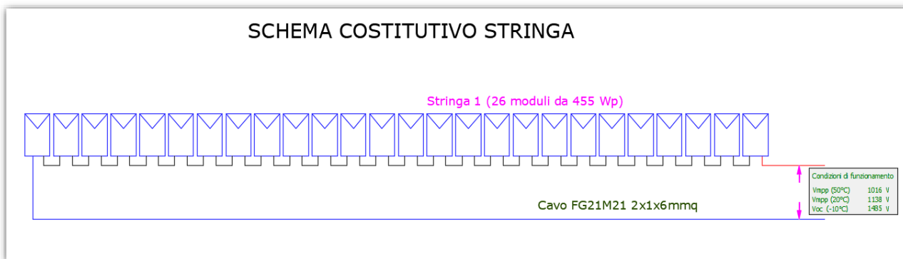
Fig. 2. Esempio di particolare serie moduli fotovoltaici
