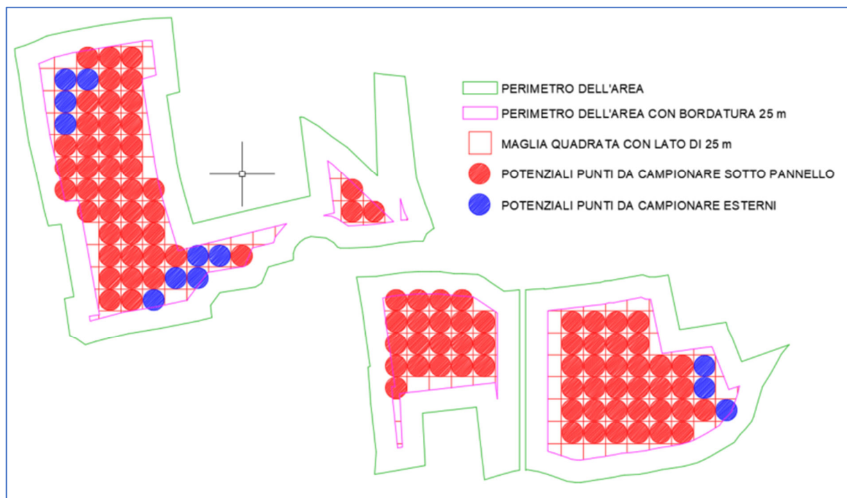
Fig. 10_ Area Impianto con bordura di 25 m, griglia a maglia quadra da 25 m di lato e potenziali punti di campionamento
