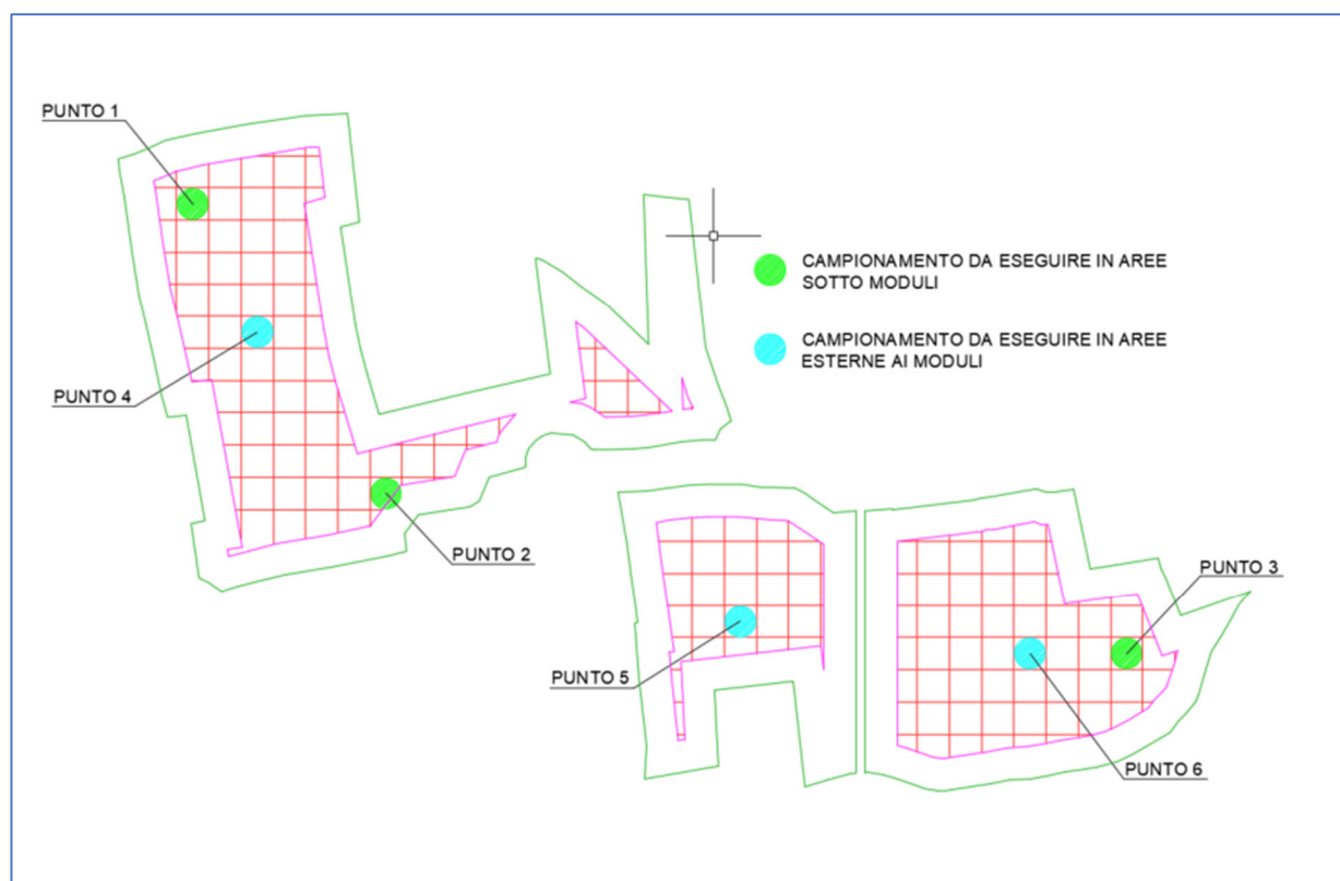
Fig.11 _ Area Impianto con indicazione dei punti da campionare
