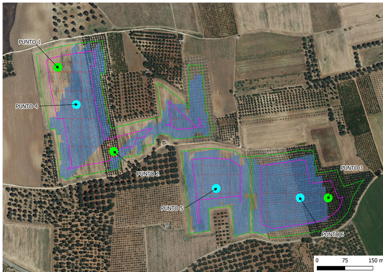
Fig. 12 _ Carta dei siti di campionamento del suolo e sottosuolo durante la fase d'esercizio dell'impianto
