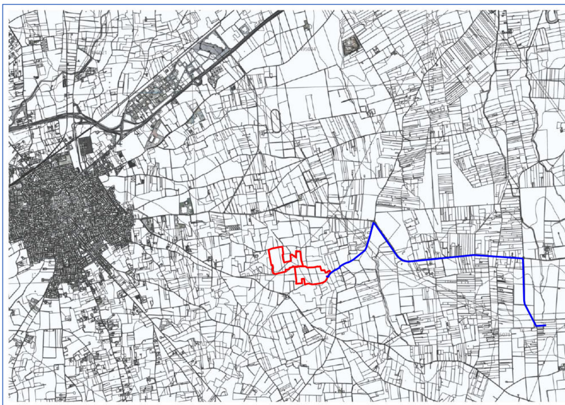
Fig. 03 _ Stralcio della CTR con ingombro dell'impianto ed elettrodotto di connessione alla rete
