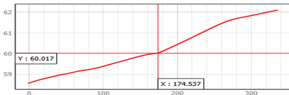
PROFILO C-C'
