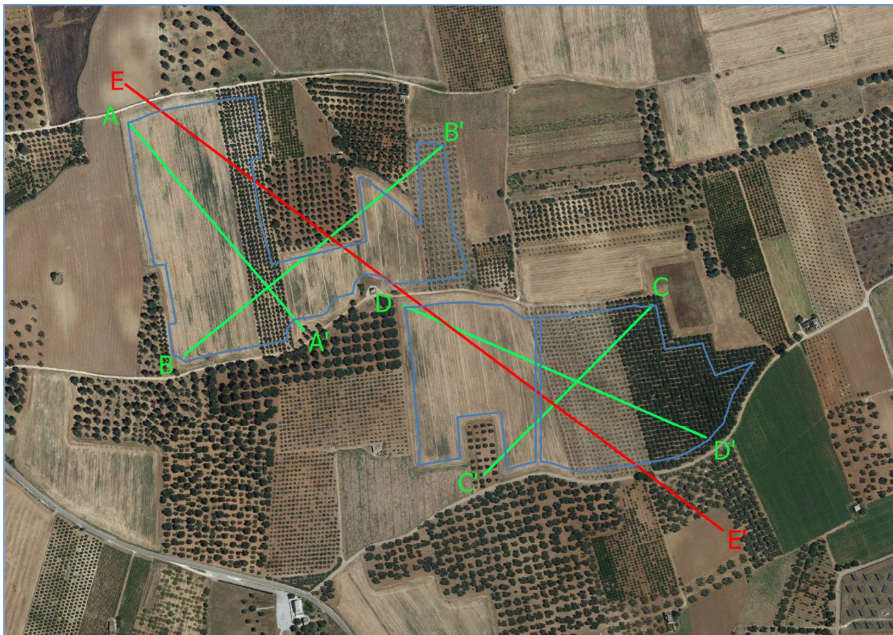
Fig. 03 _Area impianto e sezioni profilo morfologico.
