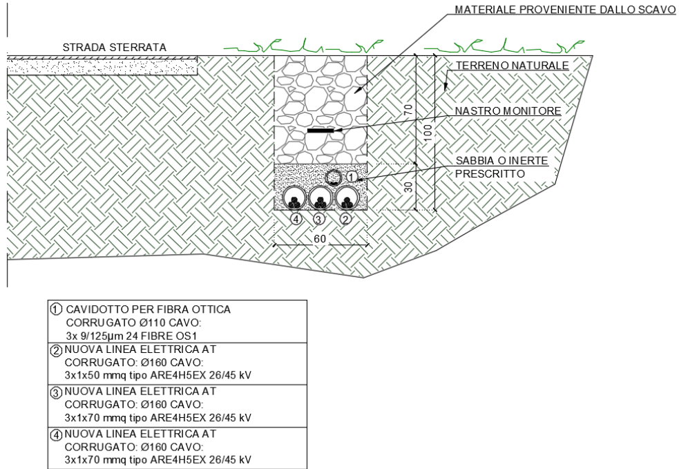
Figura 11 - Sezione tipologico D
