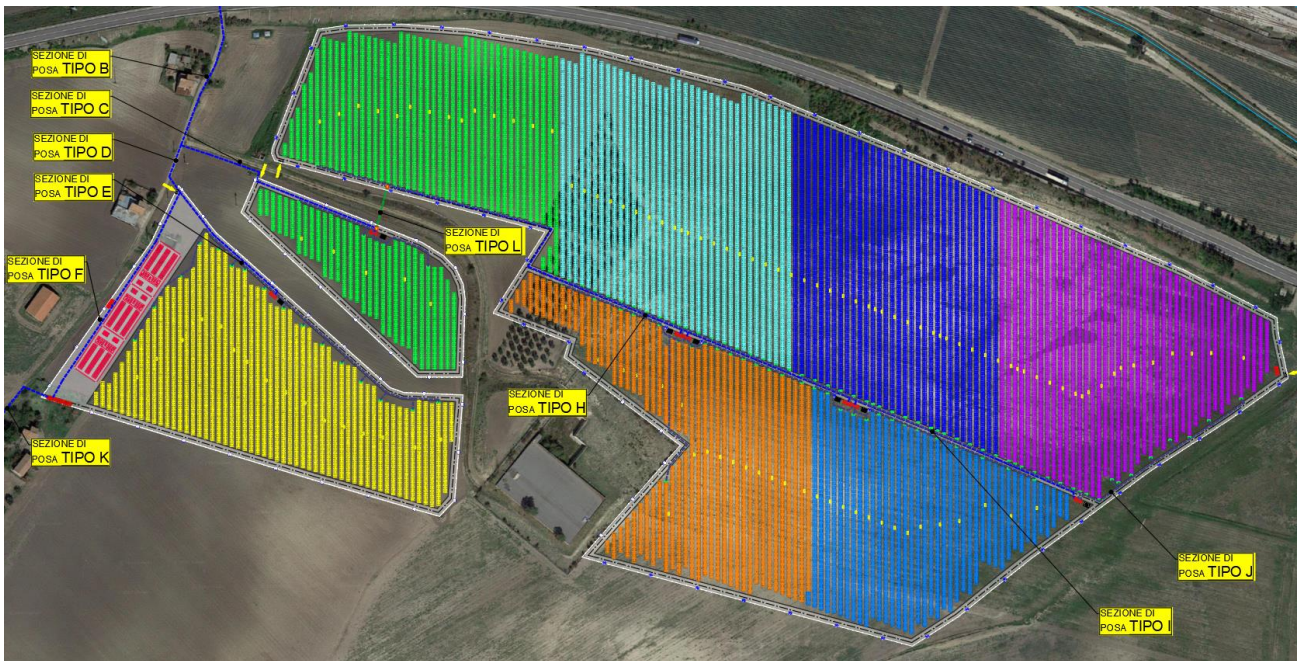
Figura 5 Planimetria stralcio 1 su ortofoto
