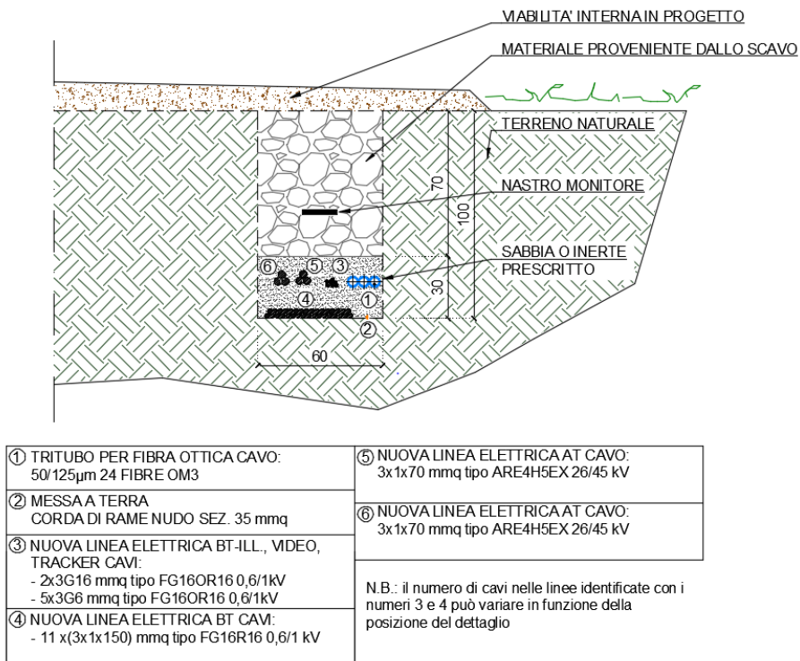
Figura 15 - Sezione tipologico H
