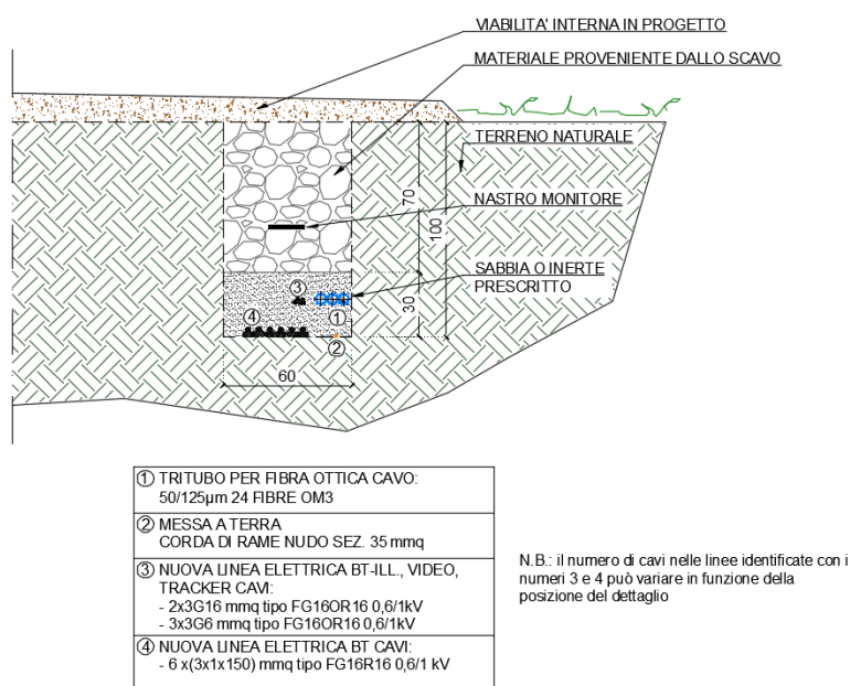
Figura 8 - Sezione tipologico A
