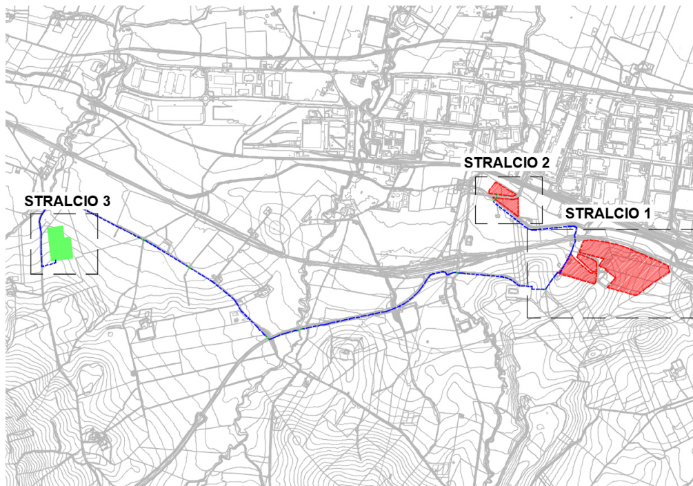
Figura 4 Kmap con sviluppo del cavidotto di connessione
