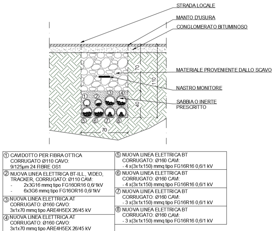
Figura 14 - Sezione tipologico G
