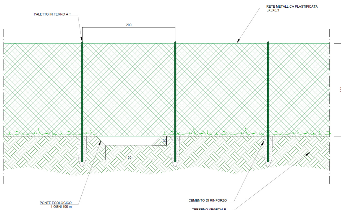
Figura 2 - Prospetto recinzione tipologico 1
