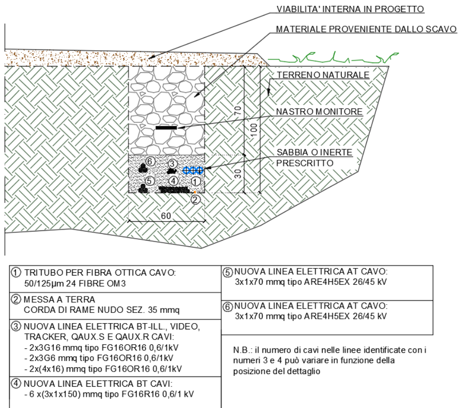
Figura 12 - Sezione tipologico E
