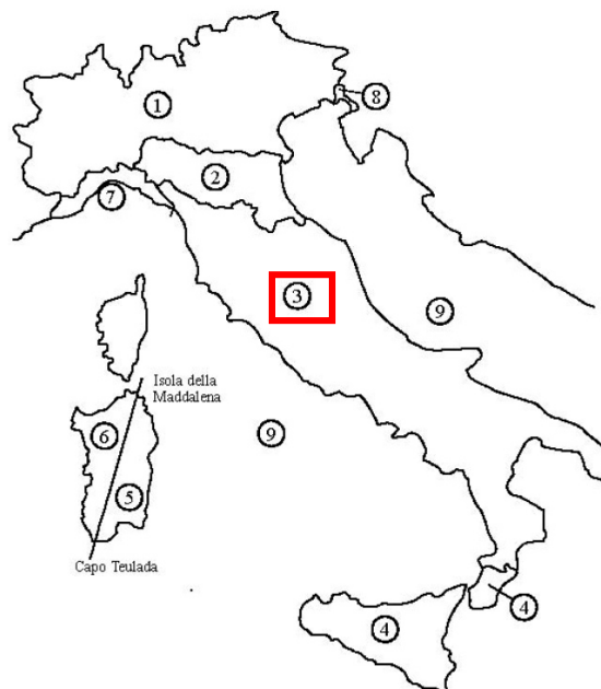
Figura 22 – Mappa delle zone in cui è diviso il territorio italiano
