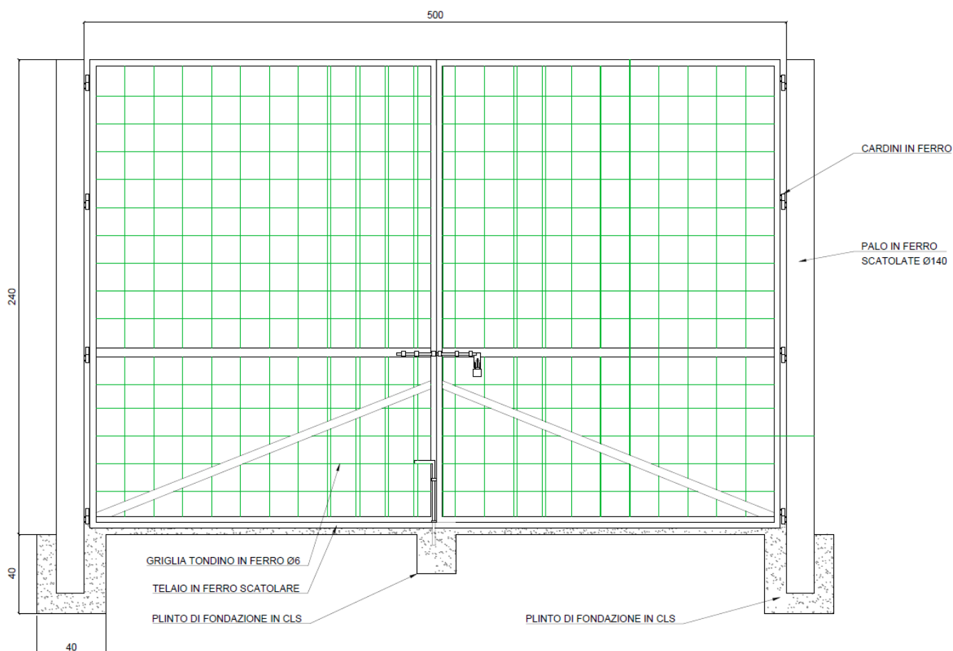
Figura 3 - Particolare cancello d'ingresso
