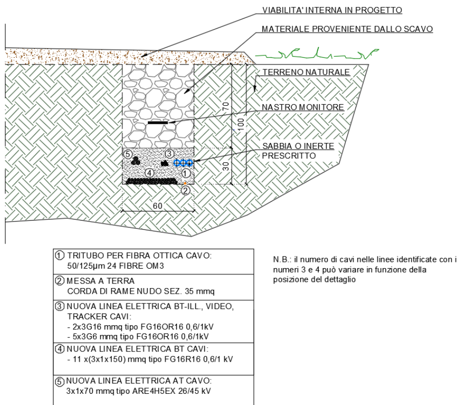
Figura 16 - Sezione tipologico I
