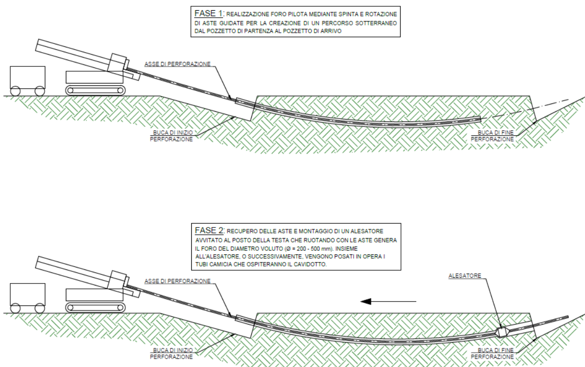
Figura 19 - Metodologia di posa tramite trivellazione TOC
