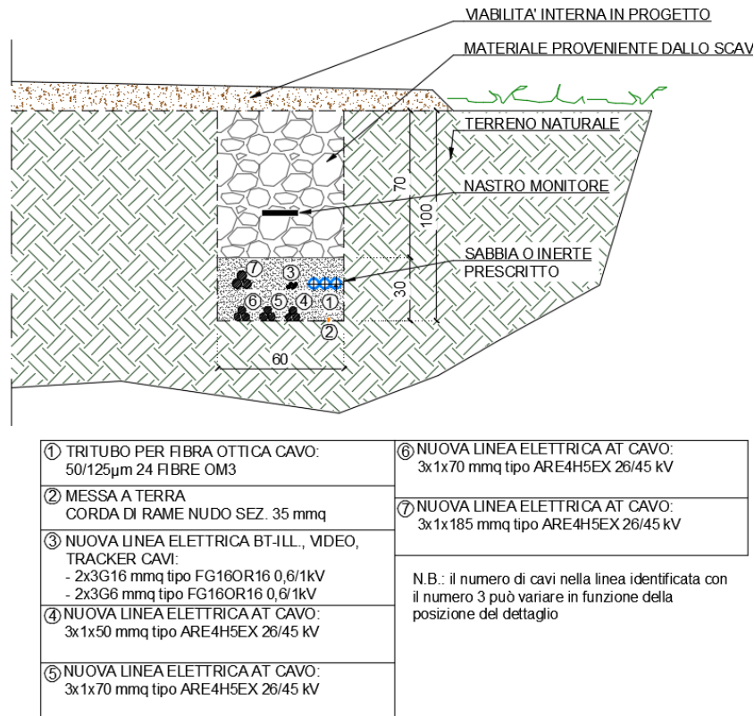
Figura 13 - Sezione tipologico F
