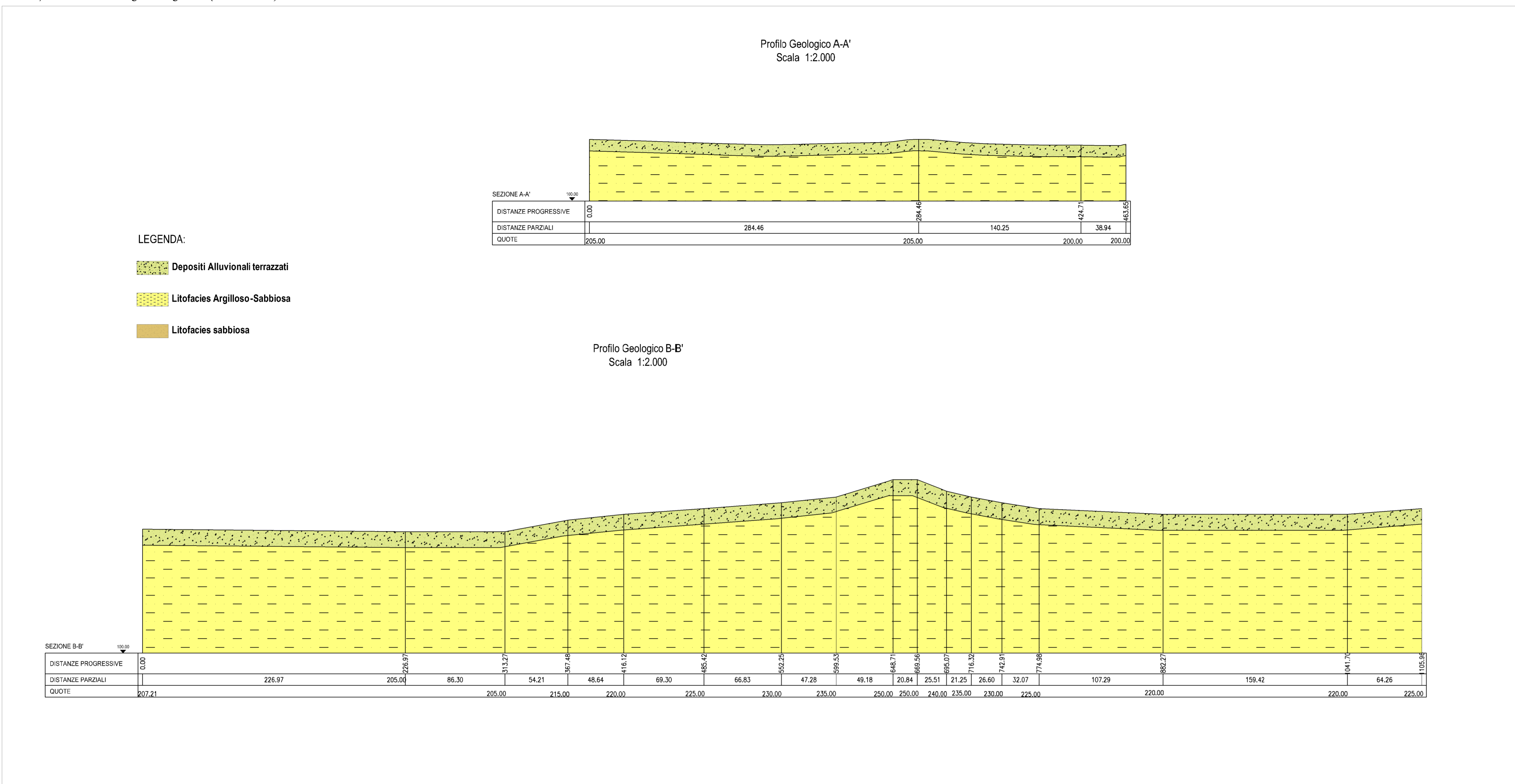
Tav.1/b: Profilo geologico (1:2.000)
