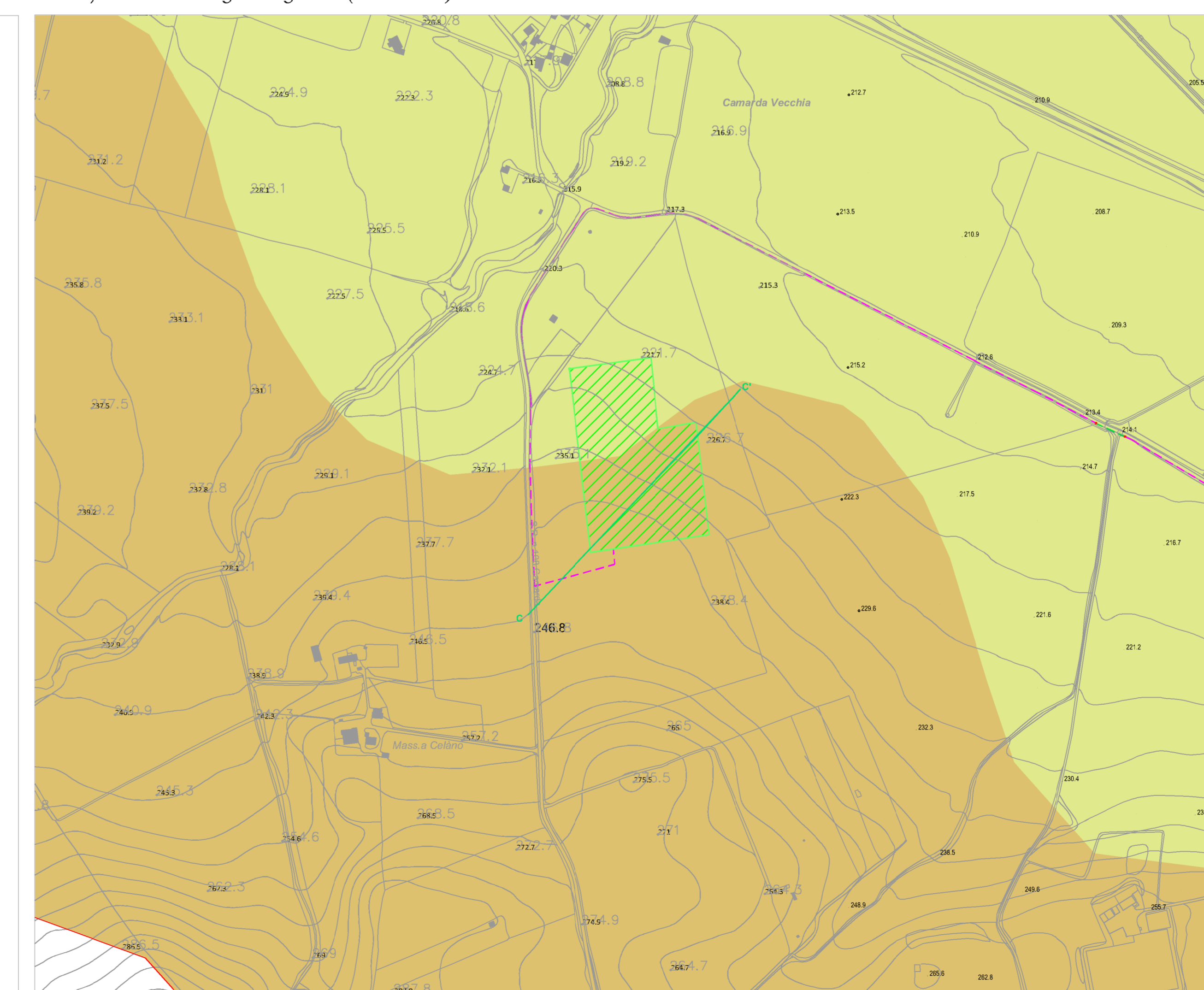
Tav.2/b: Carta geologica (1:5.000)
