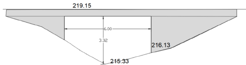
Figura 38 - Particolare dell'intersezione 1
