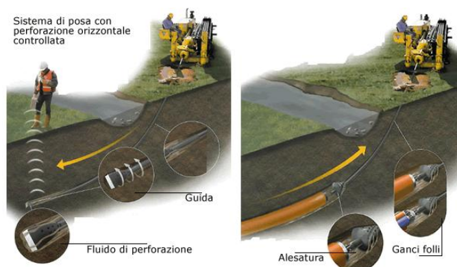
Figura 12: Posa in opera tubazione per alloggiare cavi
