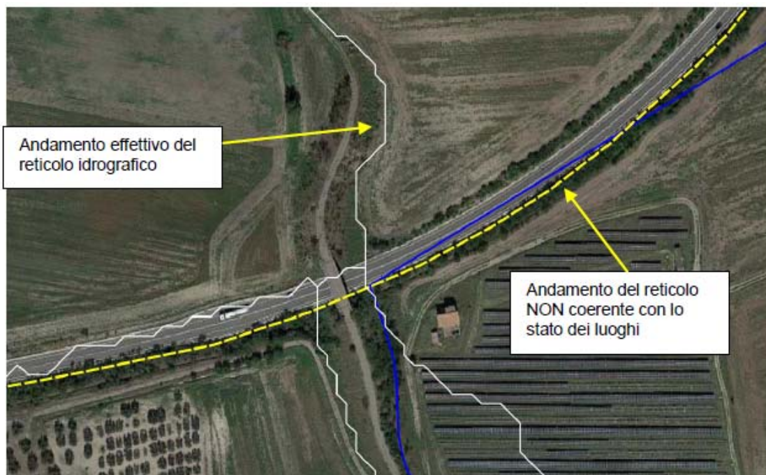
Figura 39 - Particolare dell'intersezione 2
