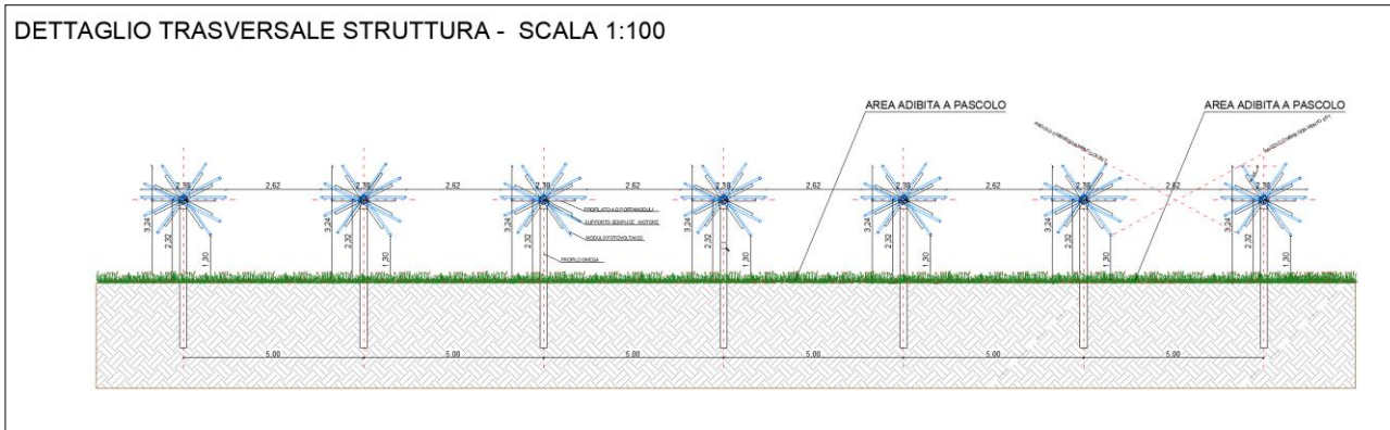
Figura 4. Dettaglio trasversale
