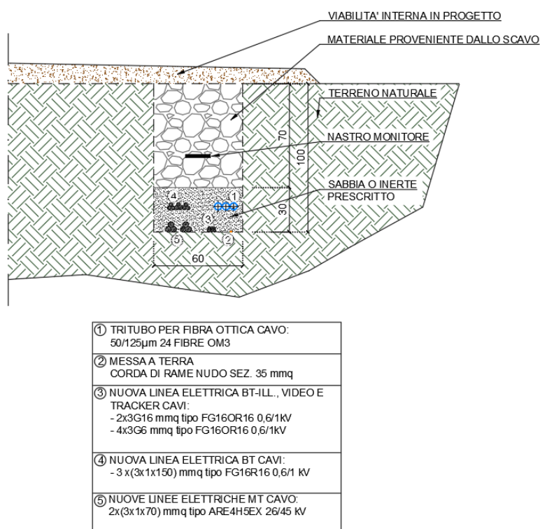
Figura 2 - Sezione tipologica di posa dei cavidotti
