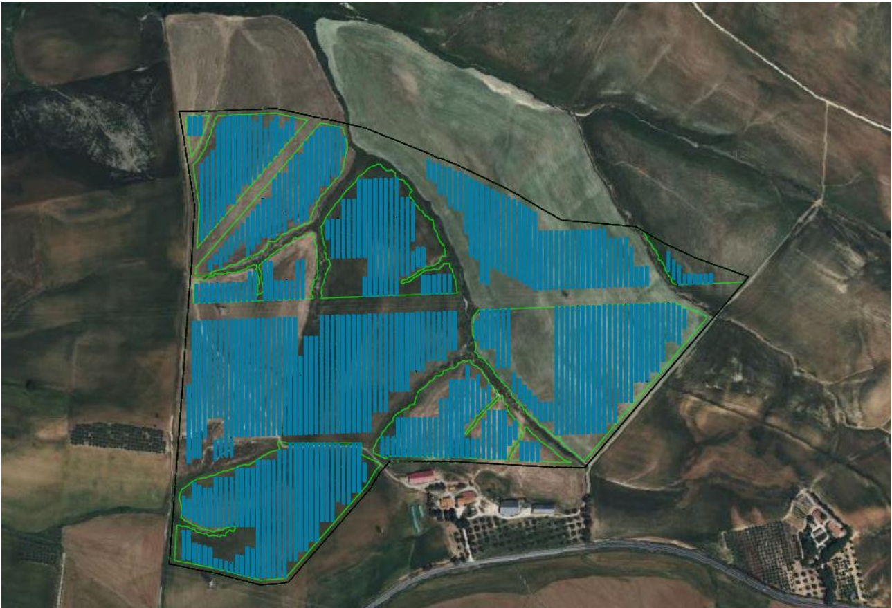
Figura 2 - VISTA DALL'ALTO DEL TERRENO: STATO DI PROGETTO
