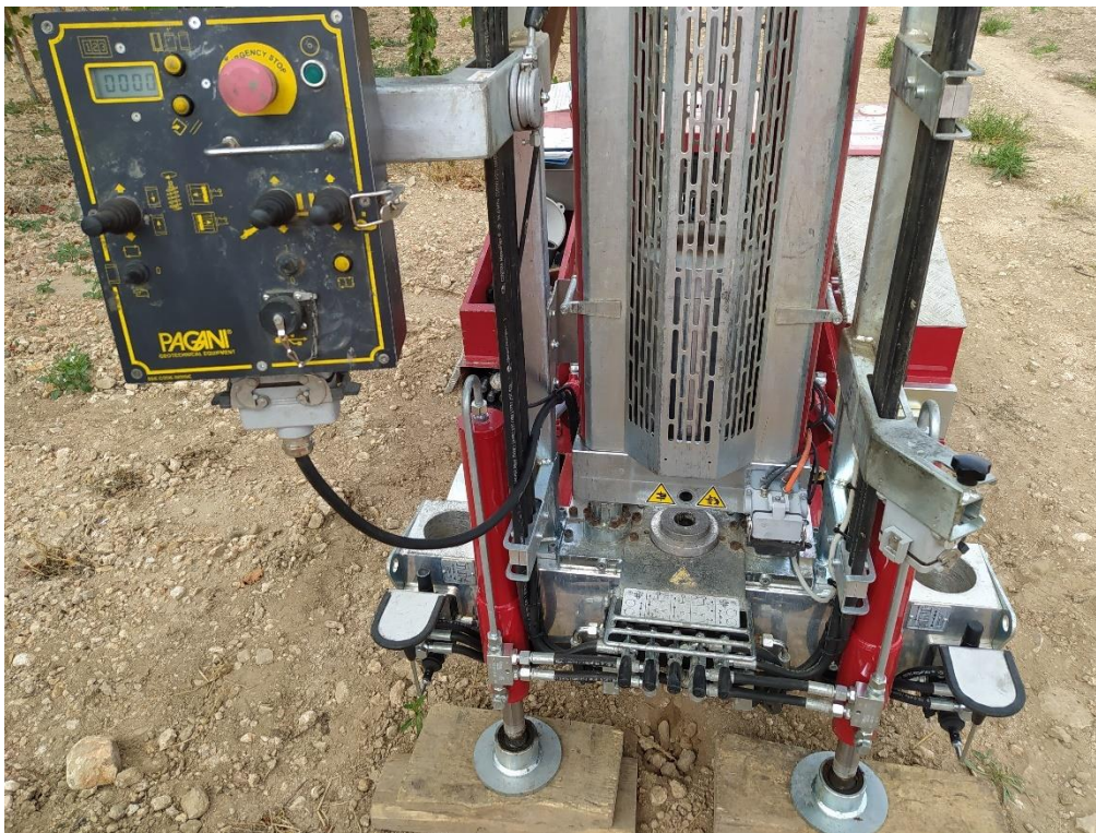
Postazione della DPSH 7
